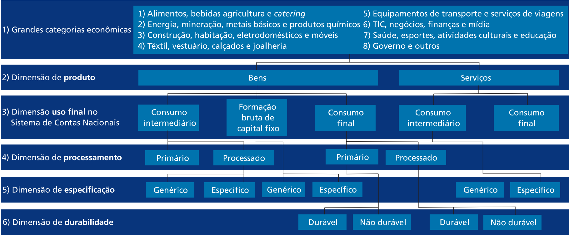
FIGURA 1 Relacionamentos na BEC revisão 5
