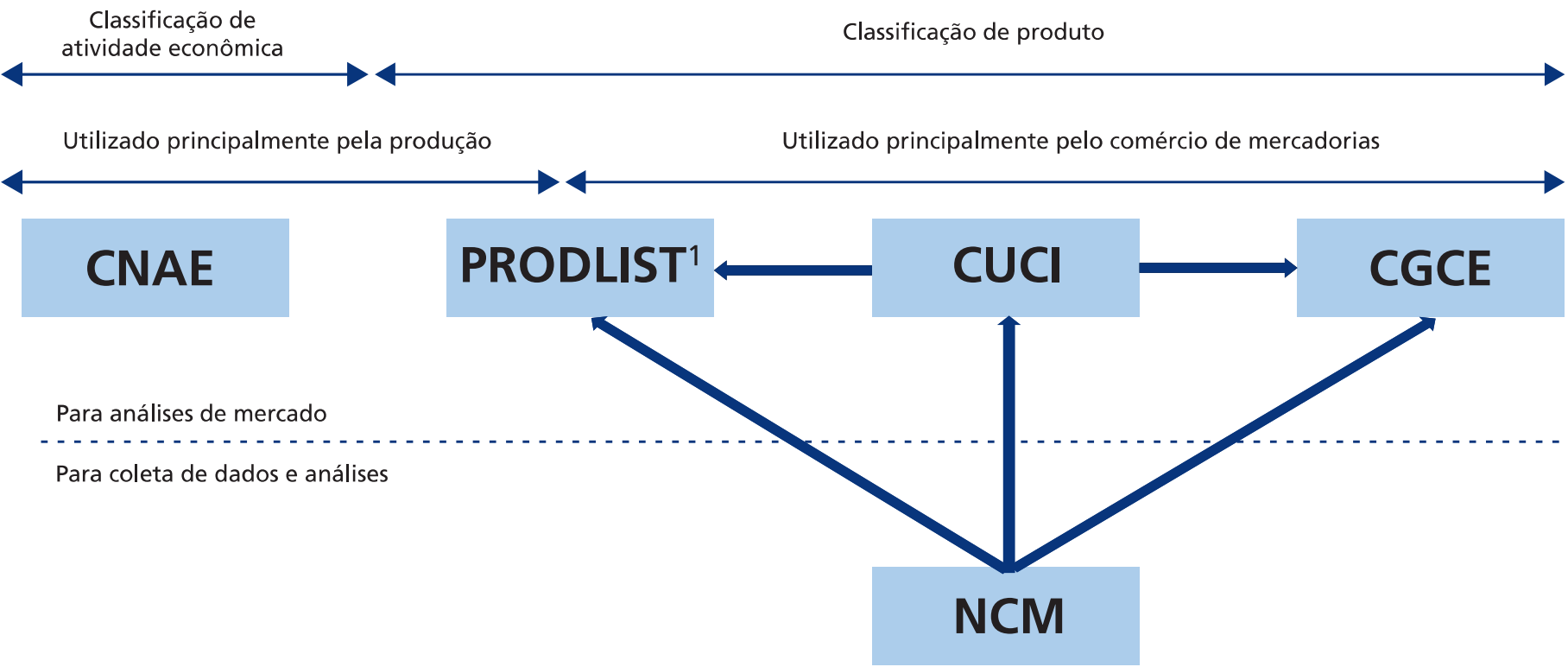
FIGURA 3 Relacionamento entre as diferentes classificações nacionais selecionadas
