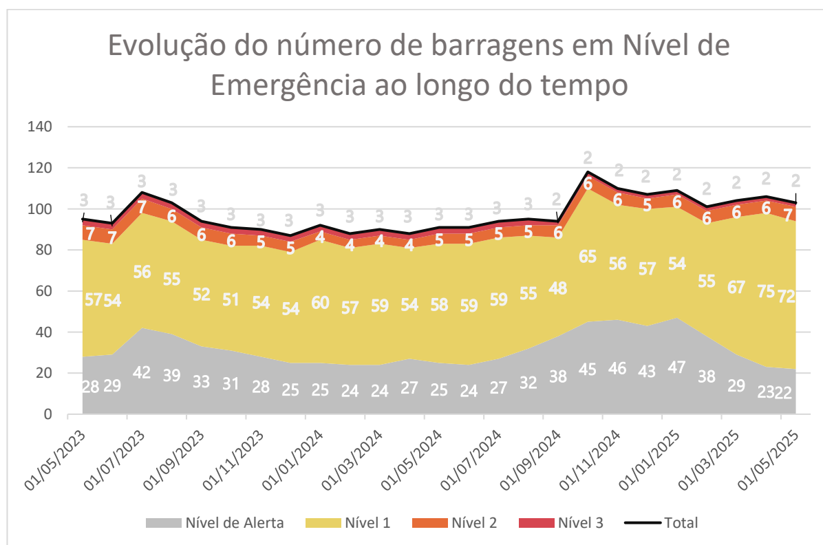
Figura 6 - Quantitativo do número de barragens em nível de alerta ou emergência ao longo dos anos.
