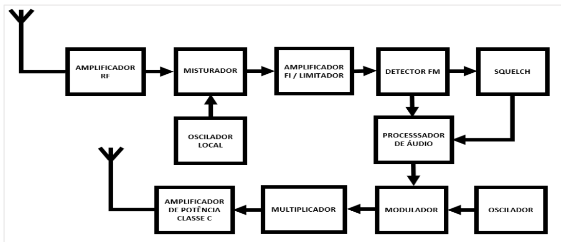
Diagrama de blocos de uma Repetidora de Radioamador
