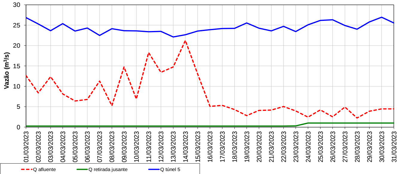
Vazões características do reservatório Atibainha
