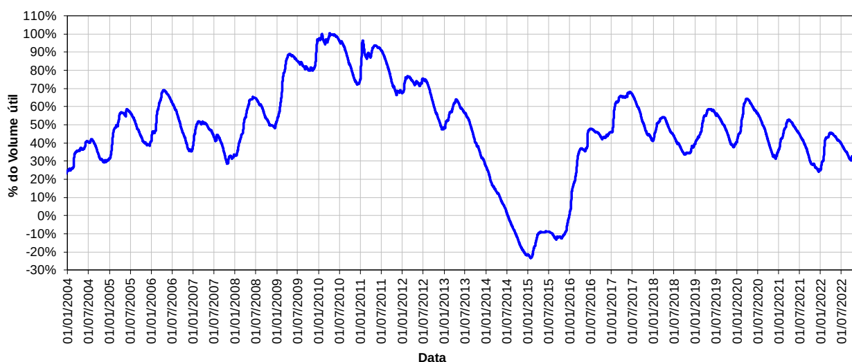
Evolução do volume útil do Sistema Cantareira - a partir de 2004
