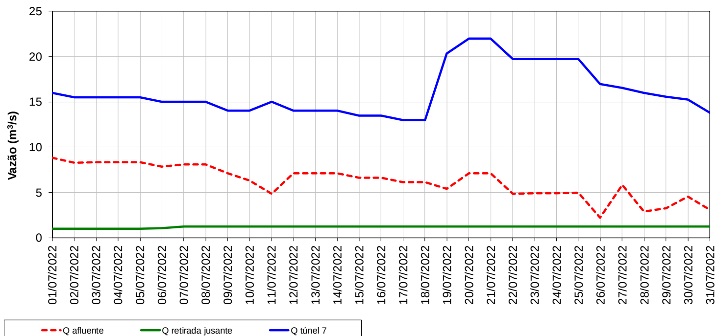
Vazões características do reservatório Jaguari-Jacareí
