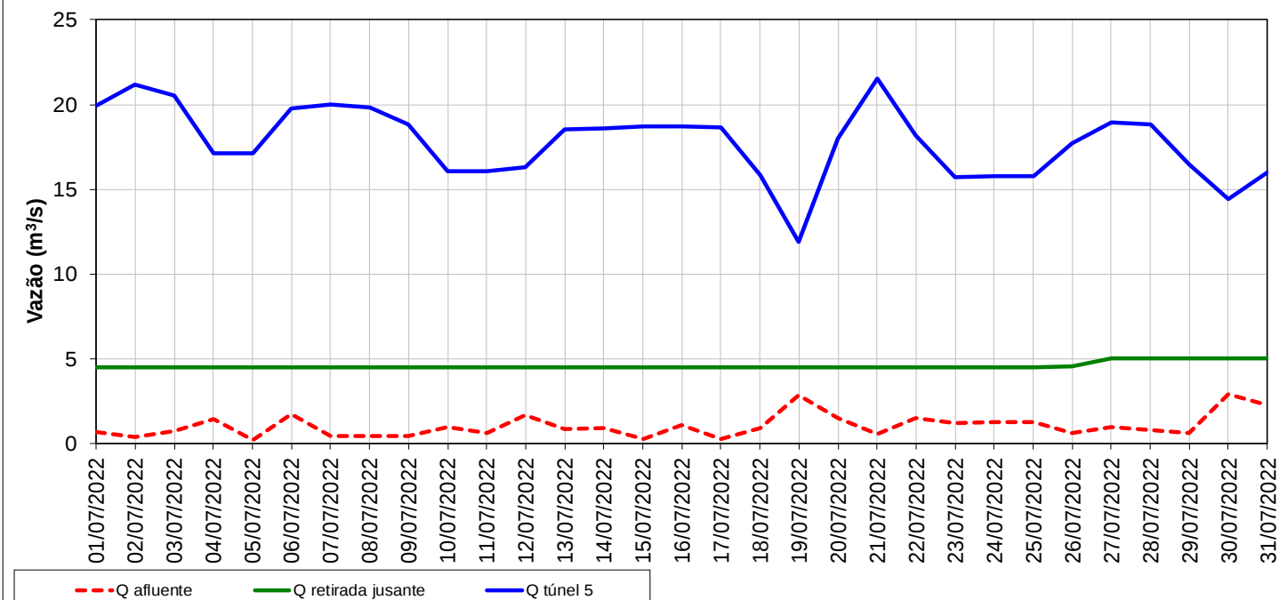
Vazões características do reservatório Atibainha
