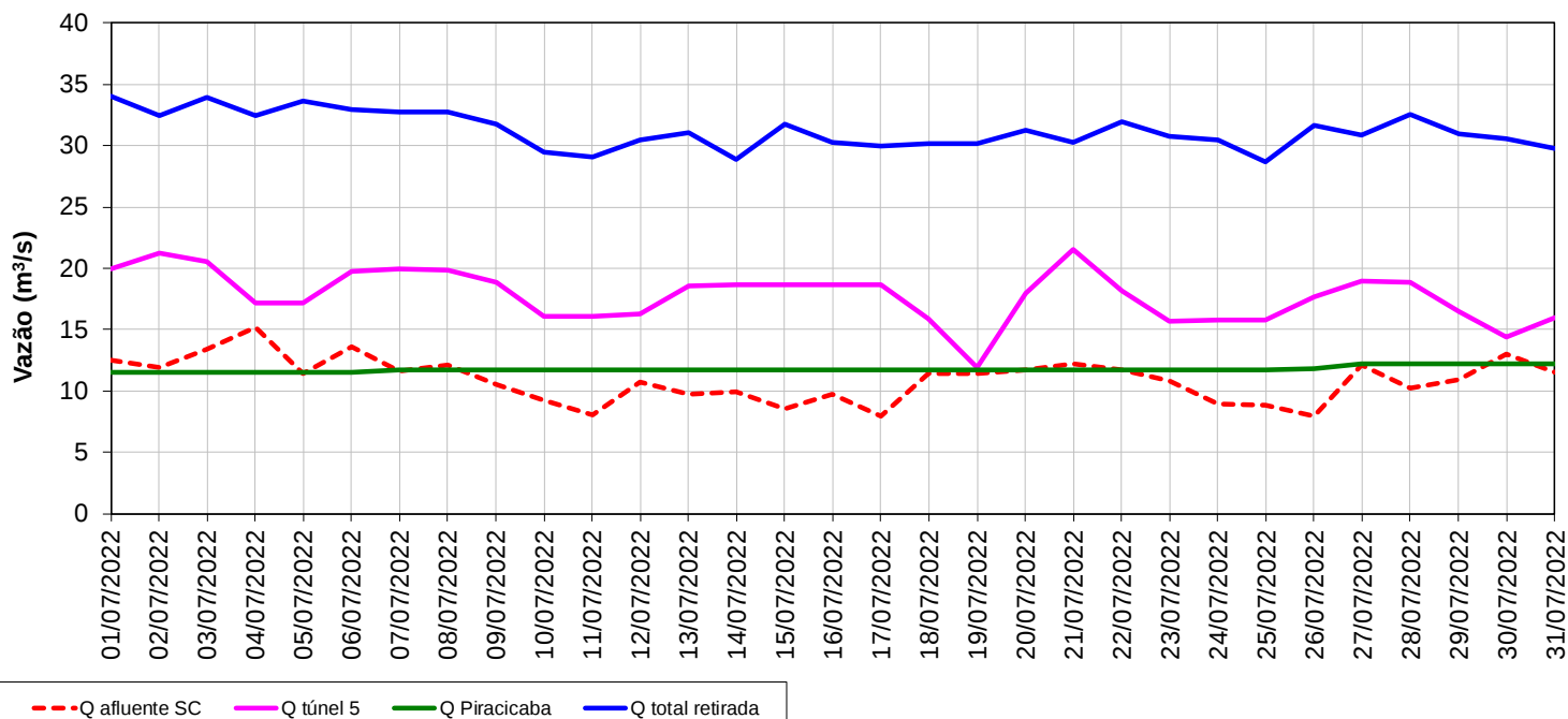
Vazões características do Sistema Cantareira
