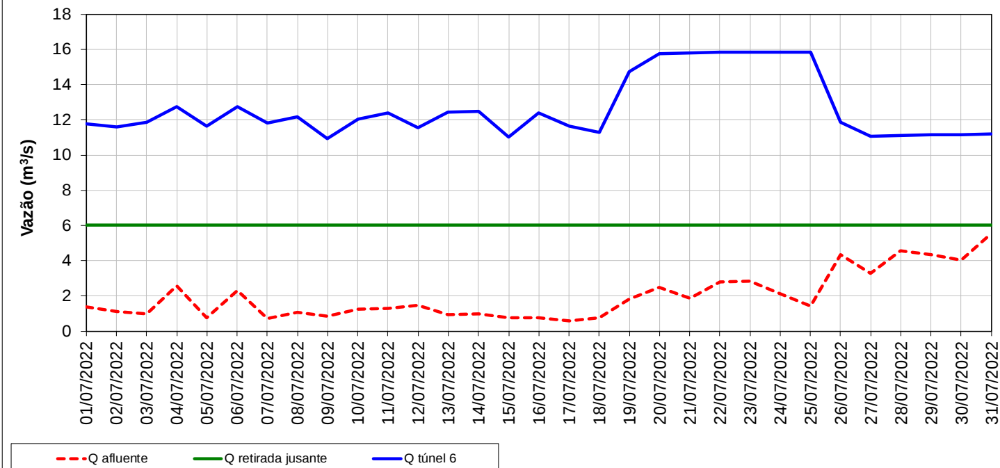
Vazões características do reservatório Cachoeira
