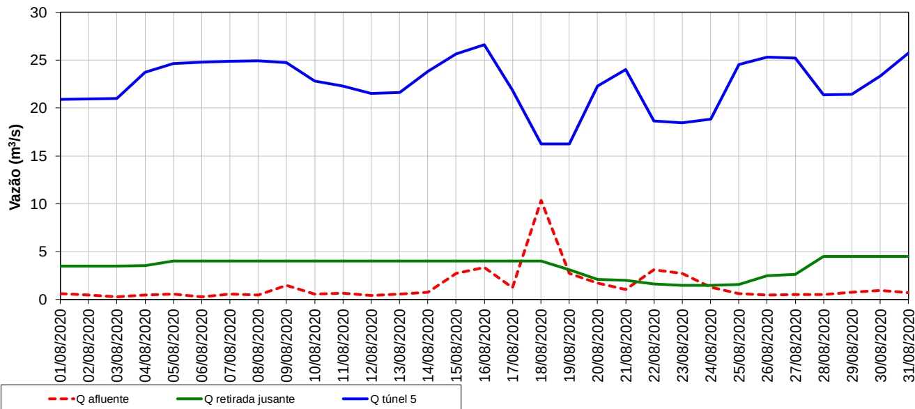
Vazões características do reservatório Atibainha
