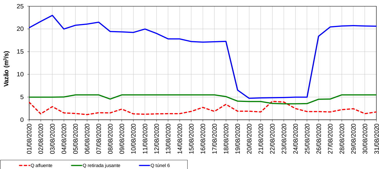
Vazões características do reservatório Cachoeira
