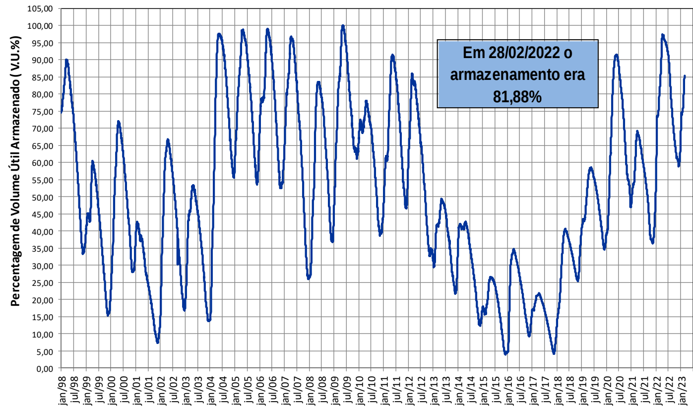
RESERVATÓRIO EQUIVALENTE - VOLUME ACUMULADO DESDE 1998
