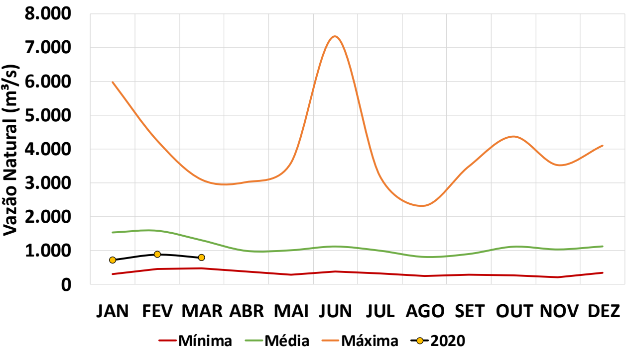
Vazões Naturais Médias Mensais em 2020
