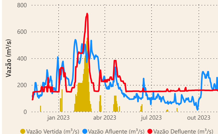
UHE Jurumirim
