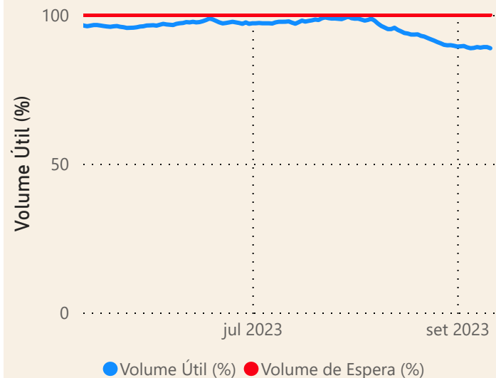
UHE Capivara
