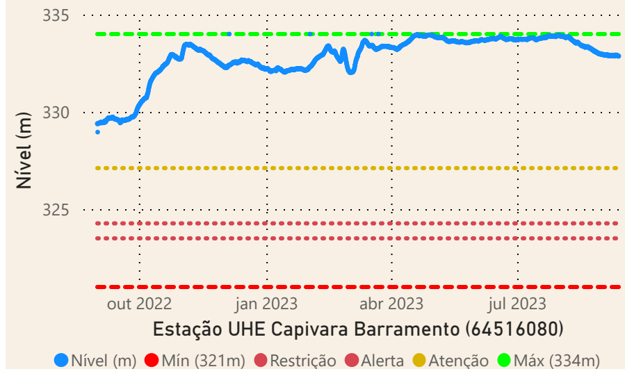
UHE Capivara
