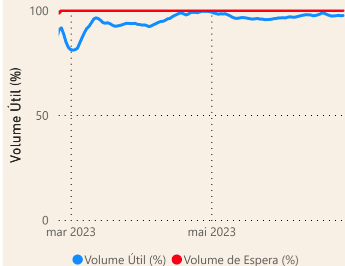
UHE Capivara
