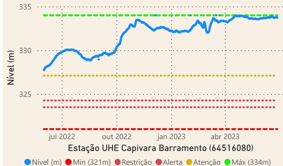
UHE Capivara
