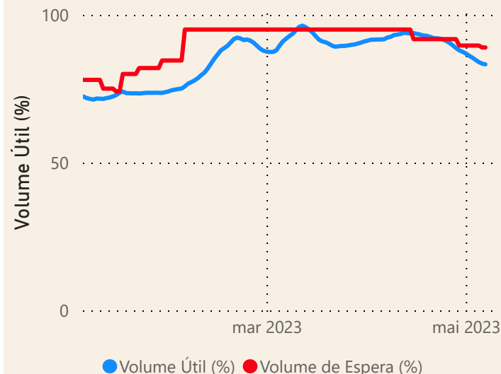
UHE Chavantes
