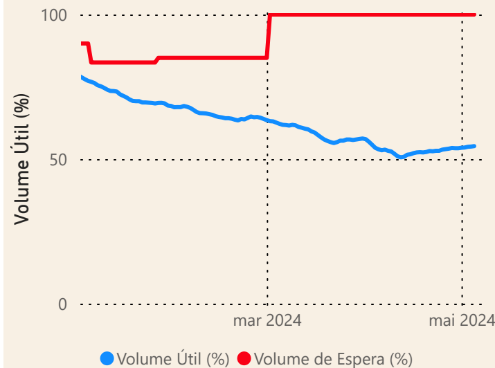
UHE Capivara
