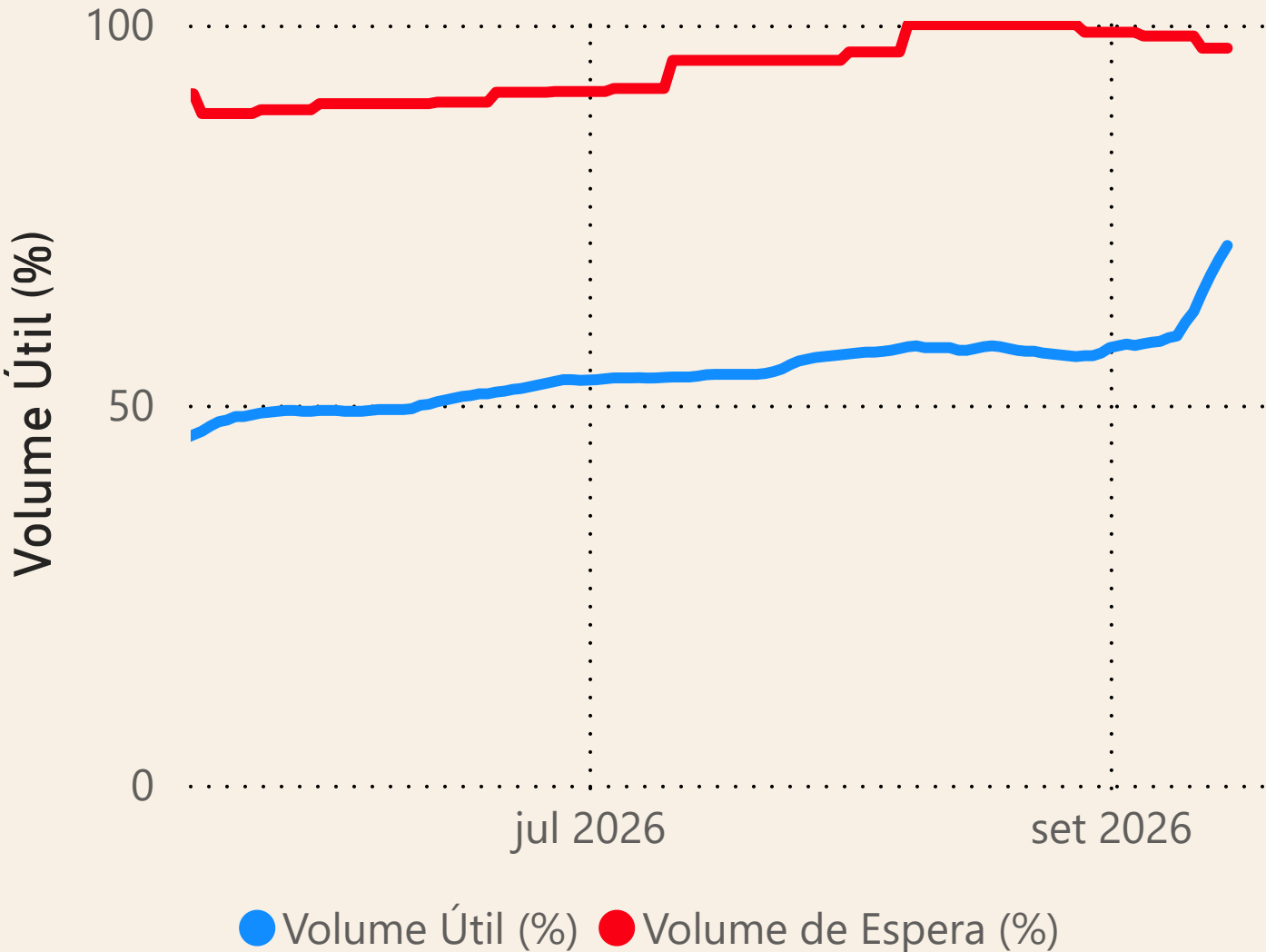
UHE Chavantes
