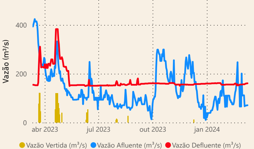
UHE Jurumirim
