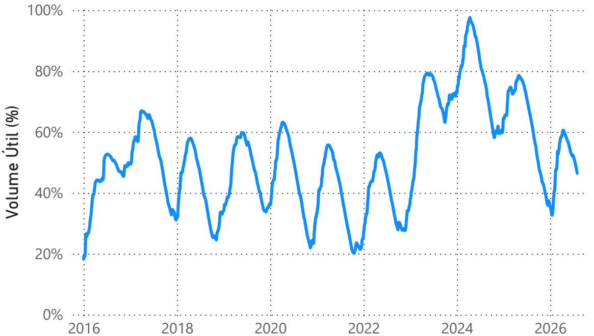
Reservatório Equivalente no fim de julho
