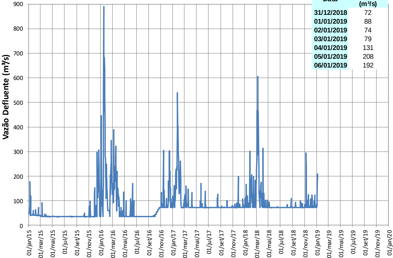
SANTA CECÍLIA - VAZÃO DEFLUENTE (m³/s)
