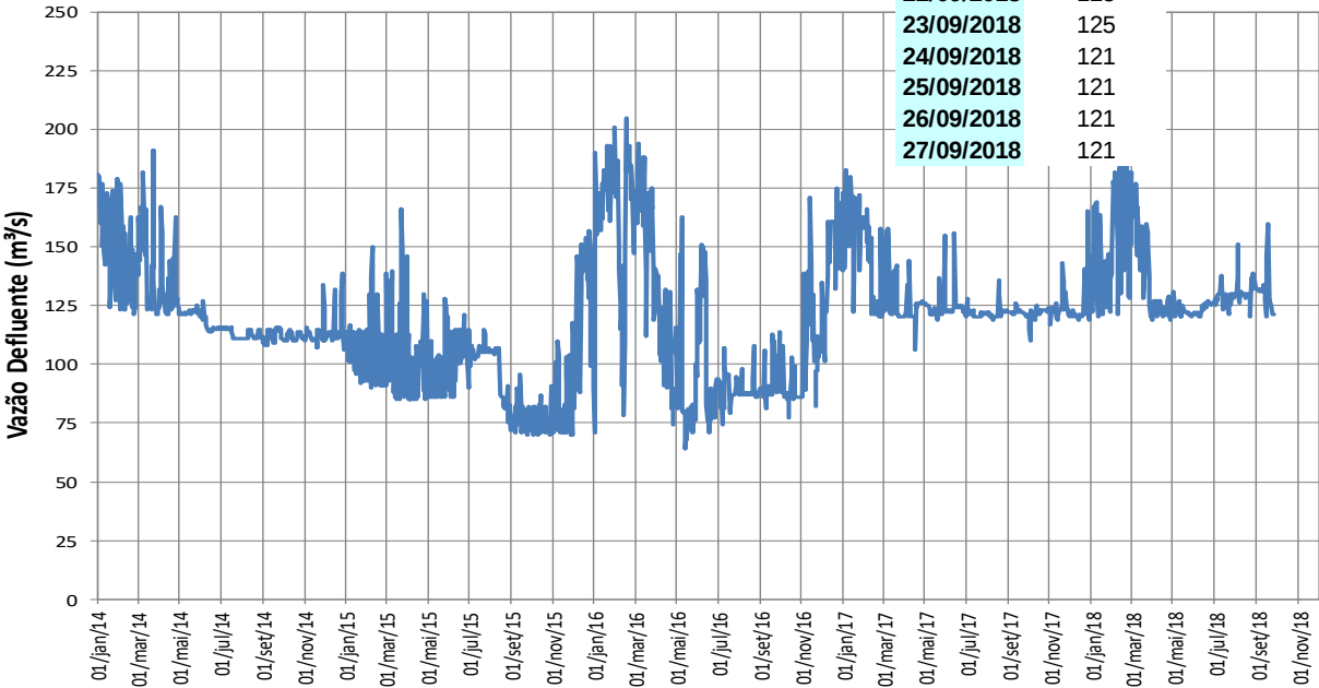
PEREIRA PASSOS - VAZÃO DEFLUENTE (m³/s)
