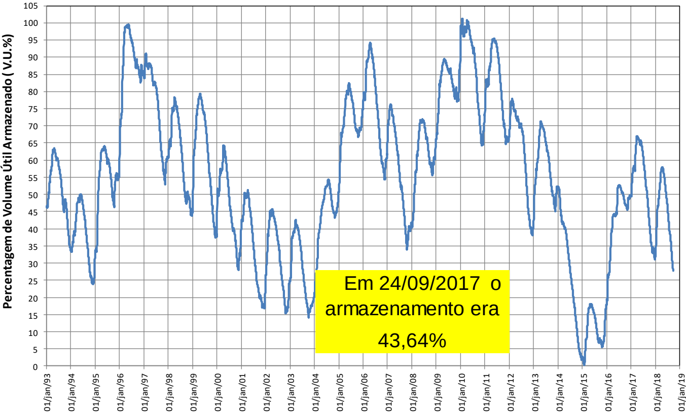
RESERVATÓRIO EQUIVALENTE
