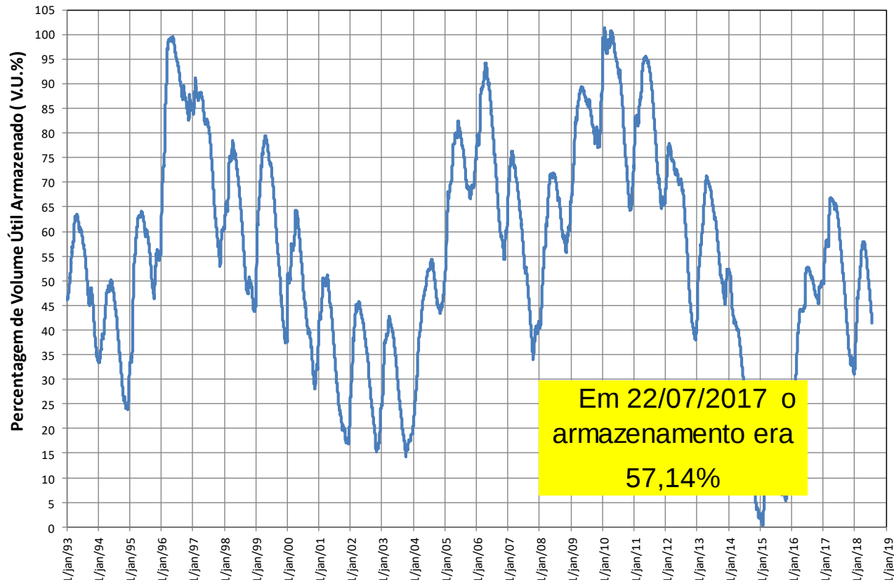
RESERVATÓRIO EQUIVALENTE
