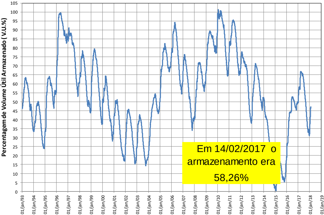
RESERVATÓRIO EQUIVALENTE
