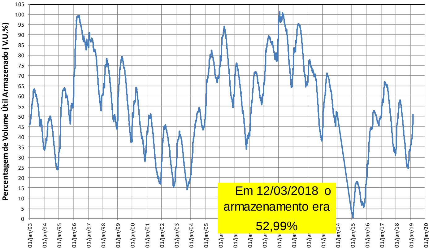
RESERVATÓRIO EQUIVALENTE
