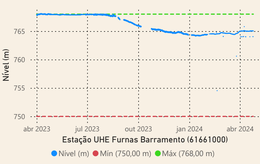
UHE Furnas
