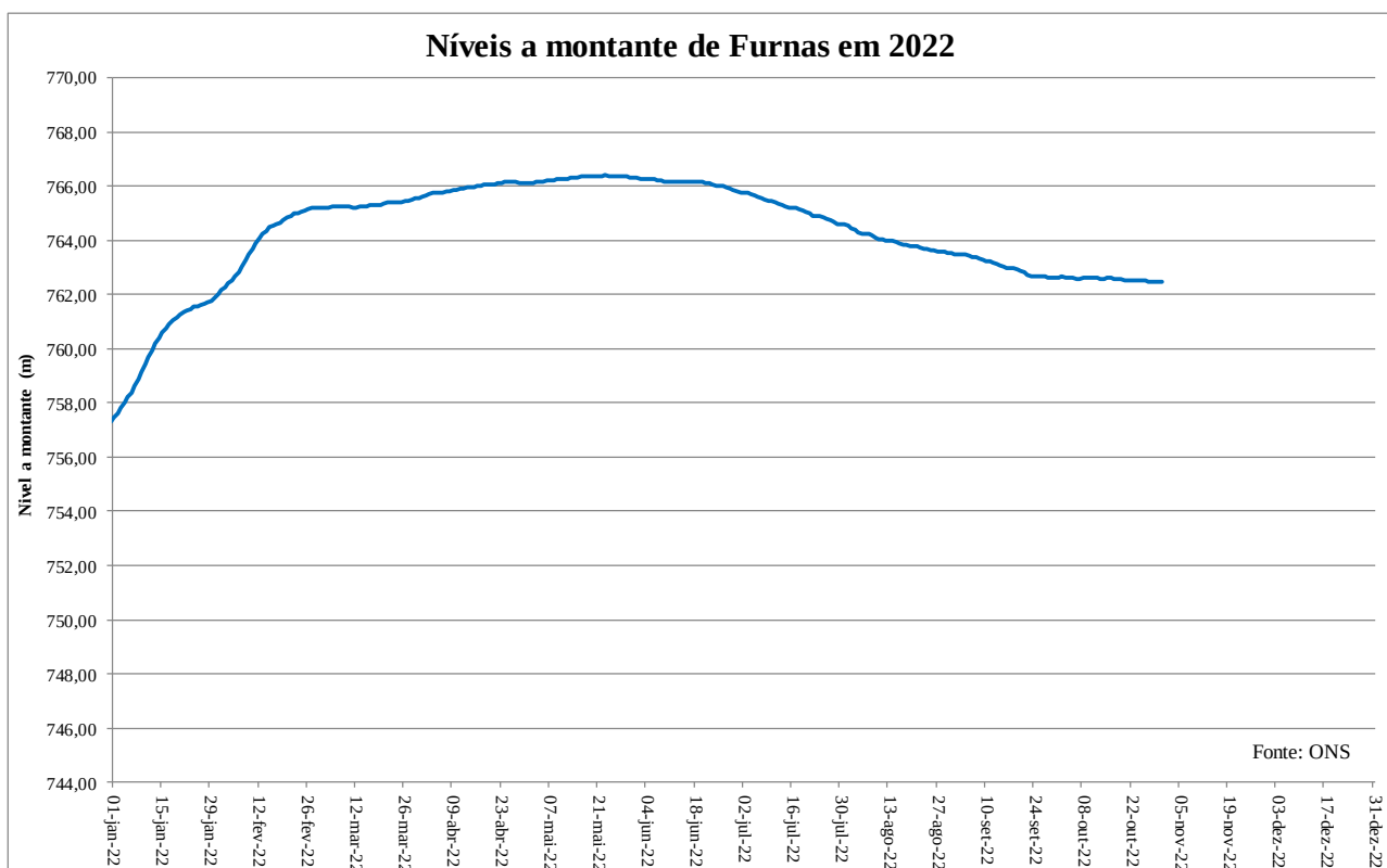
Figura 7 – Níveis a montante do reservatório de Furnas em 2022
