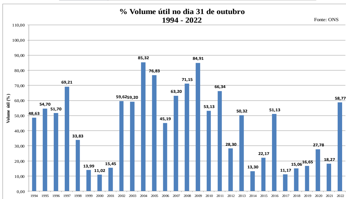
Figura 8 – Porcentagem do volume útil no dia 31 de outubro, desde 1994 até 2022
