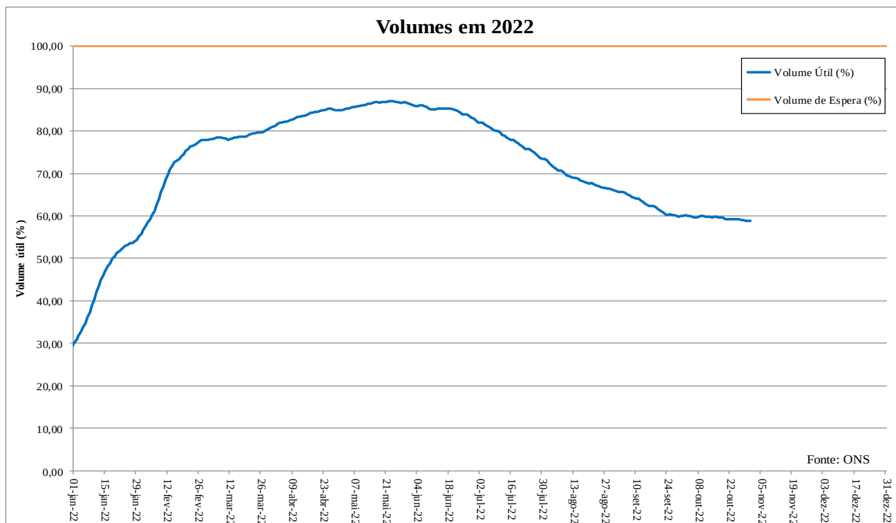
Figura 6 – Volumes no reservatório de Furnas em 2022
