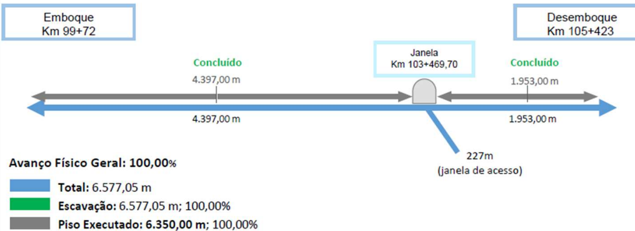
Avanço Túnel - Esquemático Extensão Total: 6.350 m (apenas túnel)
