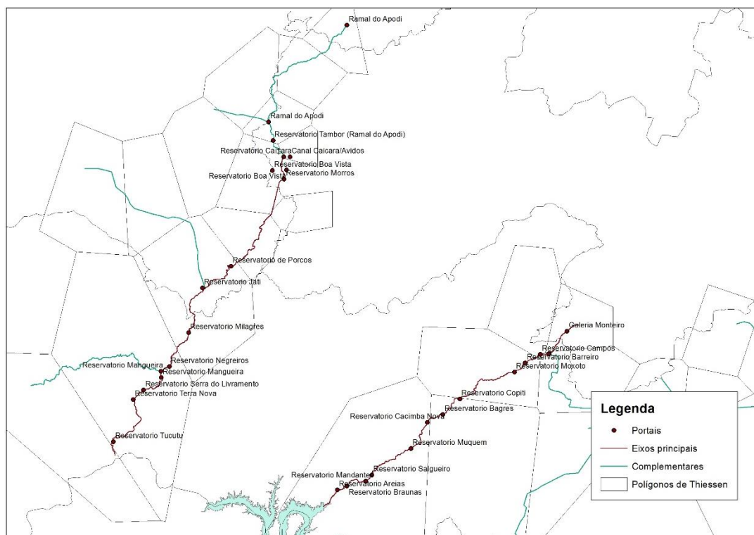
Figura 1- Polígonos de Thiessen dos vetores evaporação e traçado do PISF
