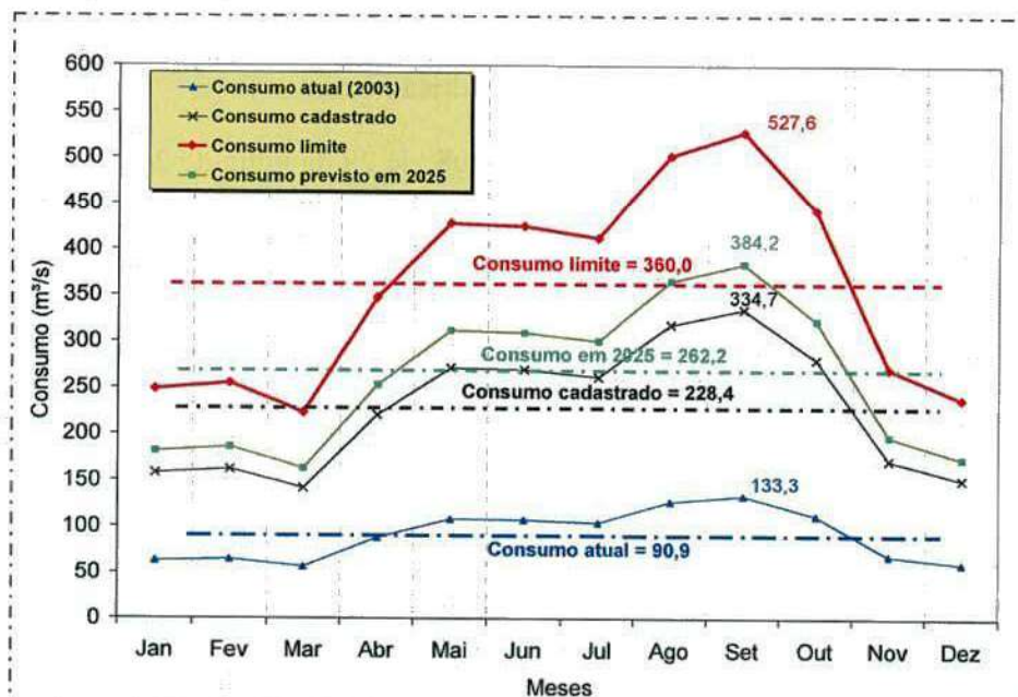
Figura 6 - Sazonalidade estimada dos consumos na bacia do rio São Francisco.
