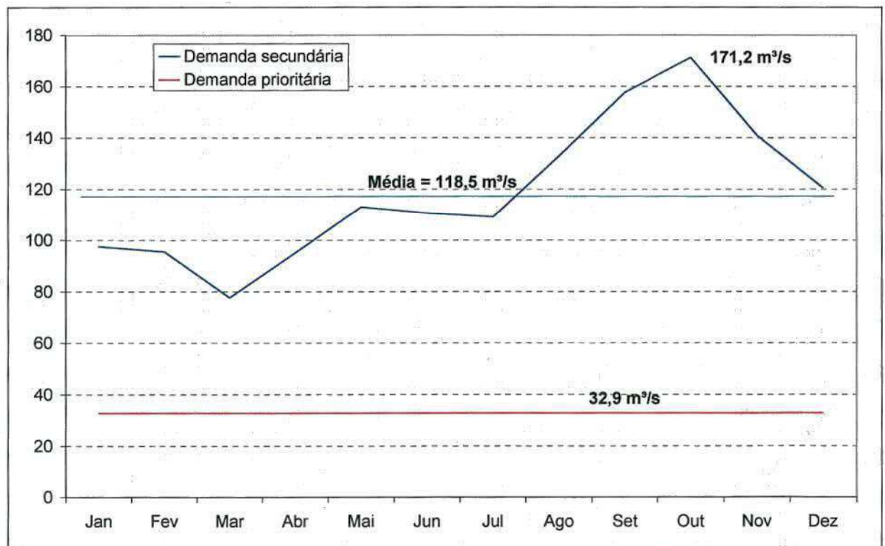
Figura 13 - Demandas hídricas totais simuladas em 2025.
