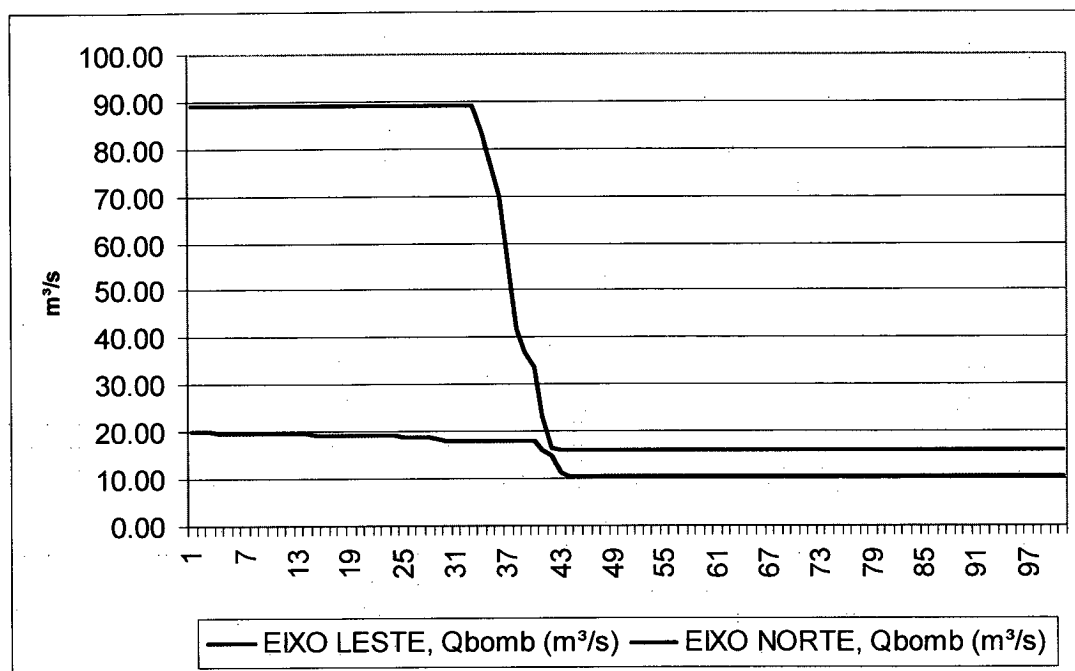
Figura 14 - Condições de bombeamento no Cenário 2005
