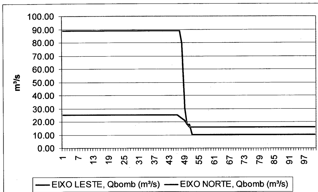
Figura 15 Condições de bombeamento no Cenário 2025
