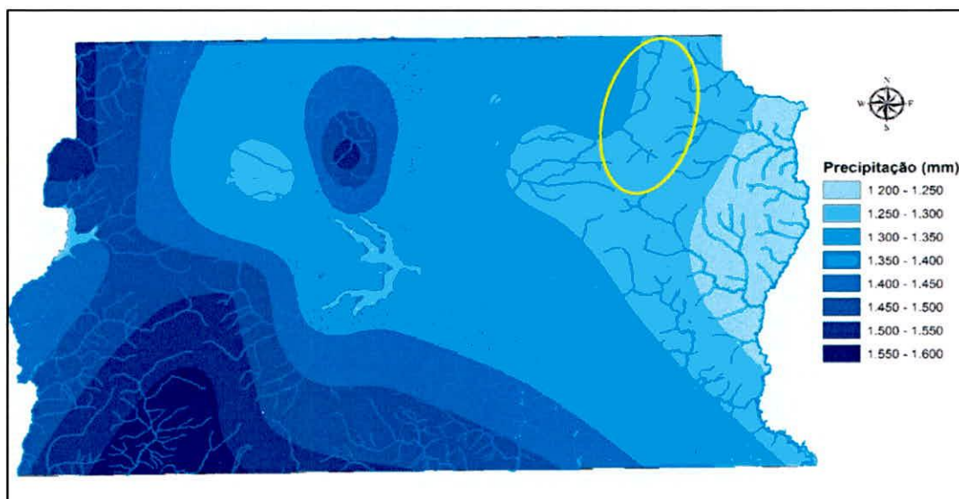
Figura 12 - Precipitação média anual (mm/ano) de 1979 a 2018.
