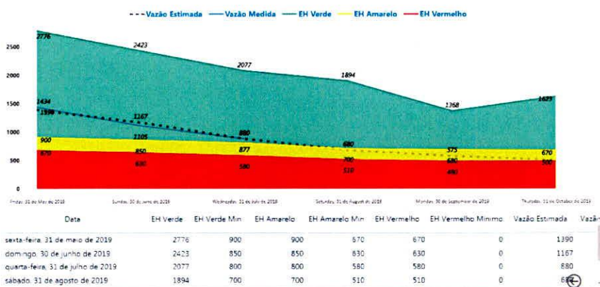
Figura 19 – Acompanhamento do comportamento do rio Pipiripau.
