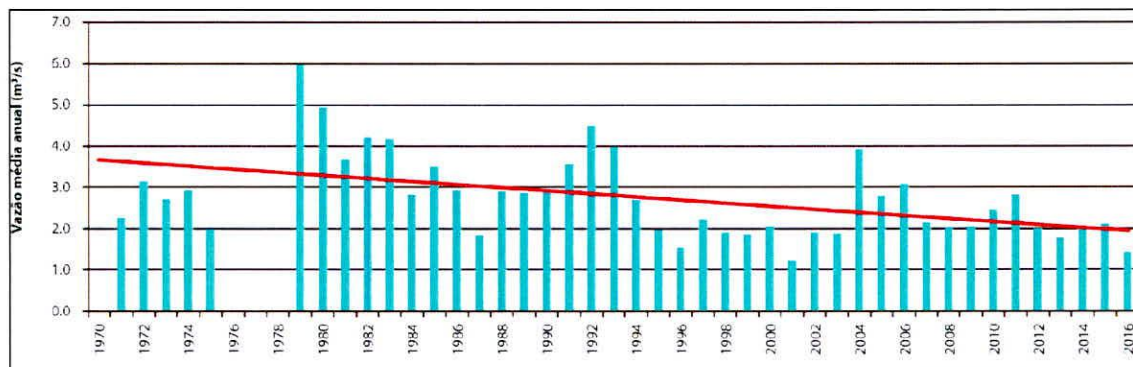
Figura 3 - Série temporal de vazões médias anuais na estação Pipiripau Frinocap DF- 130 e alinha de tendência de dados. Fonte: Maia et al., 2018, pág. 182.
