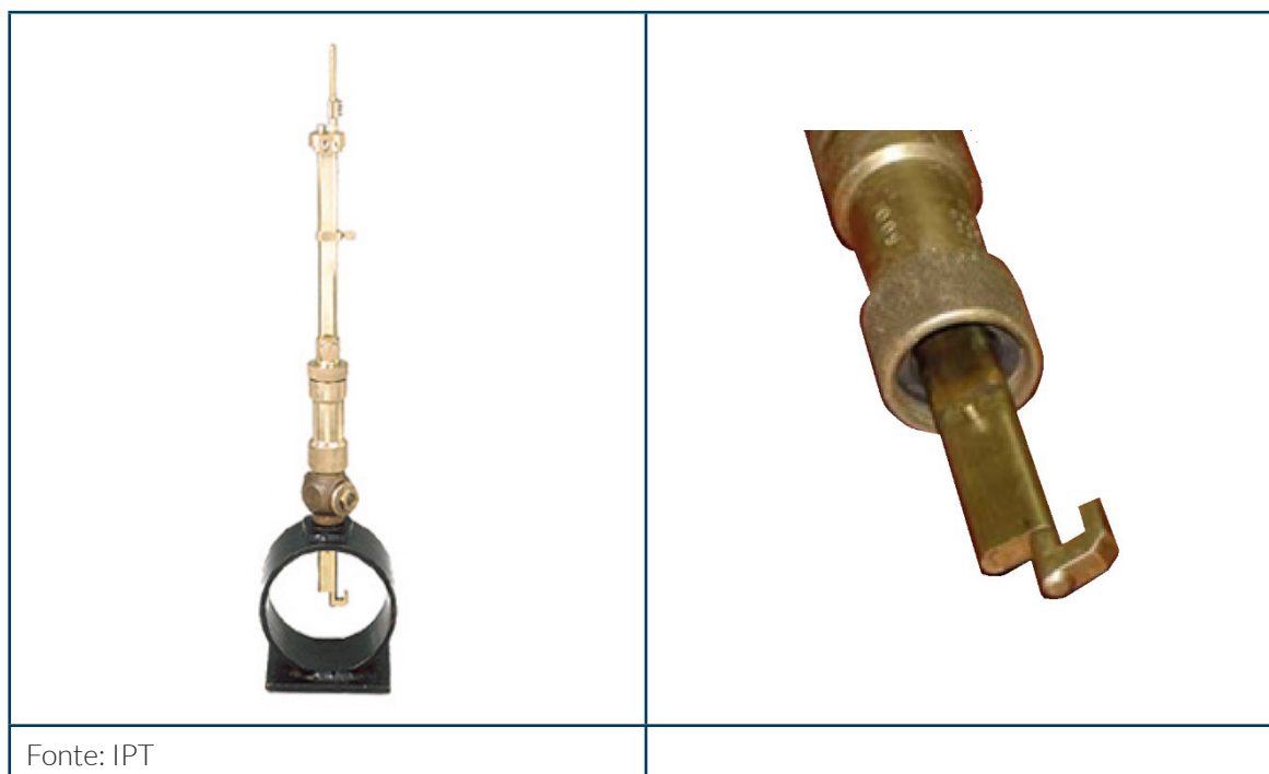
Figura 84. Calibre ou galgador de um tubo de Pitot do tipo Cole.
