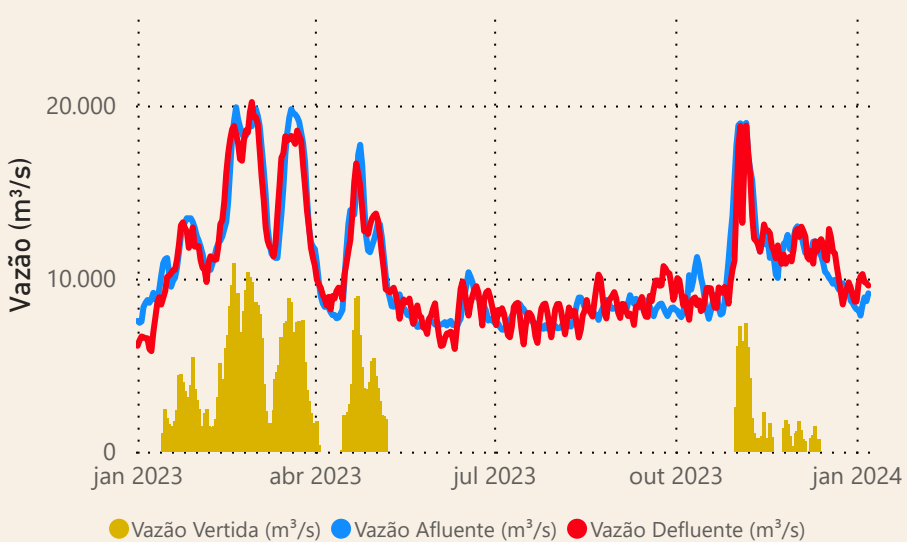
UHE Itaipu
