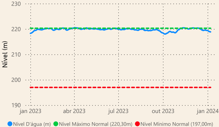
UHE Itaipu
