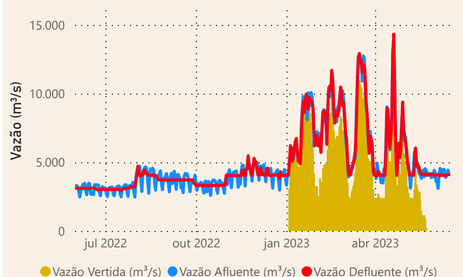
UHE Jupia
