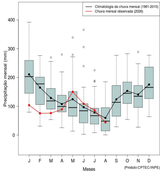
Boxplot de precipitação mensal (1981-2010): Região 112
