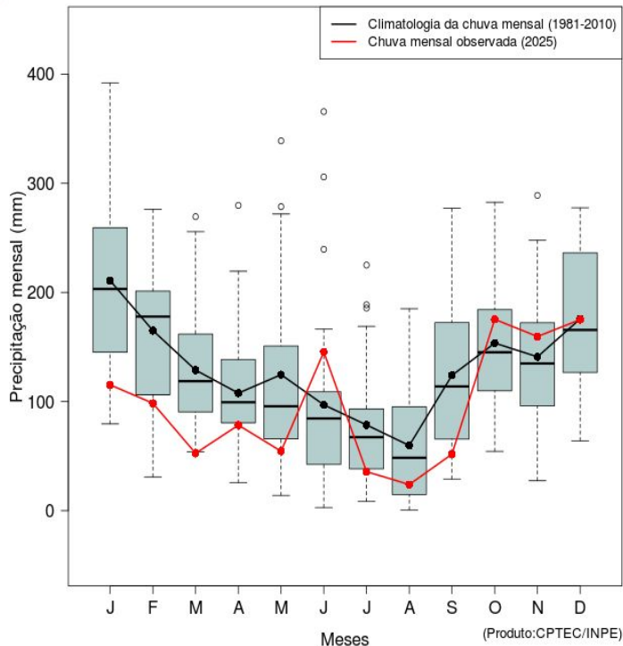
Boxplot de precipitação mensal (1981-2010): Região 112
