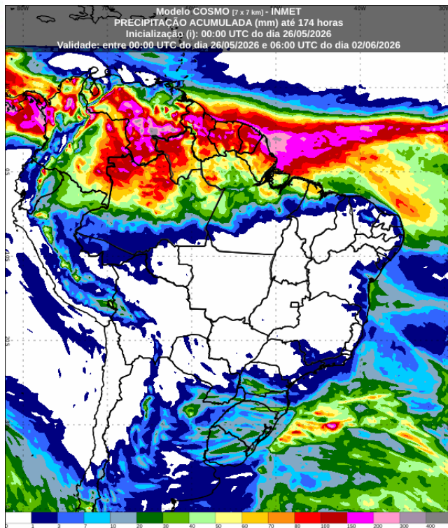
COSMO INMET
