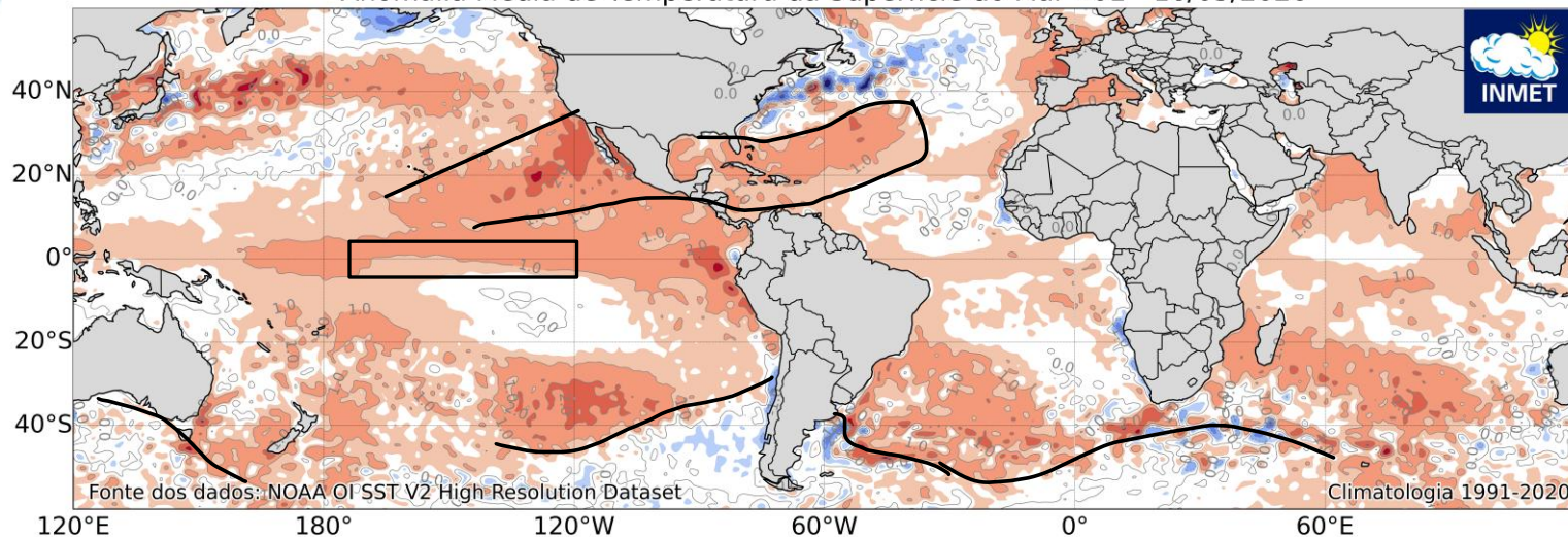
Anomalia Média de Temperatura da Superfície do Mar - 01—16/05/2026
