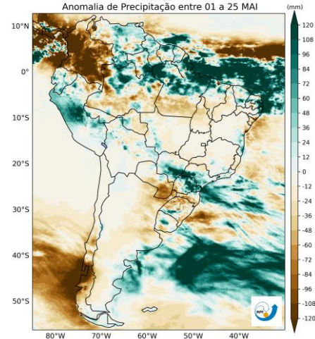
MERGE Anomalia de Precipitação entre 01 a 25 MAI
