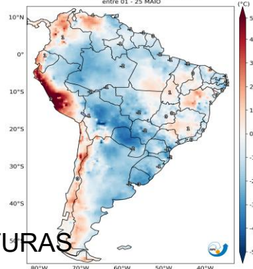
SAMeT - Anomalia da Temperatura Máxima entre 01 - 25 MAIO
