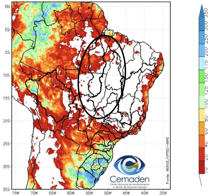
Precipitação Acumulada (mm) A.S. Período: 26/07/2026 a 25/08/2026 (30 dias)
