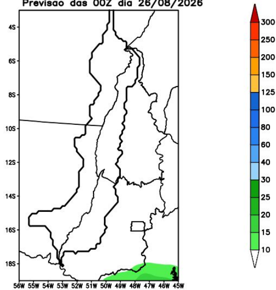
GEFS / Bacia do Rio Araguaia Precipitação acumulada em 14 dias (mm) Previsão das 00Z dia 26/08/2026
