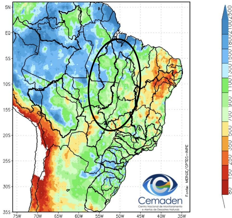
Precipitação Acumulada (mm) Ano Hidrológico Período: 01/10/2025 a 25/08/2026
