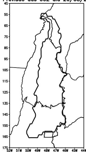
GEFS / Bacia Tocantins Precipitacao acumulada em 14 dias (mm) Previsao das 00Z dia 26/08/2026
