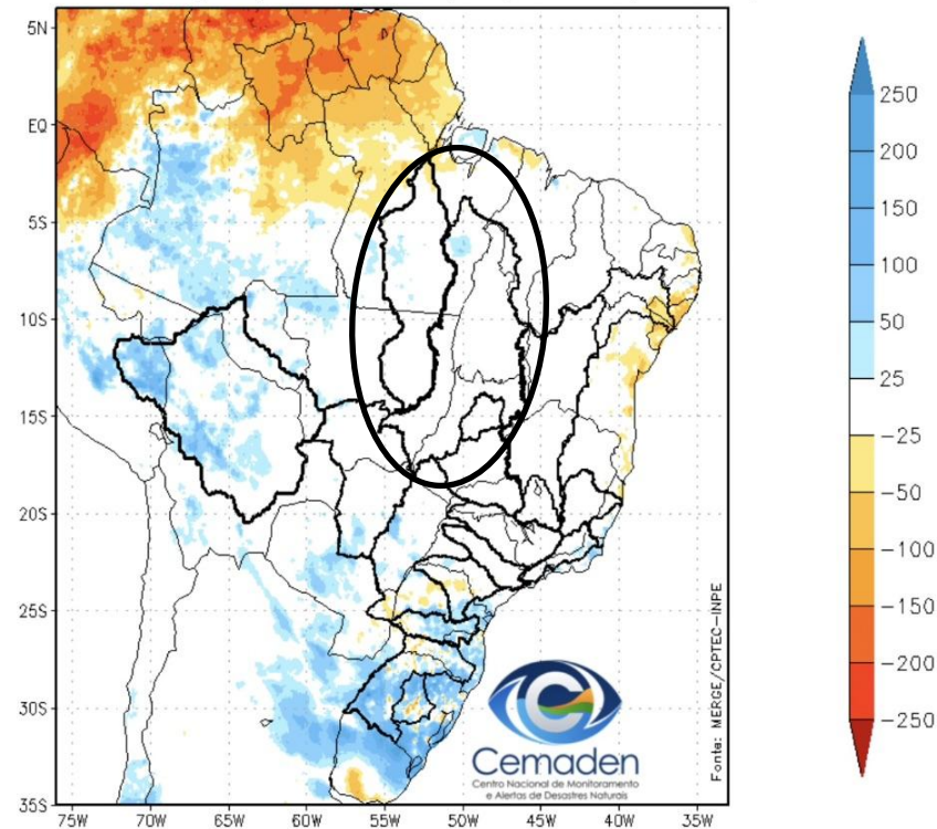
Anomalia de Precipitação (mm) A.S. Período: 26/07/2026 a 25/08/2026 (30 dias)
