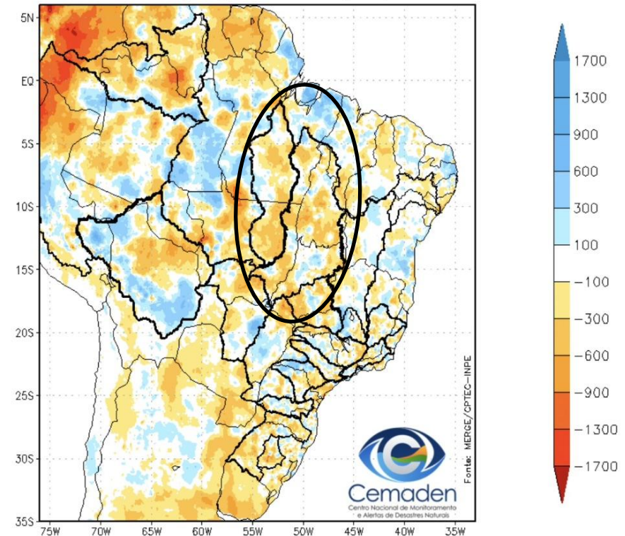
Anomalia de Precipitação (mm) Ano Hidrológico Período: 01/10/2025 a 25/08/2026
