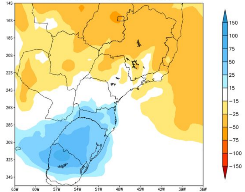
Anomalia de Precipitacao BR SUL (mm) Periodo: 2023112912 a 2023120512
