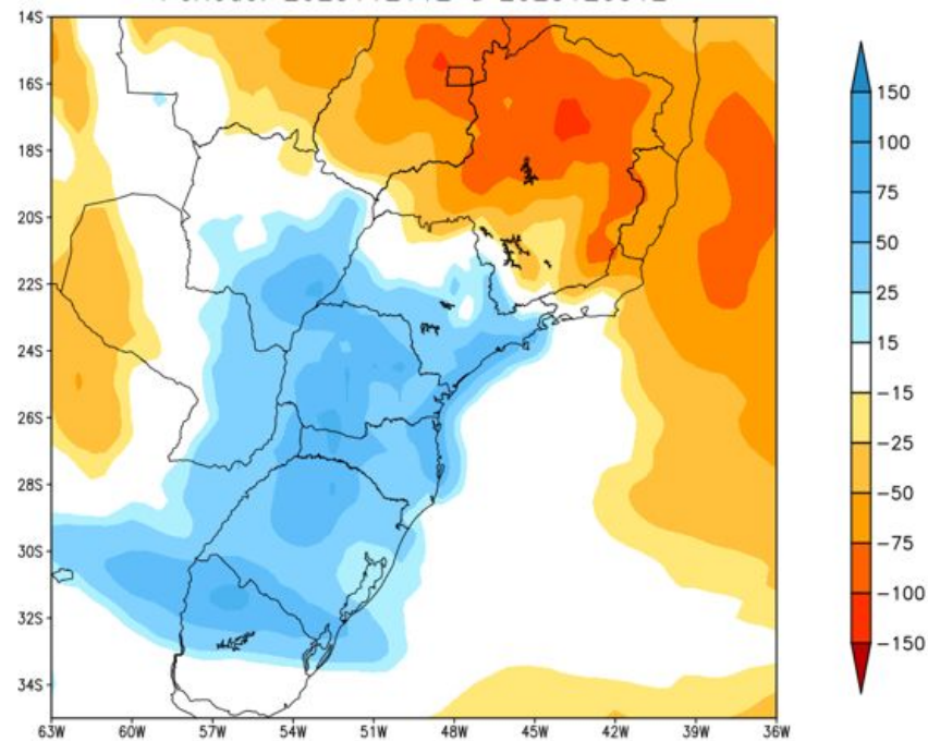
Anomalia de Precipitacao BR_SUL (mm) Periodo: 2023112112 a 2023120512
