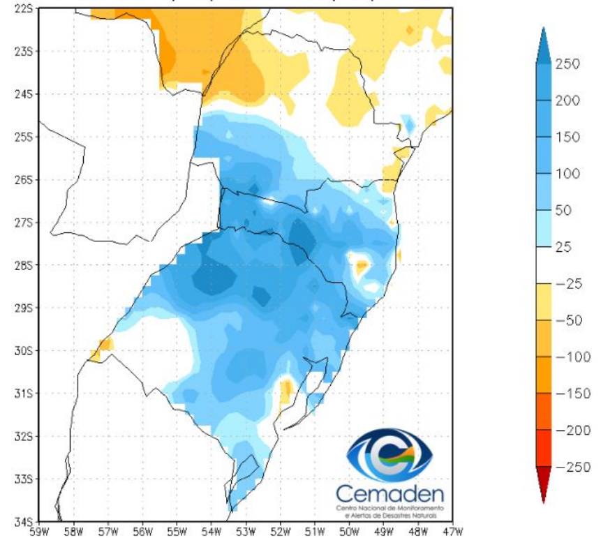
Anomalia de Precipitação (mm) Período: 01/11/2023 a 21/11/2023
