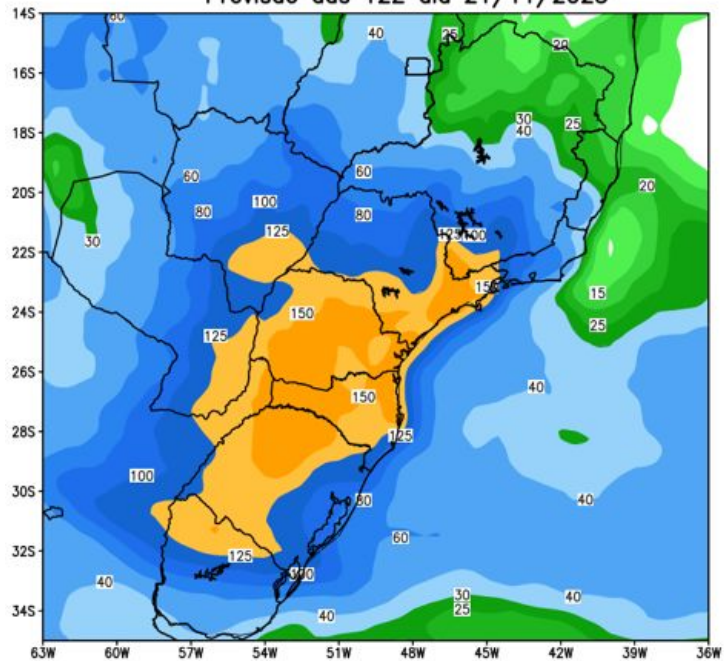
GEFS / BRASIL_SUL Precipitacao acumulada 14dias (mm) Previsao das 12Z dia 21/11/2023
