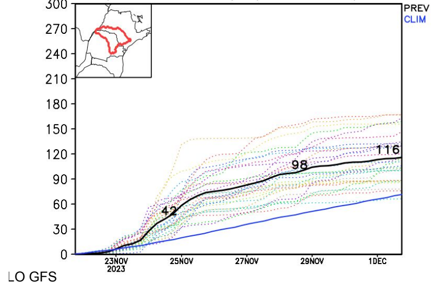
Precipitação acumulada (mm): Bacia Paranapanema
