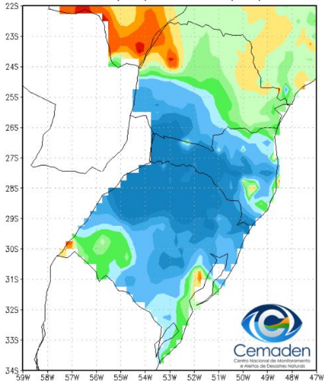
Precipitação Acumulada (mm) Período: 01/11/2023 a 21/11/2023
