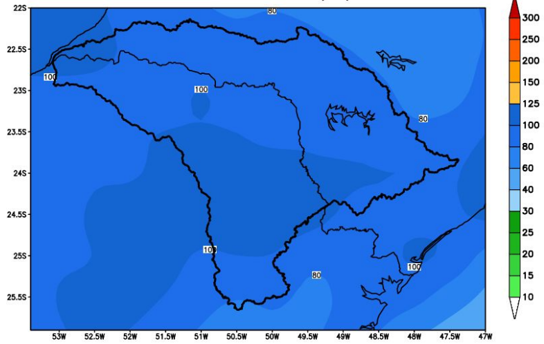
GEFS / Bacia do Rio Paranapanema Precipitação acumulada em 7 dias (mm) Previsão das 12Z dia 21/11/2023
