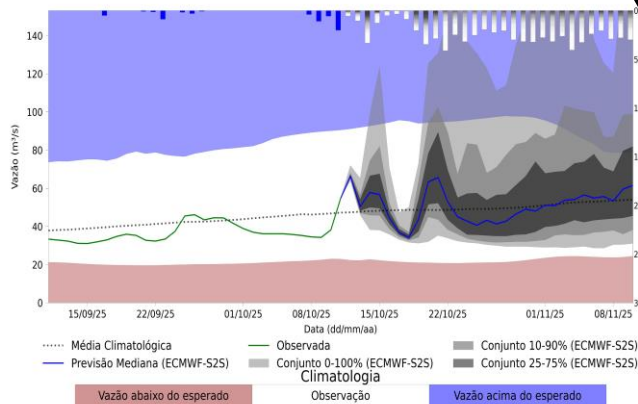
UHE Paraibuna
