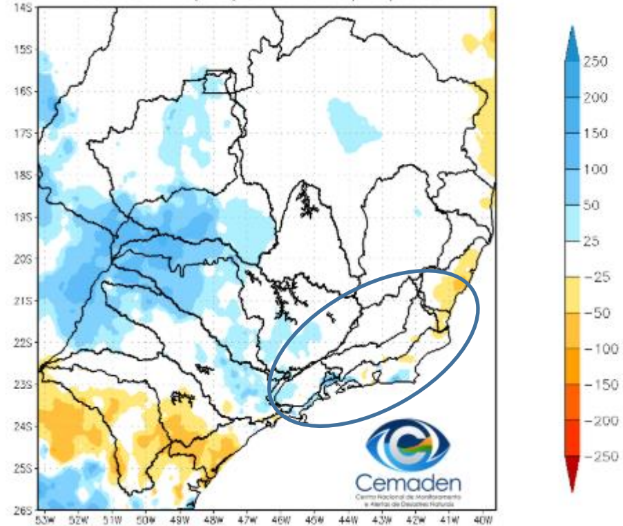
Anomalia de Precipitação (mm) A.S. Período: 13/06/2026 a 13/07/2026
