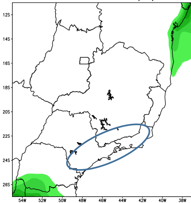
GEFS / BRASIL_SE Precipitacao acumulada 1aSem (mm) Previsao das 00Z dia 14/07/2026
