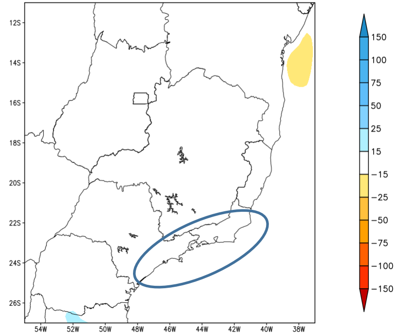
Anomalia de Precipitacao BR SE (mm) Periodo: 2026072200 a 2026072800
