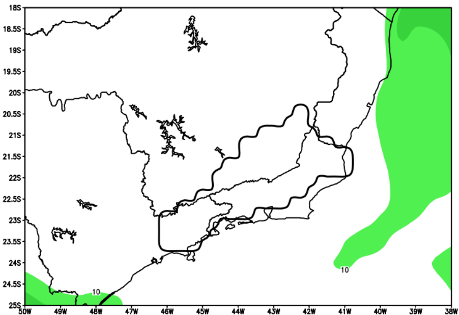
GEFS / Bacia do Rio Paraíba do Sul Precipitação acumulada em 14 dias (mm) Previsão das 00Z dia 14/07/2026
