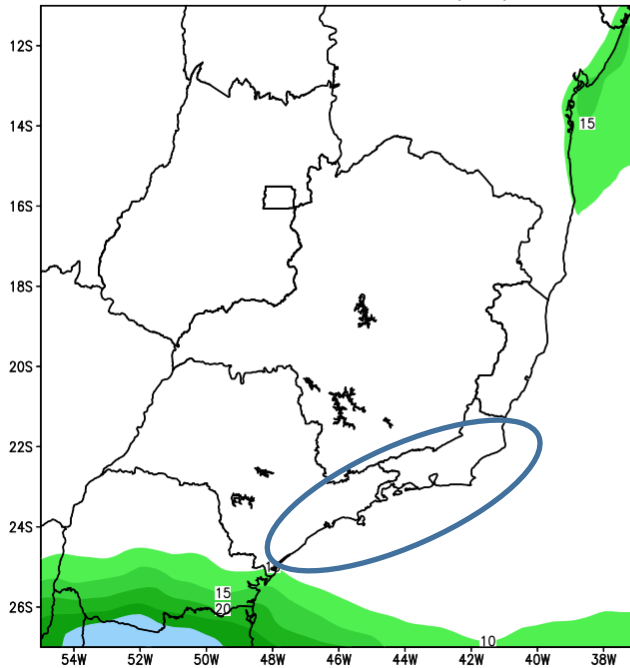
GEFS / BRASIL_SE Precipitacao acumulada 2aSem (mm) Previsao das 00Z dia 14/07/2026
