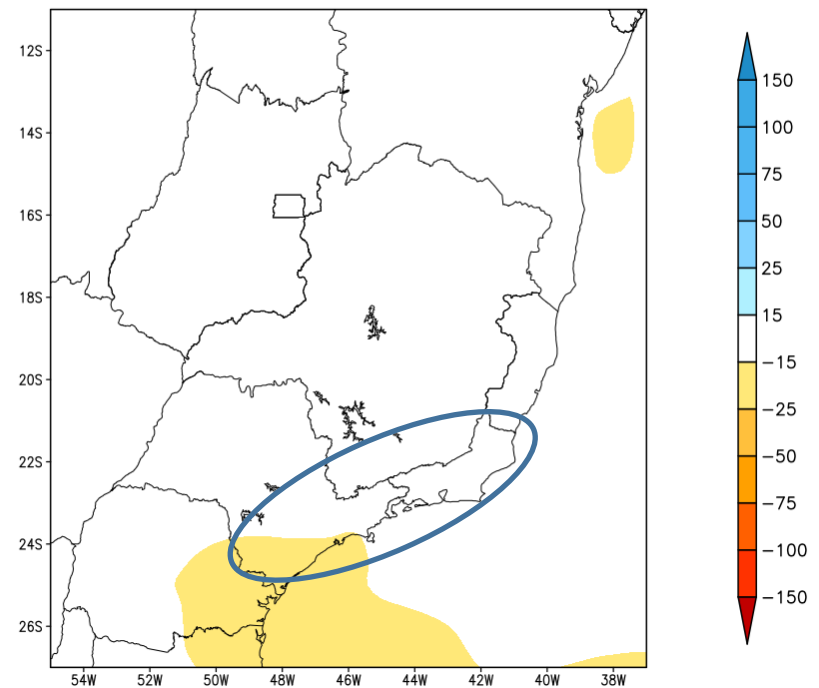
Anomalia de Precipitacao BR_SE (mm) Periodo: 2026071400 a 2026072100
