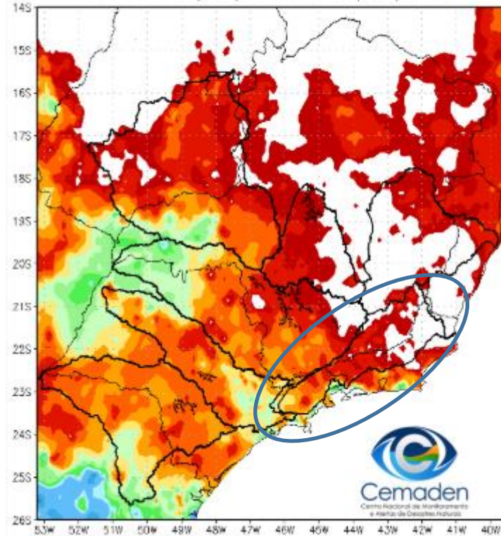
Precipitação Acumulada (mm) A.S. Período: 13/06/2026 a 13/07/2026
