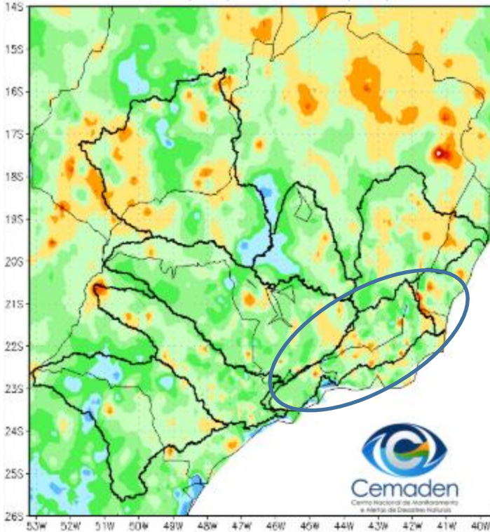
Precipitação Acumulada (mm) A.S. Período: 01/10/2025 a 13/07/2026
