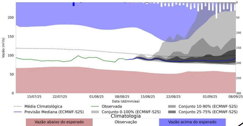
UHE Funil
