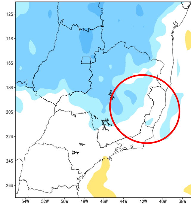
Anomalia de Precipitacao BR_SE (mm) Periodo: 2024040300 a 2024040900
