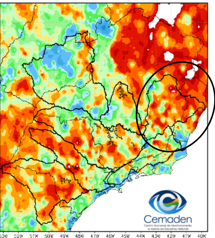
Precipitação Acumulada (mm) A.S. Período: 24/02/2024 a 25/03/2024
