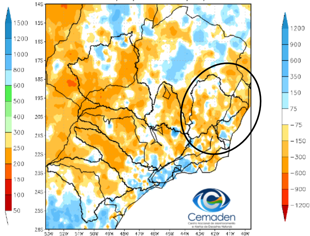
Anomalia de Precipitação (mm) A.S. Período: 01/10/2023 a 25/03/2024
