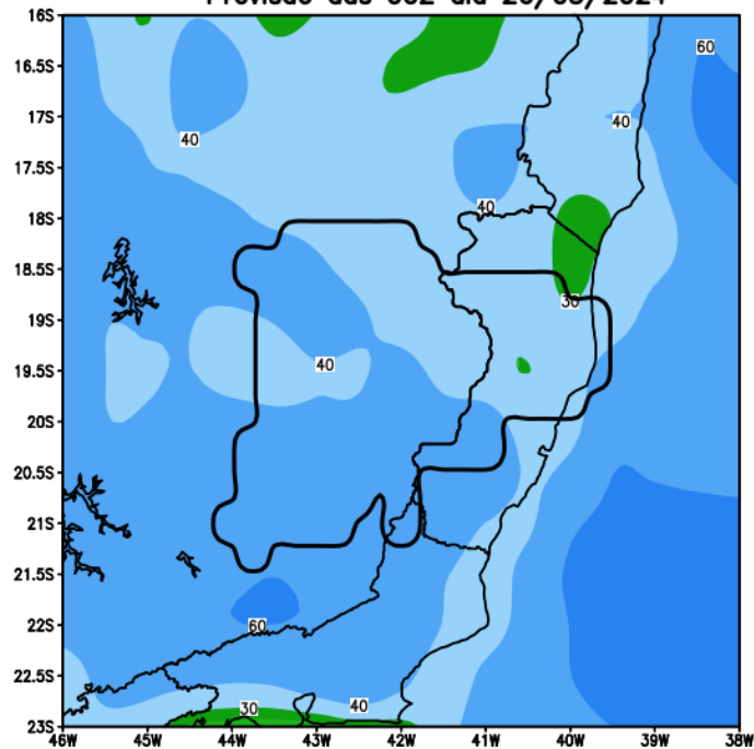
GEFS / Bacia do Rio Doce Precipitacao acumulada em 7 dias (mm) Previsao das 00Z dia 26/03/2024
