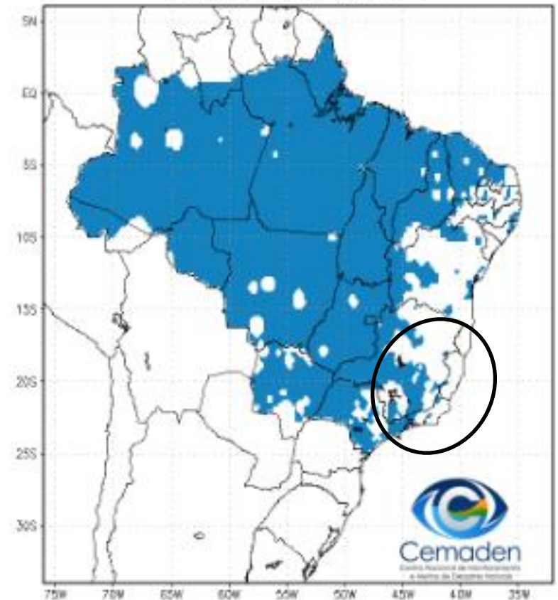
Precipitação Inferior 2 mm/dia por 4 de 5 dias Período: 25/03/2024
