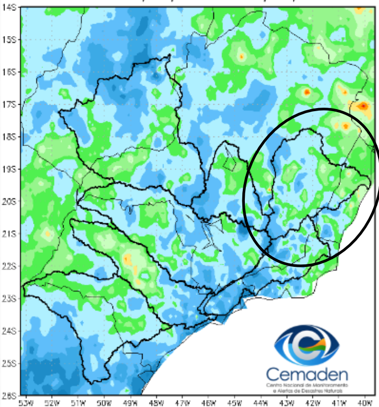
Precipitação Acumulada (mm) A.S. Período: 01/10/2023 a 25/03/2024
