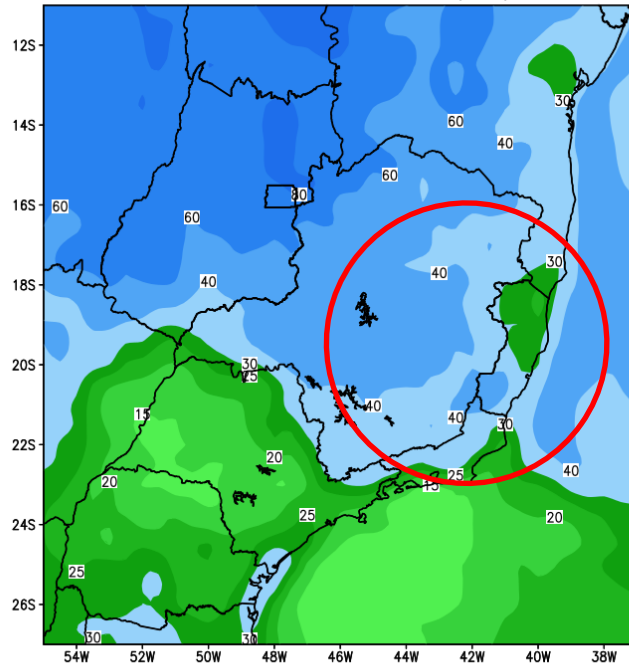
GEFS / BRASIL_SE Precipitacao acumulada 2aSem (mm) Previsao das 00Z dia 26/03/2024
