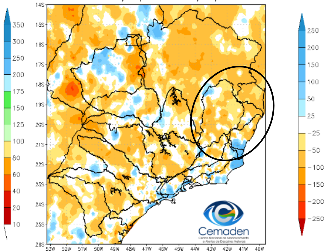
Anomalia de Precipitação (mm) A.S. Período: 24/02/2024 a 25/03/2024
