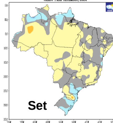
PREVISÃO DE ANOMALIAS DE PRECIPITAÇÃO (mm) ATUALIZAÇÃO - JULHO/2024 VÁLIDO PARA SETEMBRO/2024
