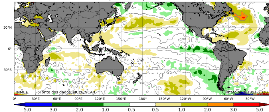
Anomalia da Temperatura da Superfície do Mar - 16-30/06/2024
