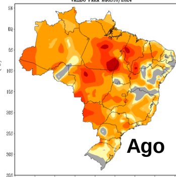
PREVISÃO DE ANOMALIAS DE TEMPERATURA (°C) ATUALIZAÇÃO - JULHO/2024 VÁLIDO PARA AGOSTO/2024
