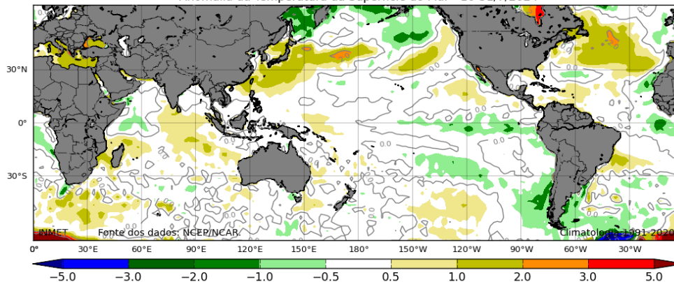
Anomalia da Temperatura da Superfície do Mar - 16-31/7/2024
