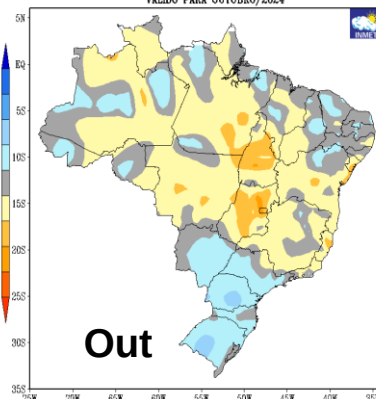
PREVISÃO DE ANOMALIAS DE PRECIPITAÇÃO (mm) ATUALIZAÇÃO - JULHO/2024 VÁLIDO PARA OUTUBRO/2024
