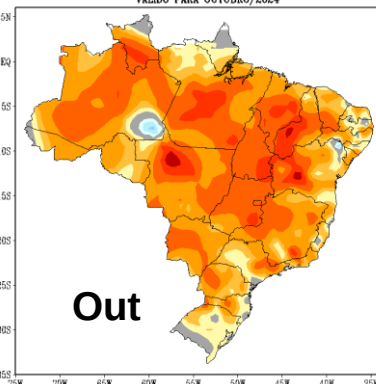
PREVISÃO DE ANOMALIAS DE TEMPERATURA (°C) ATUALIZAÇÃO - JULHO/2024 VÁLIDO PARA OUTUBRO/2024
