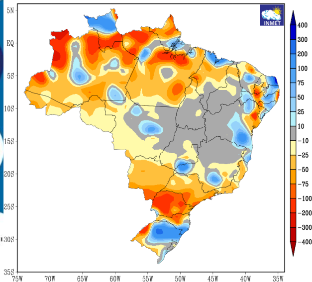
ANOMALIA DE PRECIPITAÇÃO VALIDO PARA JUNHO DE 2024
