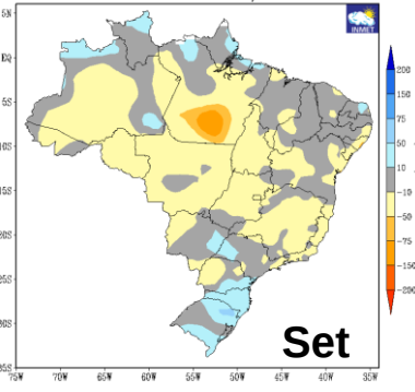
PREVISÃO DE ANOMALIAS DE PRECIPITAÇÃO (mm) ATUALIZAÇÃO - JUNHO/2024 VALIDO PARA SETEMBRO/2024
