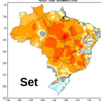
PREVISÃO DE ANOMALIAS DE TEMPERATURA (°C) ATUALIZAÇÃO - JULHO/2024 VÁLIDO PARA SETEMBRO/2024
