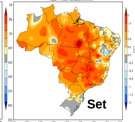
PREVISÃO DE ANOMALIAS DE TEMPERATURA (°C) ATUALIZAÇÃO - JUNHO/2024 VALIDO PARA SETEMBRO/2024
