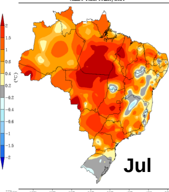
PREVISÃO DE ANOMALIAS DE TEMPERATURA (°C) ATUALIZAÇÃO - JUNHO/2024 VALIDO PARA JULHO/2024
