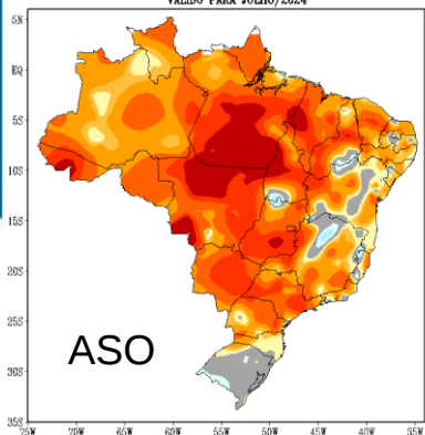
PREVISÃO DE ANOMALIAS DE TEMPERATURA (°C) ATUALIZAÇÃO - JULHO/2024 VÁLIDO PARA JULHO/2024
