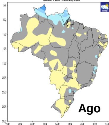
PREVISÃO DE ANOMALIAS DE PRECIPITAÇÃO (mm) ATUALIZAÇÃO - JULHO/2024 VÁLIDO PARA AGOSTO/2024
