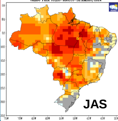
PREVISÃO DE ANOMALIAS DE TEMPERATURA (°C) ATUALIZAÇÃO - JUNHO/2024 VALIDO PARA JULHO-AGOSTO-SETEMBRO/2024
