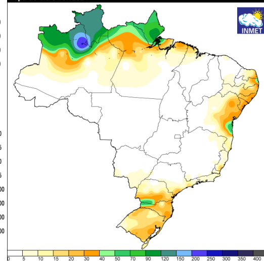
Instituto Nacional de Meteorologia - INMET Precipitação Acumulada nos últimos 15 dias Mapa do dia 31/07/2024
