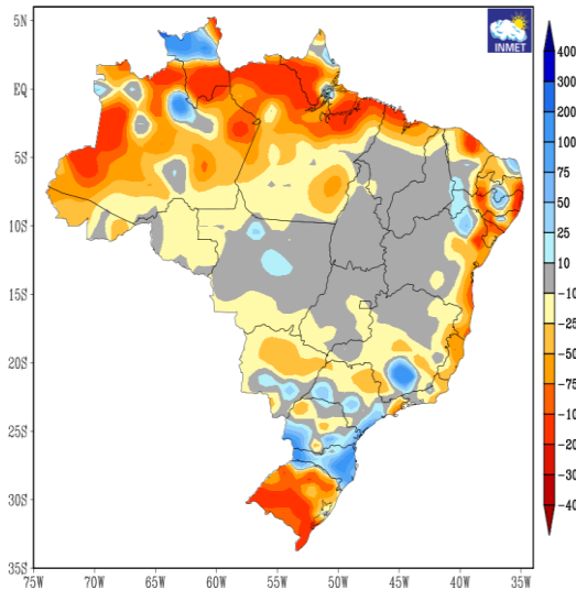
ANOMALIA DE PRECIPITAÇÃO VALIDO PARA JULHO DE 2024
