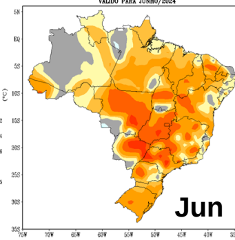
PREVISÃO DE ANOMALIAS DE TEMPERATURA (°C) ATUALIZAÇÃO - MARÇO/2024 VÁLIDO PARA JUNHO/2024
