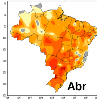
PREVISÃO DE ANOMALIAS DE TEMPERATURA (°C) ATUALIZAÇÃO - MARÇO/2024 VÁLIDO PARA ABRIL/2024
