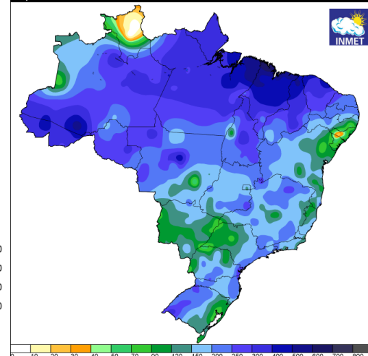
Instituto Nacional de Meteorologia - INMET Precipitação Acumulada nos últimos 30 dias Mapa do dia 19/03/2024
