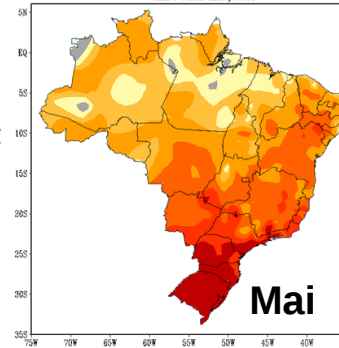
PREVISÃO DE ANOMALIAS DE TEMPERATURA (°C) ATUALIZAÇÃO - MARÇO/2024 VÁLIDO PARA MAIO/2024
