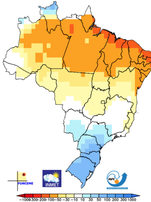
Previsão de Anomalia de Precipitação AMJ/2024 média [CPTEC1.2+INMET+FUNCEME]
