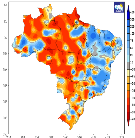
ANOMALIA DE PRECIPITAÇÃO VALIDO PARA FEVEREIRO DE 2024
