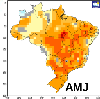
PREVISÃO DE ANOMALIAS DE TEMPERATURA (°C) ATUALIZAÇÃO - MARÇO/2024 VÁLIDO PARA ABRIL-MAIO-JUNHO/2024
