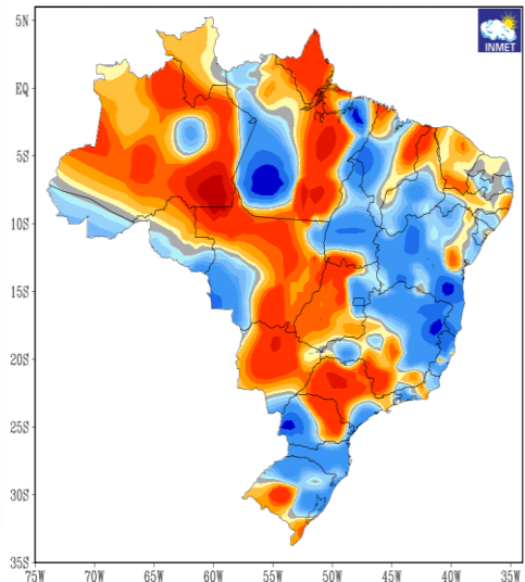
ANOMALIA DE PRECIPITAÇÃO VALIDO PARA JANEIRO DE 2024
