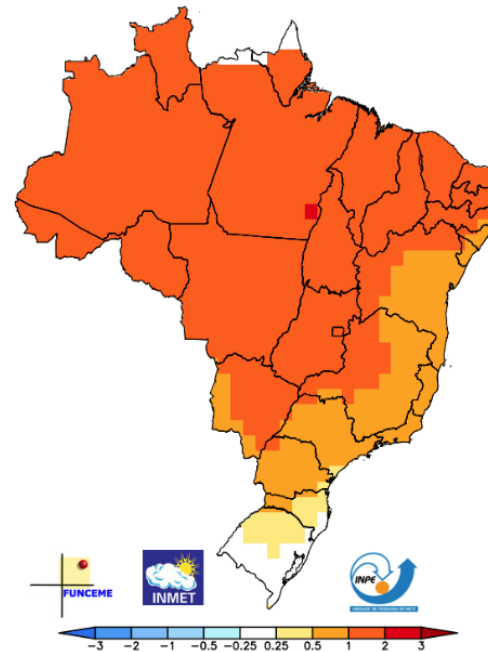
Previsão de Anomalia de Temperatura AMJ/2024 média [CPTEC1.2+INMET+FUNCEME]
