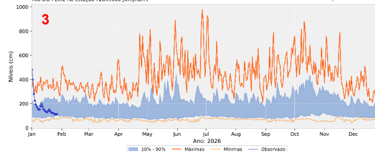
Níveis observados e comparação com histórico RIO DO PEIXE na estação 72849000 JOAÇABA I
