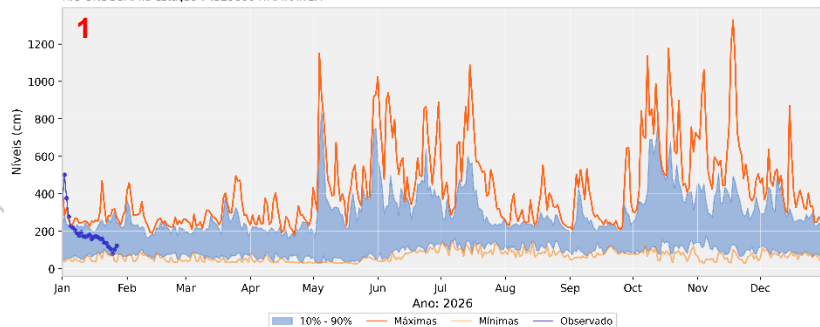
Níveis observados e comparação com histórico RIO URUGUAI na estação 74329000 ITAPIRANGA
