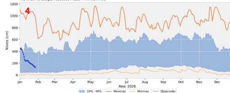
Níveis observados e comparação com histórico RIO IBICUI na estação 76800000 PASSO MARIANO PINTO
