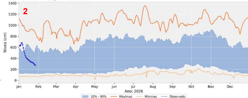
Níveis observados e comparação com histórico RIO URUGUAI na estação 77150000 URUGUAIANA
