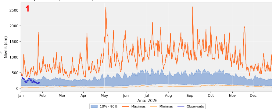
Níveis observados e comparação com histórico RIO TAQUARI na estação 86510000 MUÇUM
