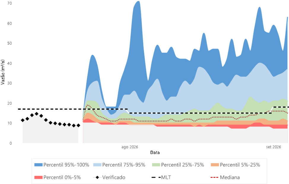
Acompanhamento da previsão de vazão natural G. P SOUZA
