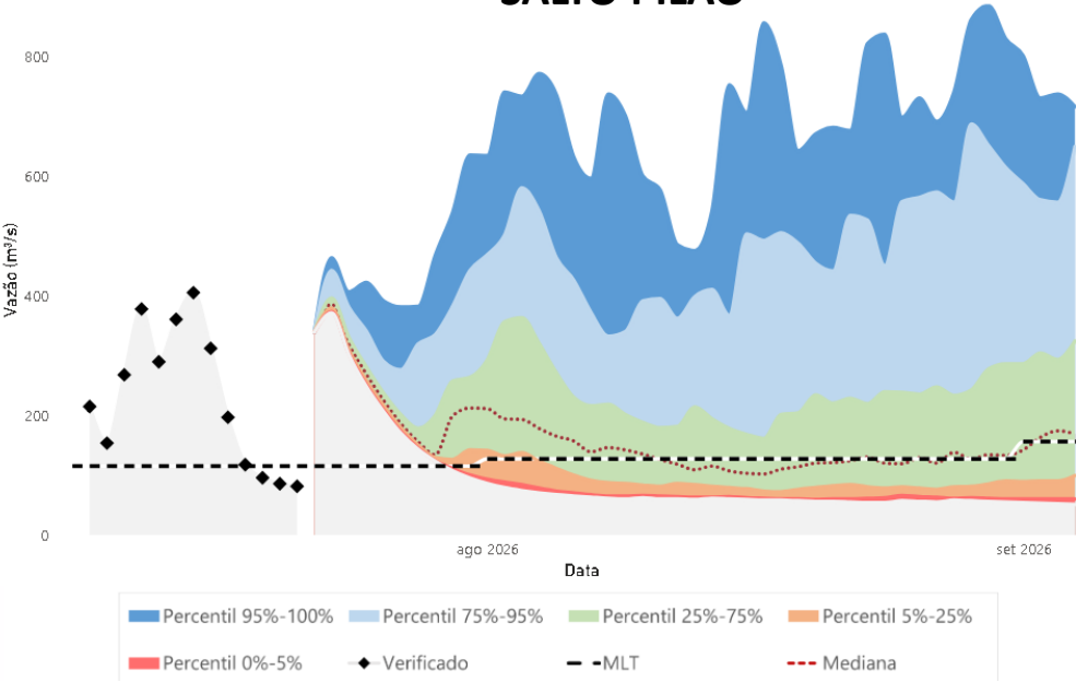
Acompanhamento da previsão de vazão natural SALTO PILAO
