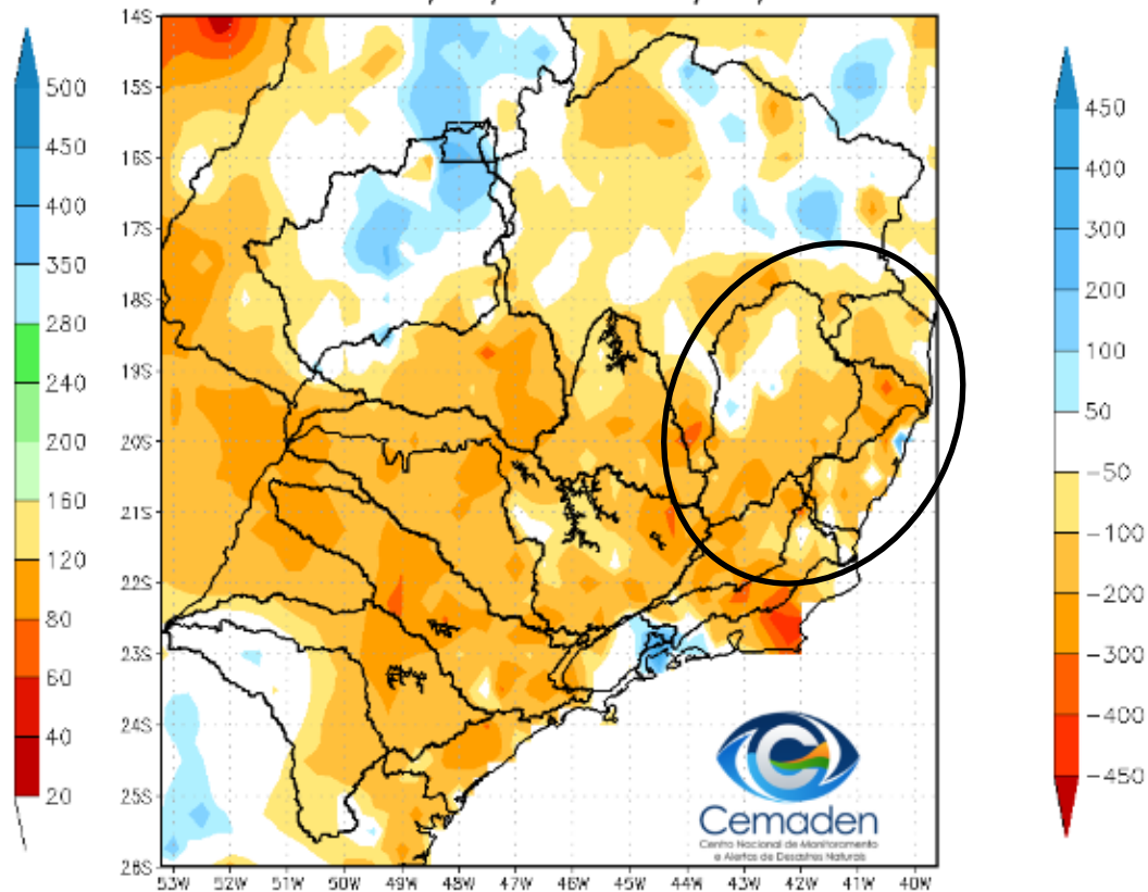
Anomalia de Precipitação (mm) A.S. Período: 26/11/2023 a 25/01/2024
