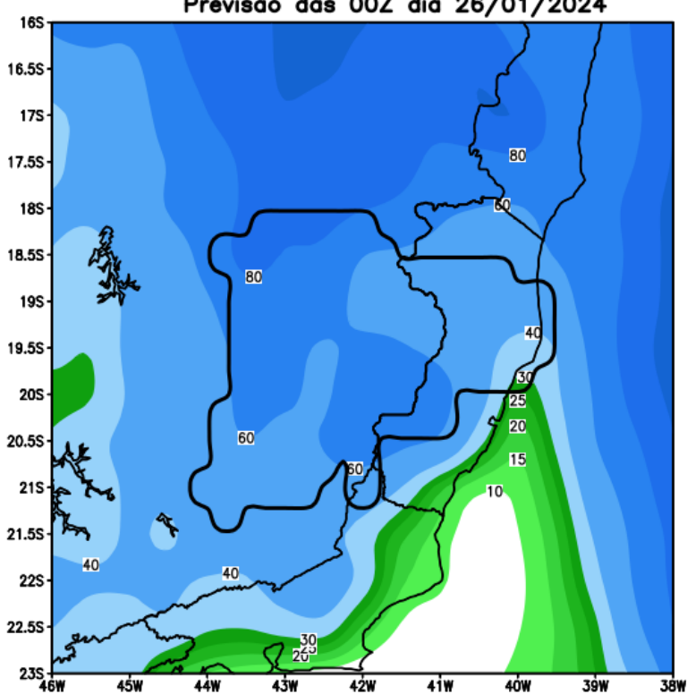
GEFS / Bacia do Rio Doce Precipitacao acumulada em 7 dias (mm) Previsao das 00Z dia 26/01/2024
