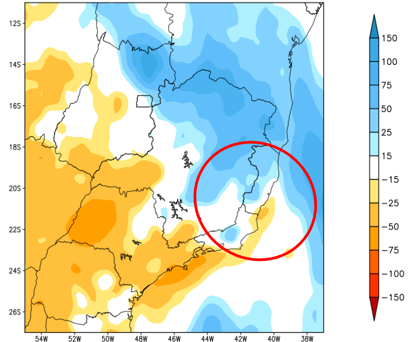
Anomalia de Precipitacao BR SE (mm) Periodo: 2024012600 a 2024020900
