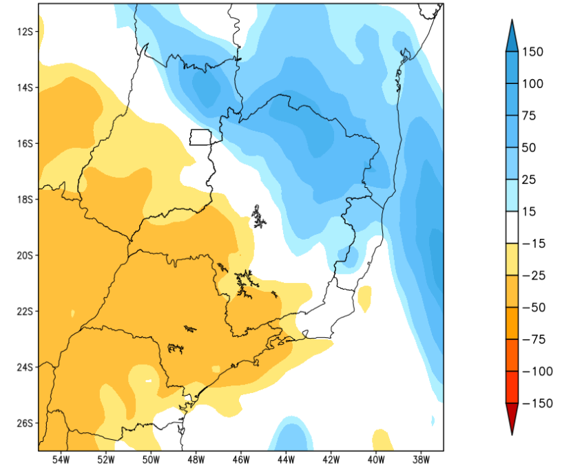
Anomalia de Precipitacao BR SE (mm) Periodo: 2024012600 a 2024020200
