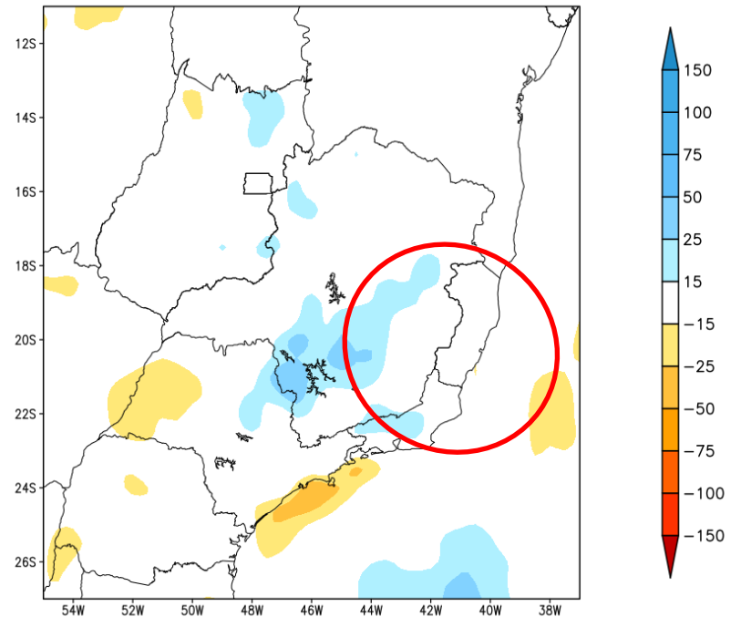
Anomalia de Precipitacao BR SE (mm) Periodo: 2024020300 a 2024020900
