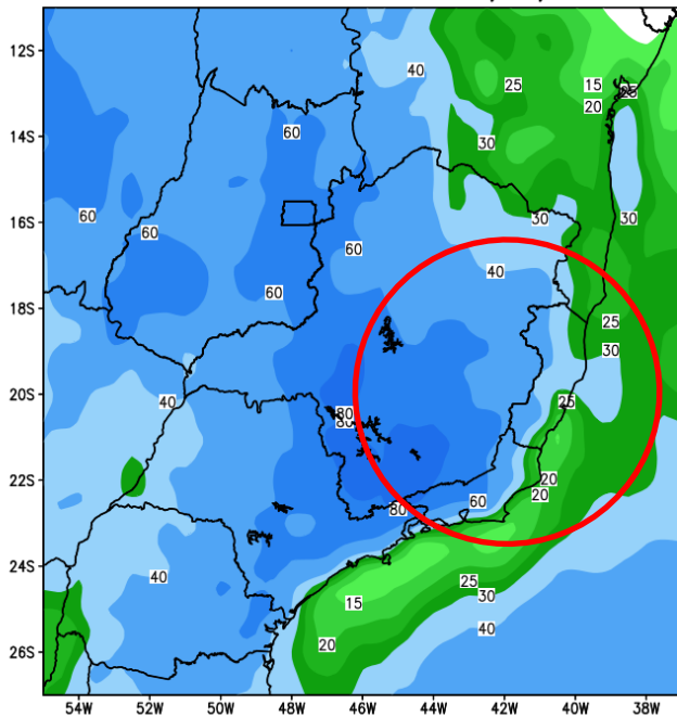
GEFS / BRASIL_SE Precipitacao acumulada 2aSem (mm) Previsao das 00Z dia 26/01/2024
