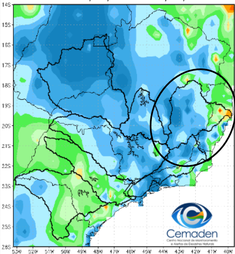
Precipitação Acumulada (mm) A.S. Período: 26/11/2023 a 25/01/2024
