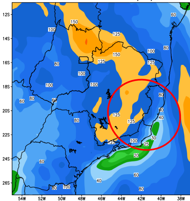
GEFS / BRASIL_SE Precipitacao acumulada 14dias (mm) Previsao das 00Z dia 26/01/2024
