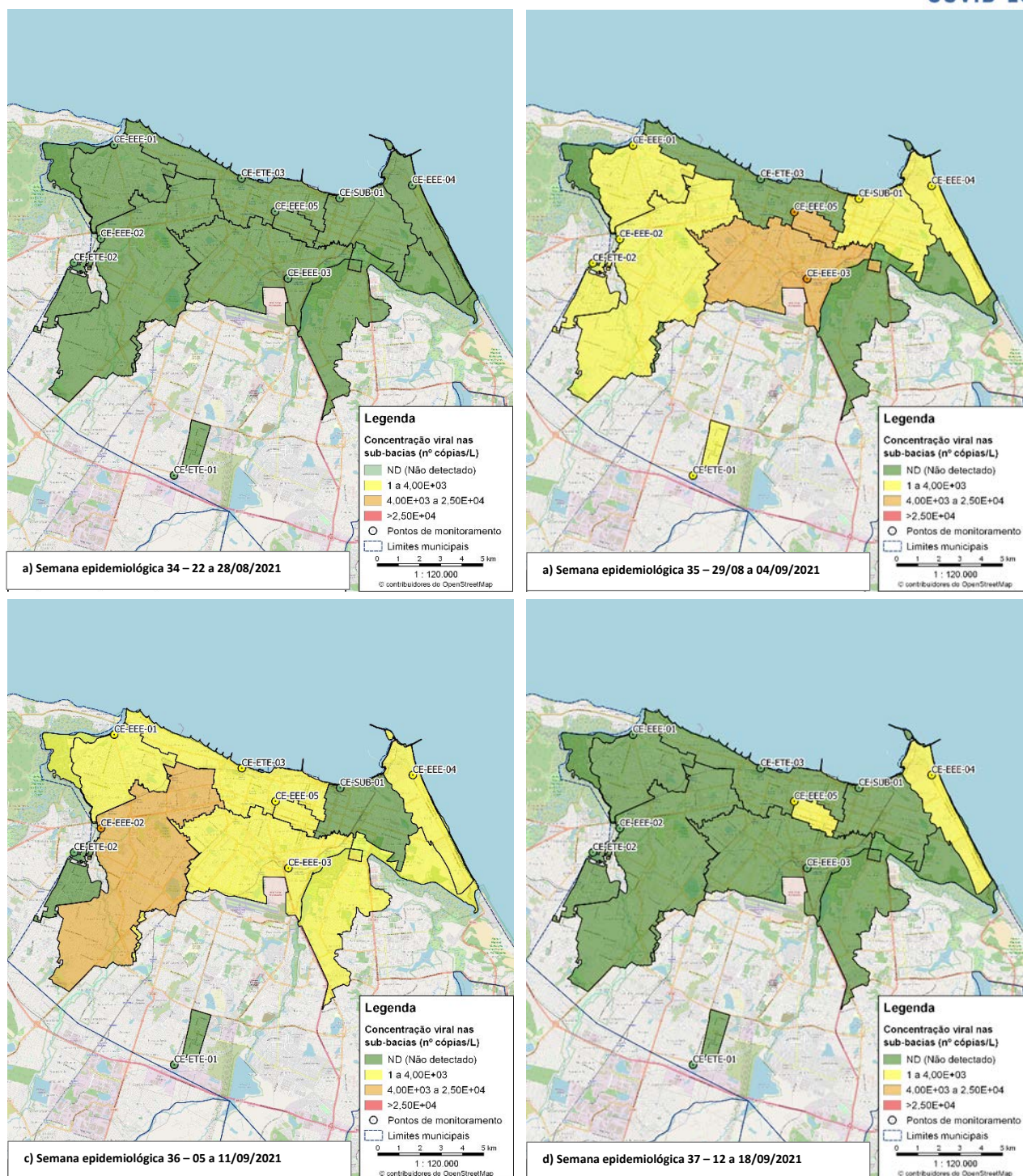
Figura 19 – Distribuição espacial das concentrações do SARS-CoV-2 nas ETEs, sub-bacia e estações elevatórias monitoradas em Fortaleza nas semanas epidemiológicas (a) 34, (b) 35, (c) 36 e (d) 37 de 2021
