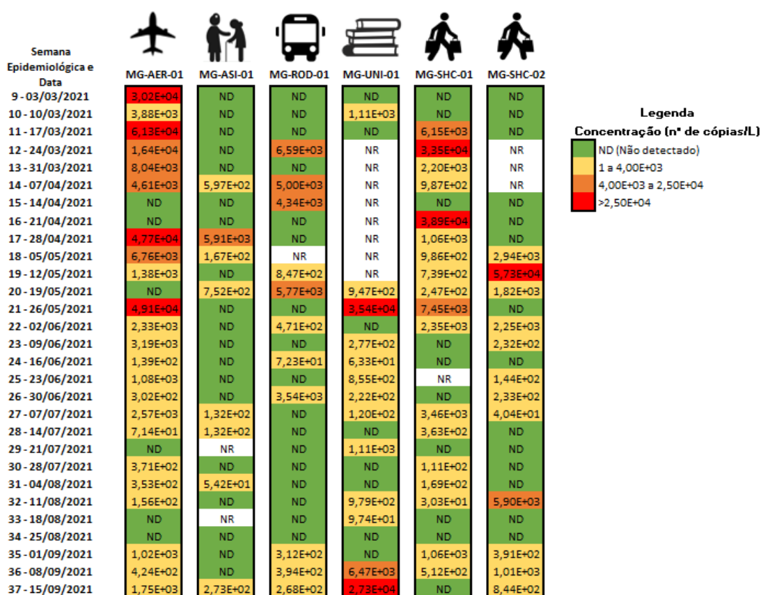
Figura 11 – Concentração de SARS-CoV-2 no esgoto dos pontos especiais monitorados em Belo Horizonte
