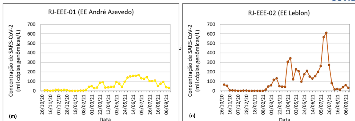
Figura 26 – Série temporal da média móvel de duas semanas das concentrações do SARS-CoV-2 no esgoto das ETEs (a até l) e estações elevatórias (m e n) monitoradas no Rio de Janeiro
