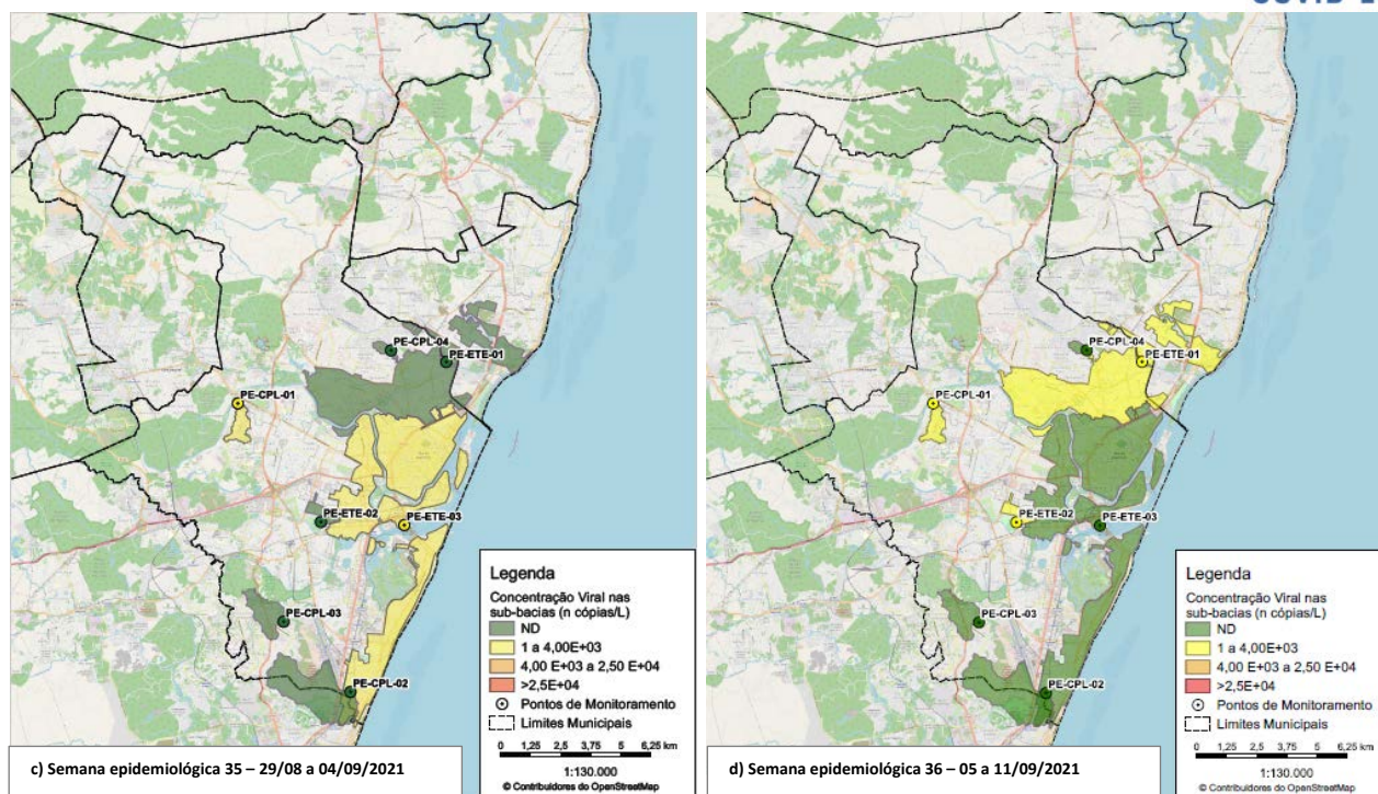
Figura 22 – Distribuição espacial das concentrações do SARS-CoV-2 nas ETEs monitoradas em Recife nas semanas epidemiológicas (a) 33, (b) 34, (c) 35 e (d) 36 de 2021
