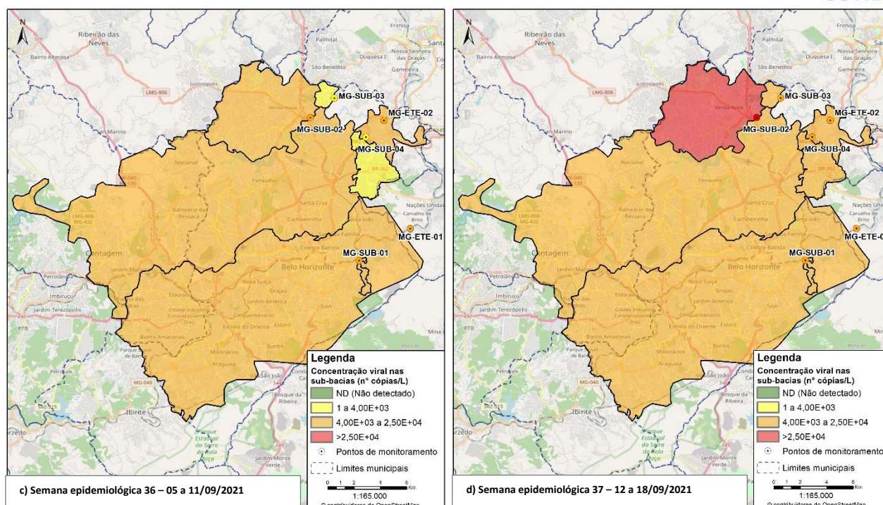
Figura 8 – Distribuição espacial das concentrações do SARS-CoV-2 nas ETEs e sub-bacias monitoradas em Belo Horizonte nas semanas epidemiológicas (a) 34, (b) 35, (c) 36 e (d) 37 de 2021
