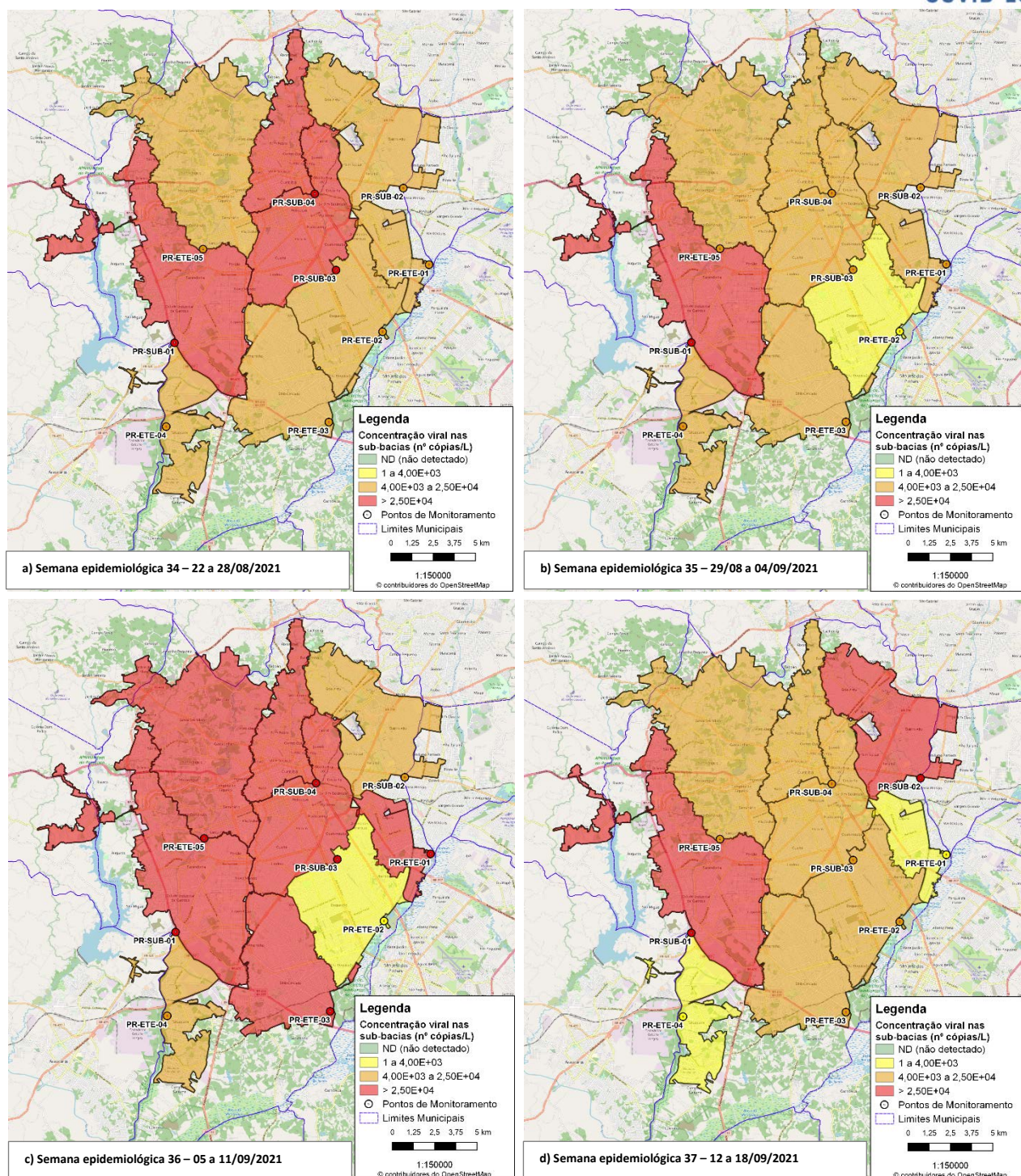
Figura 12 – Distribuição espacial das concentrações do SARS-CoV-2 nas ETEs e sub-bacias monitoradas em Curitiba nas semanas epidemiológicas (a) 34, (b) 35, (c) 36 e (d) 37 de 2021
