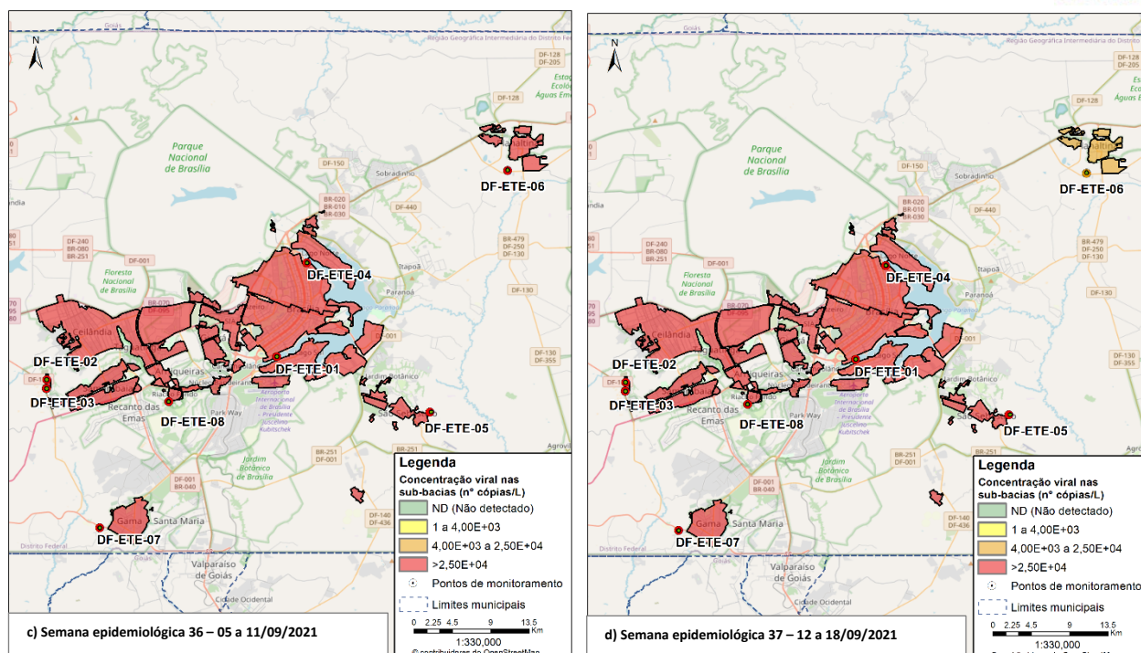
Figura 16 – Distribuição espacial das concentrações do SARS-CoV-2 nas ETEs monitoradas no Distrito Federal nas semanas epidemiológicas (a) 34, (b) 35, (c) 36 e (d) 37 de 2021
