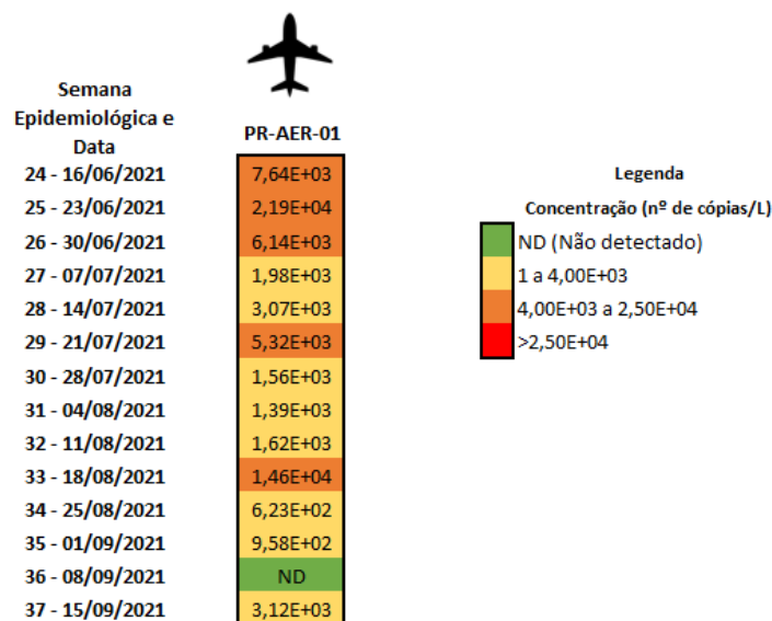
Figura 15 - Concentração de SARS-CoV-2 no esgoto do ponto especial monitorado em Curitiba
