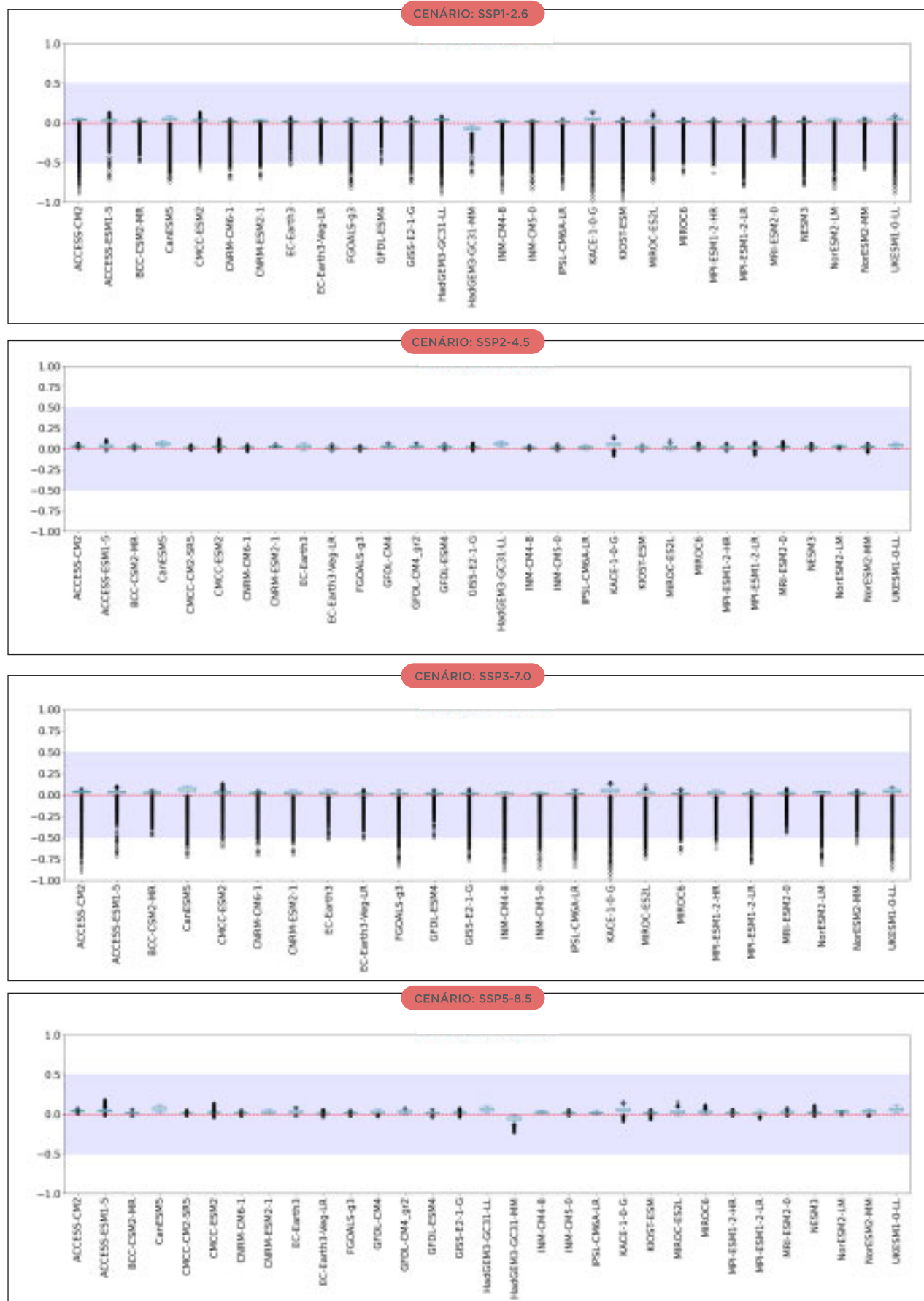
Figura 21 - Box Plot com todos os valores de E_0 em todo o Brasil no período 2015-2040 considerando todos os MCGs e cenários de emissão.
