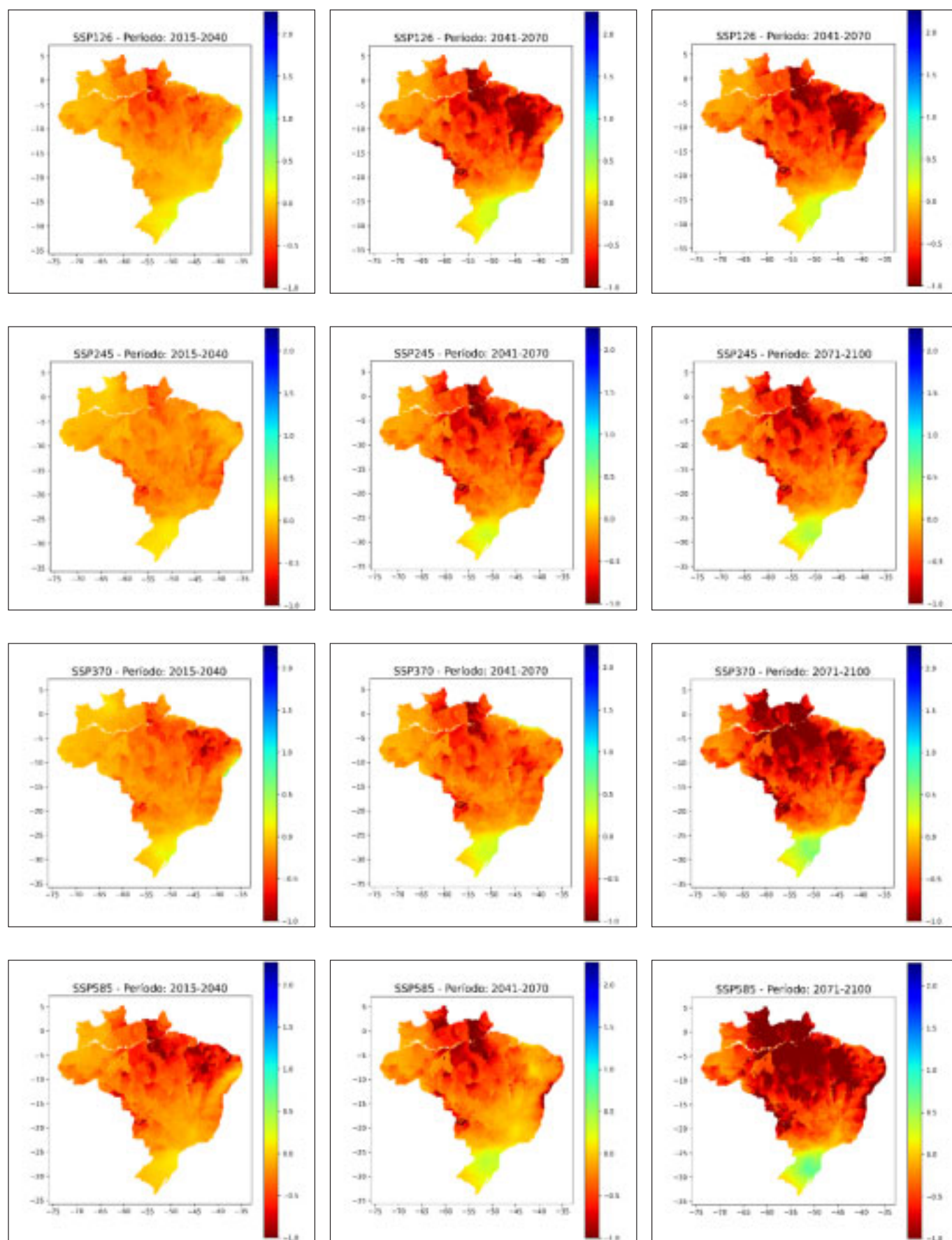
Figura 39 - Mapas da diferença relativa da P para todos os períodos e cenários de emissão do MCG ACCESS-ESM1-5.
