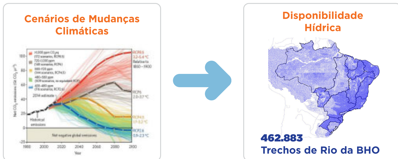
Figura 3 - Ilustração esquemática do objetivo geral do estudo.
