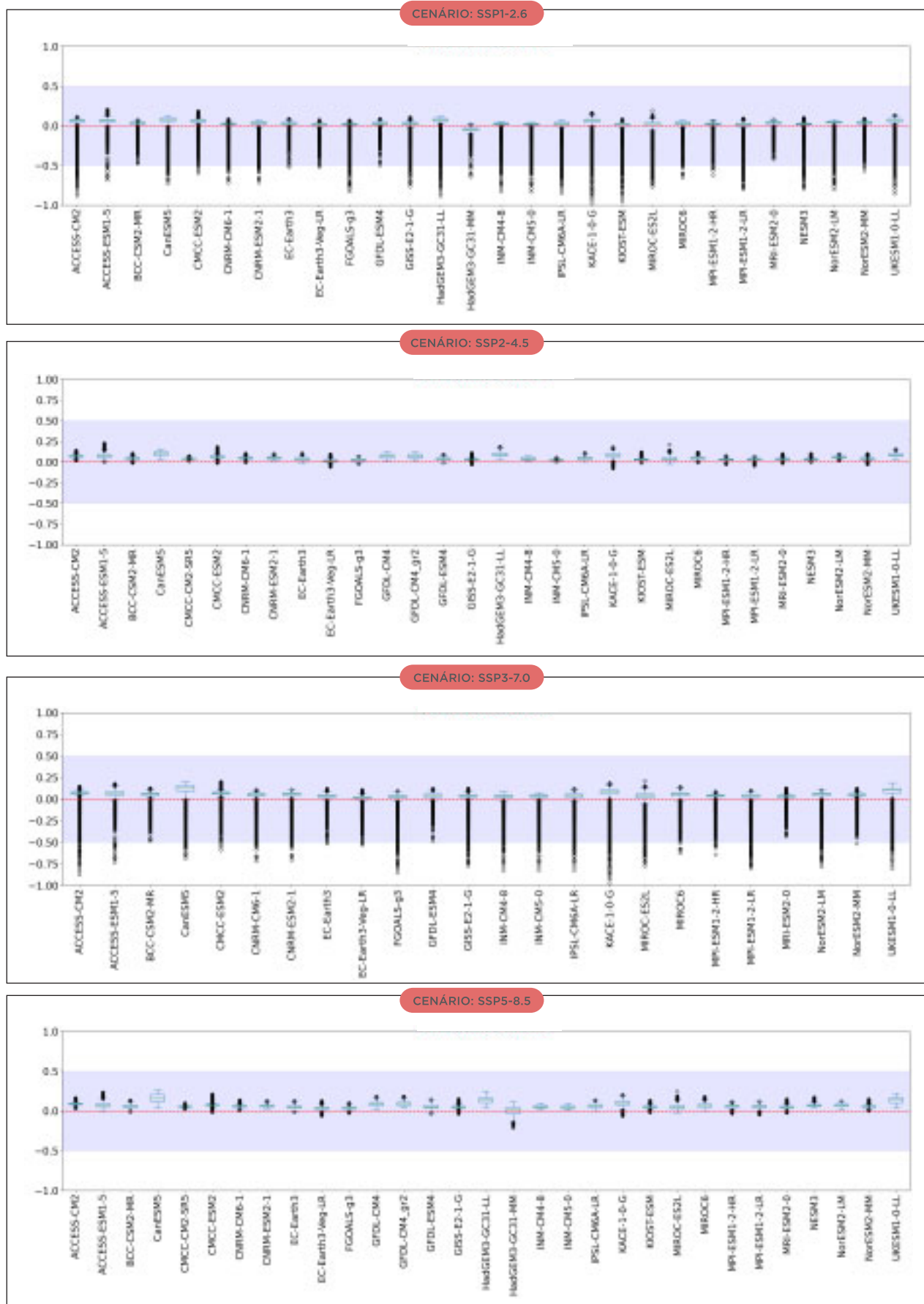
Figura 22 - Box Plot com todos os valores de E_0 em todo o Brasil no período 2041-2070 considerando todos os MCGs e cenários de emissão.
