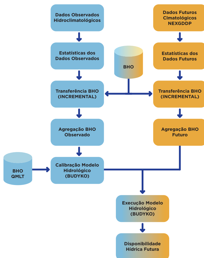
Figura 6 - Esquema metodológico utilizado na avaliação do impacto da mudança climática nos recursos hídricos do Brasil.
