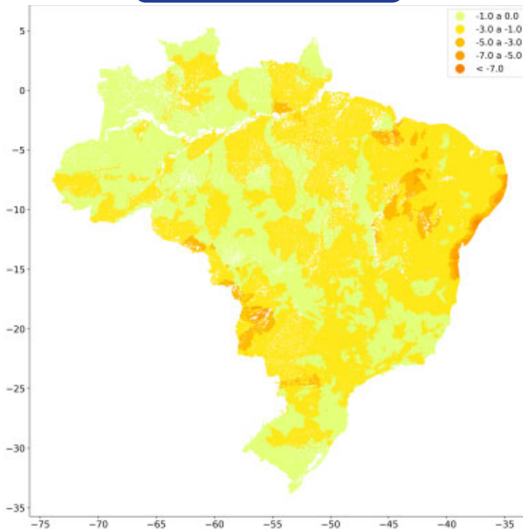
Figura 18 - Valores da elasticidade-evapotranspiração potencial ( \epsilon_2 ) com relação a vazão definidos para cada trecho ou subárea da BHO.
