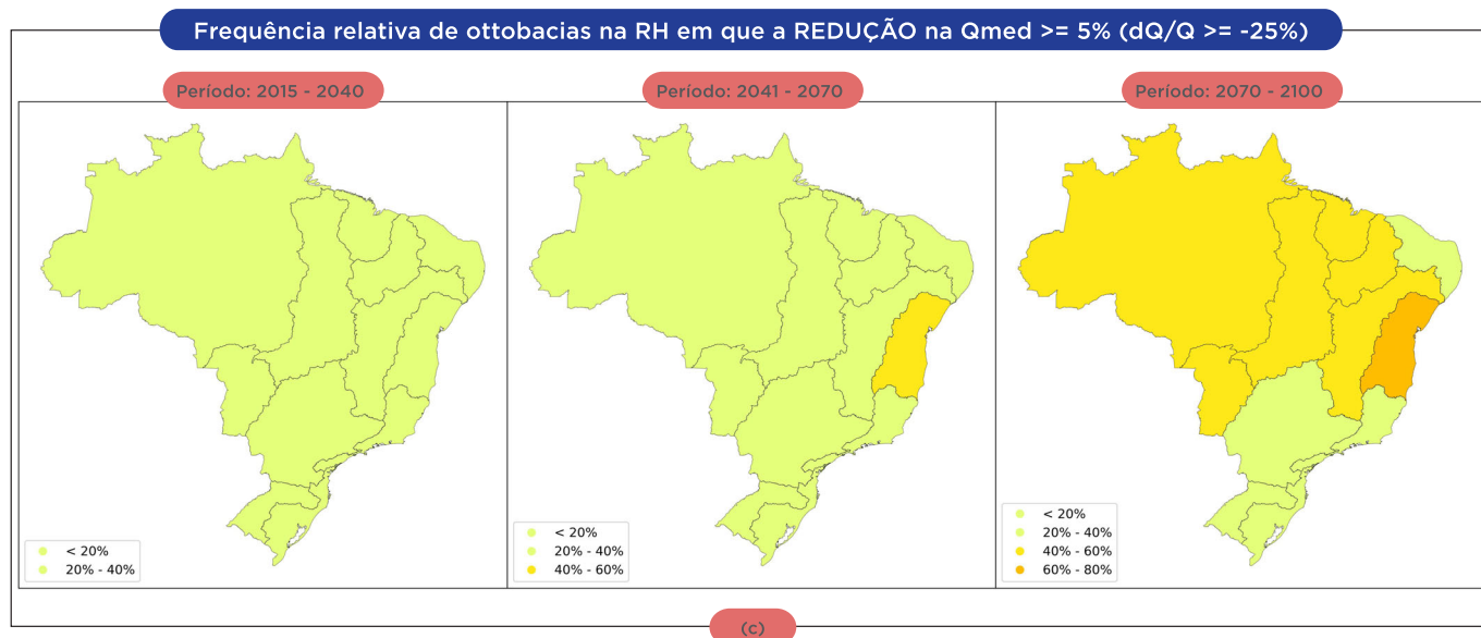
Figura 43 - Mapas do grau de convergência dos cenários climáticos para diminuição na Qmlt em todos os períodos.
