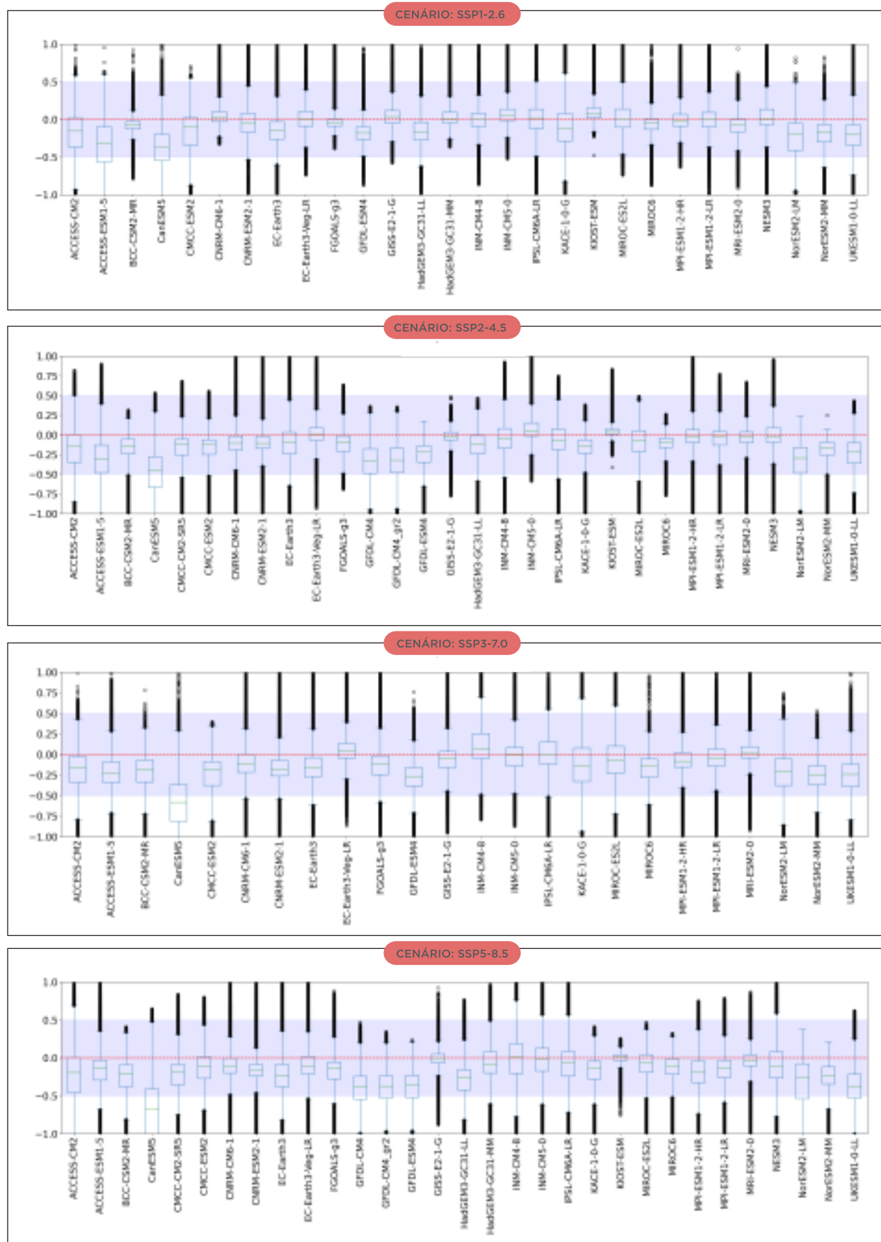
Figura 36 - Box Plot com todos os valores de Qmlt em todo o Brasil no período 2041-2070 considerando todos os MCGs e cenários de emissão.
