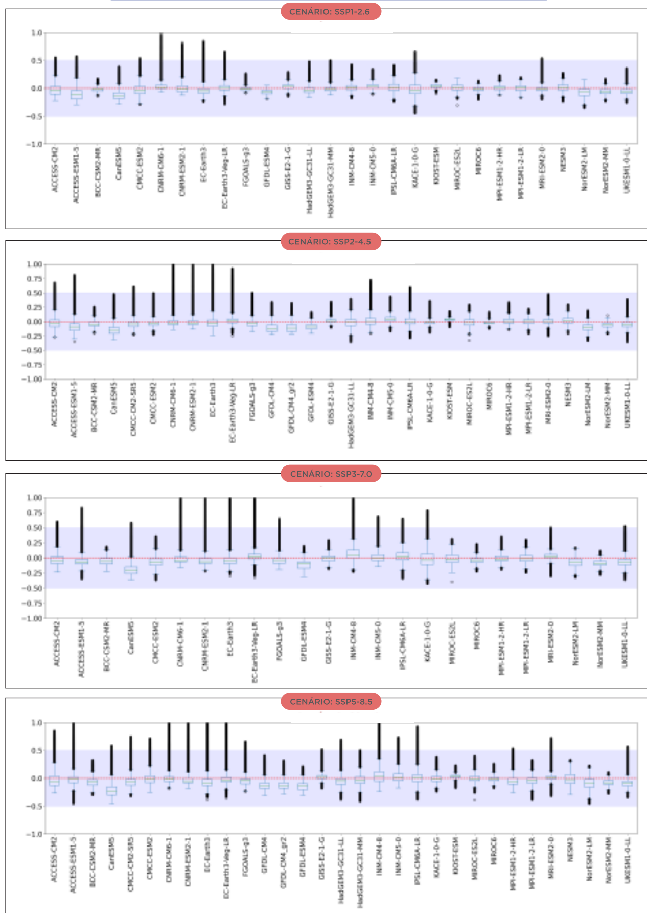
Figura 29 - Box Plot com todos os valores de P em todo o Brasil no período 2041-2070 considerando todos os MCGs e cenários de emissão.
