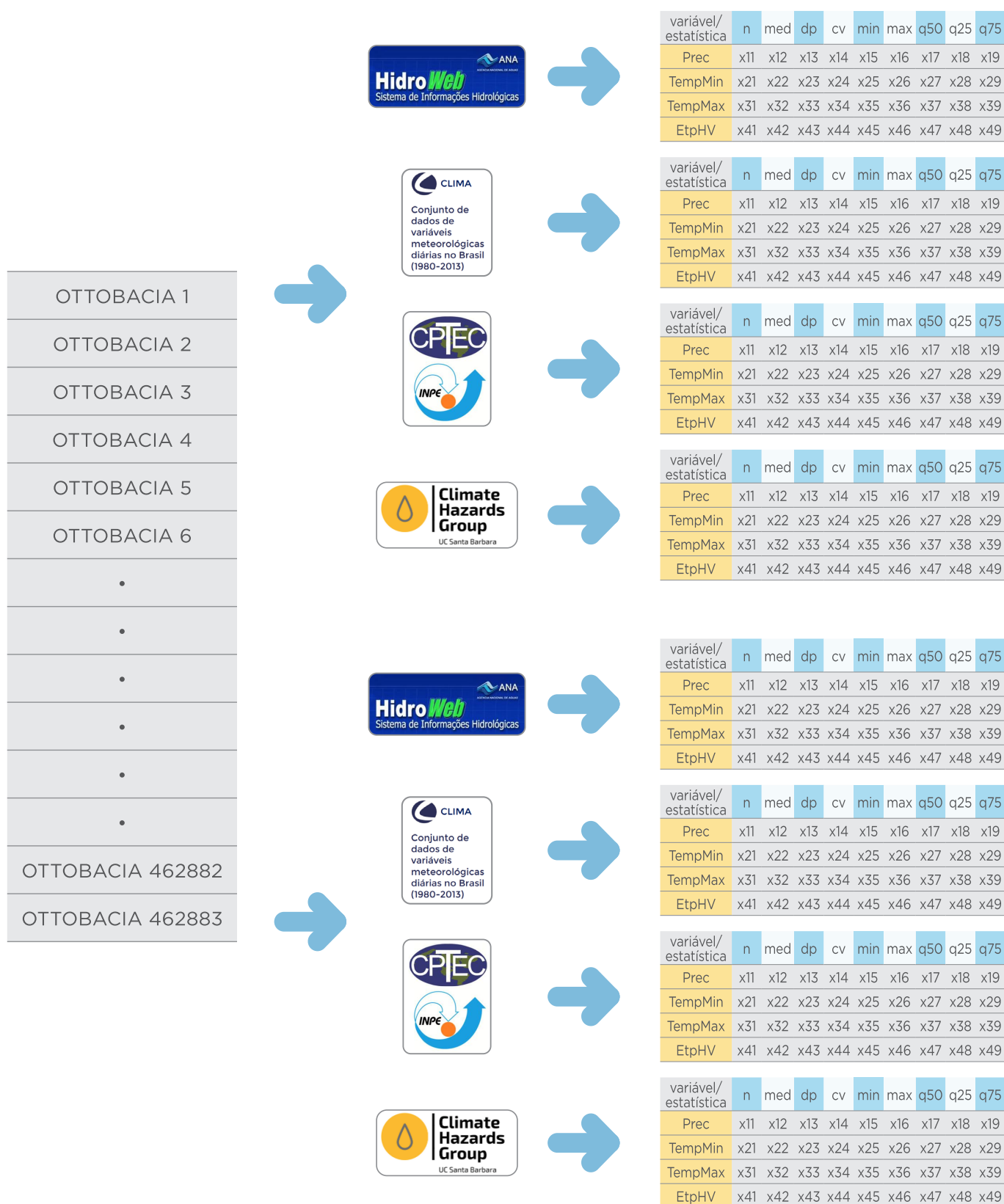
Figura 13 - Esquema da transferência das estatísticas de interesse dos dados climáticos observados para cada um dos 462883 trechos da BHO.
