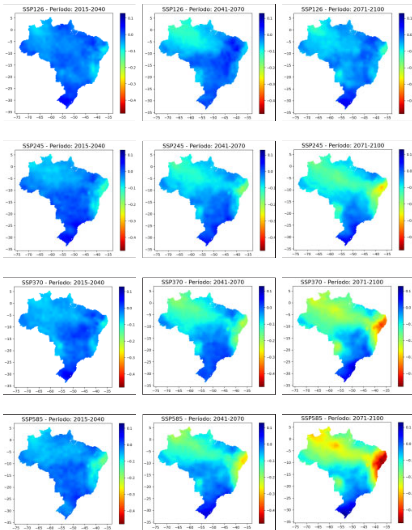
Figura 33 - Mapas da diferença relativa da P para todos os períodos e cenários de emissão do MCG BCC-CSM2-MR.
