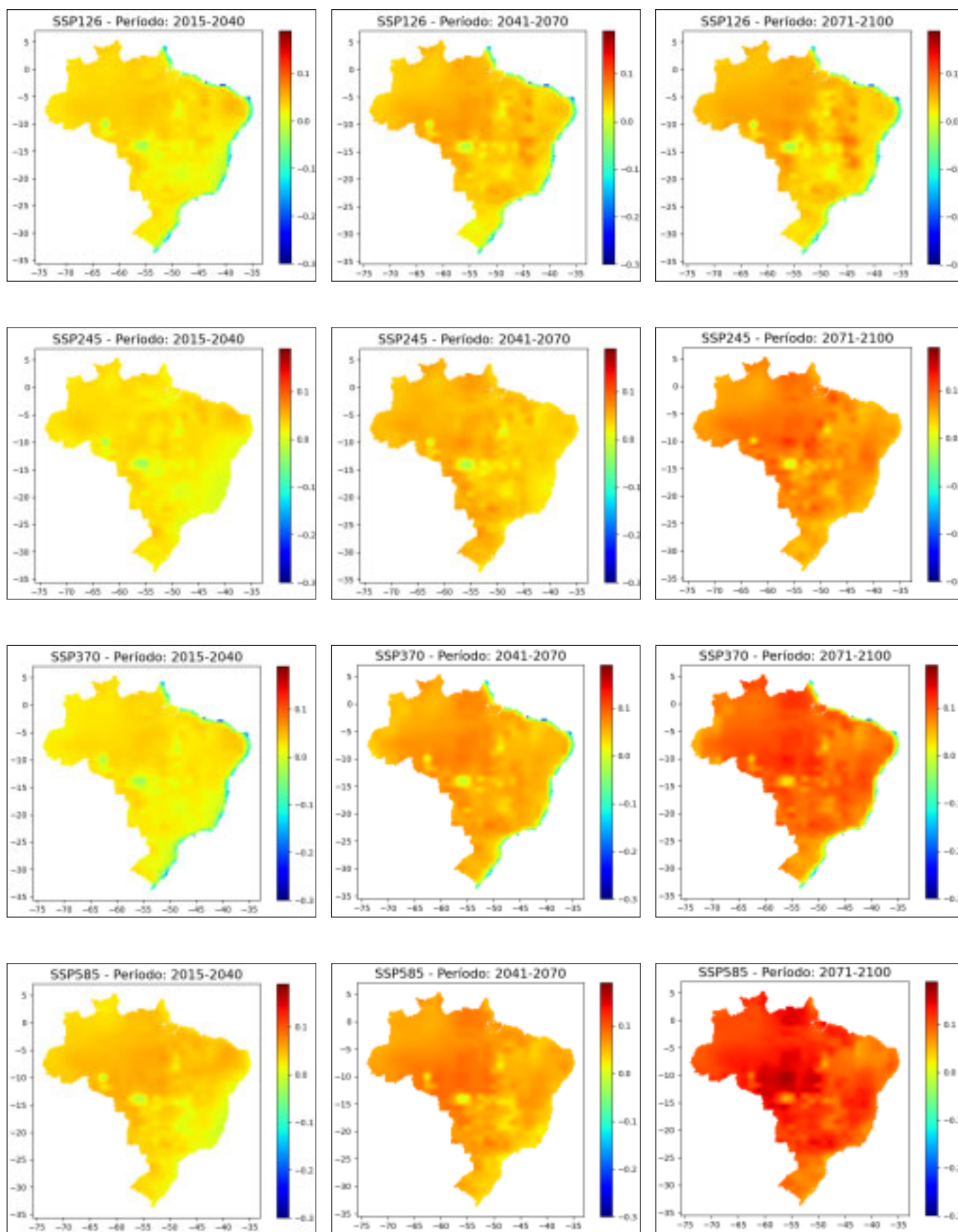
Figura 27 - Mapas da diferença relativa da EO para todos os períodos e cenários de emissão do MCG NORESM2-MM.
