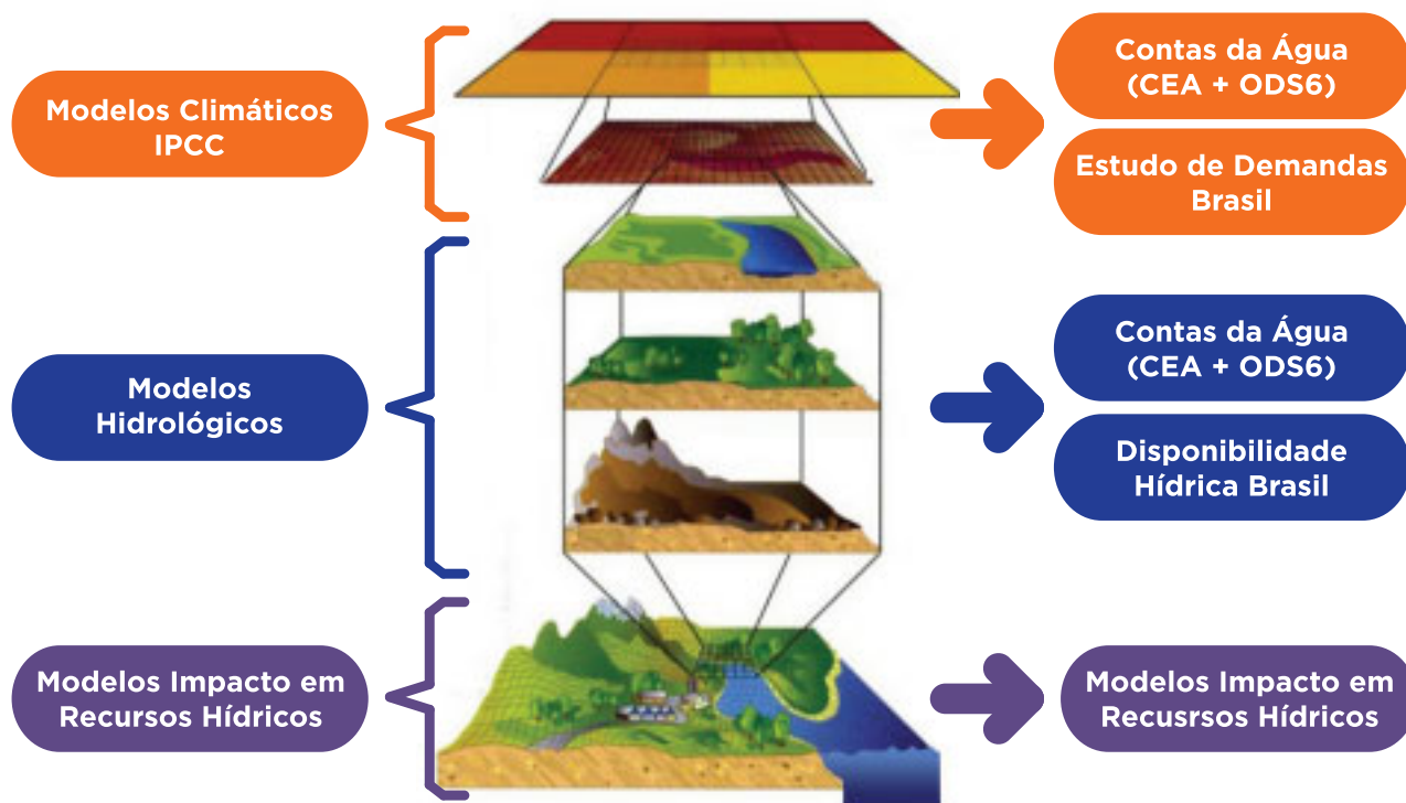
Figura 4 - Abordagem “top-down” na avaliação do impacto da mudança climática nos recursos hídricos. (Adaptado de García et al. 2014)
