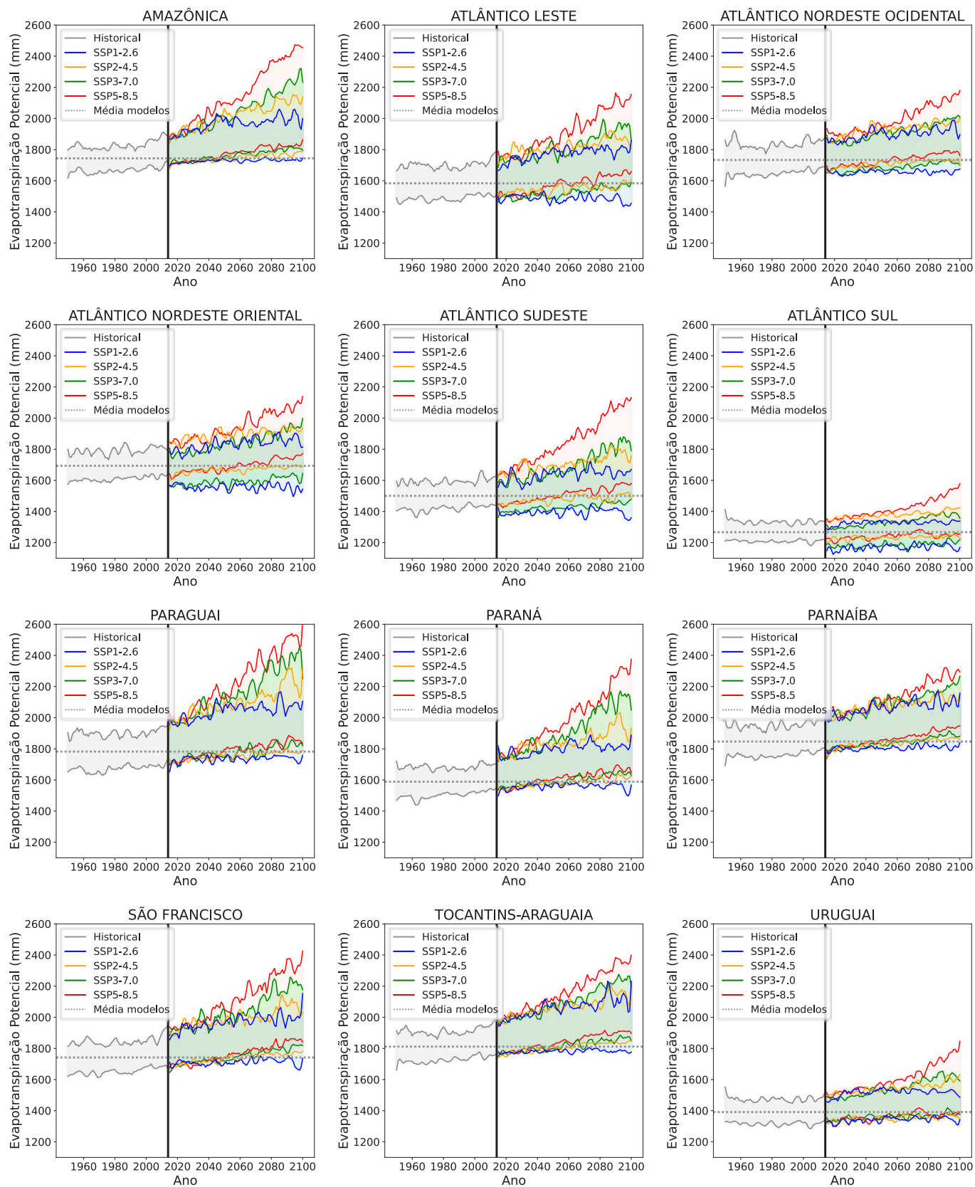
Figura 24 - Evolução das projeções futuras de EO média de todos os MCGs e cenários de emissão para as 12 regiões hidrográficas brasileiras. As curvas coloridas são os limites de cada cenário.
