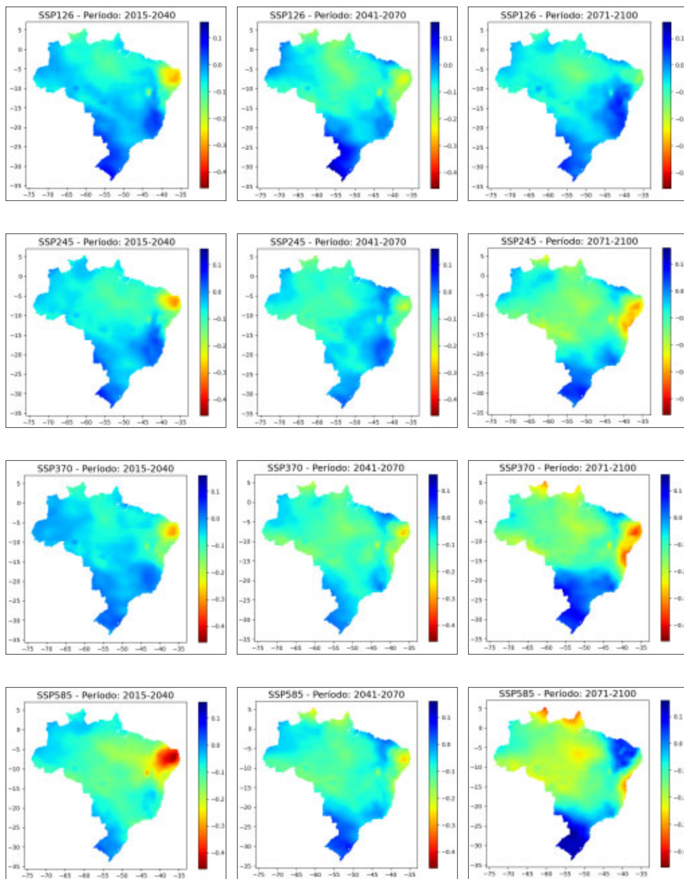
Figura 34 - Mapas da diferença relativa da P para todos os períodos e cenários de emissão do MCG NORESM2-MM.
