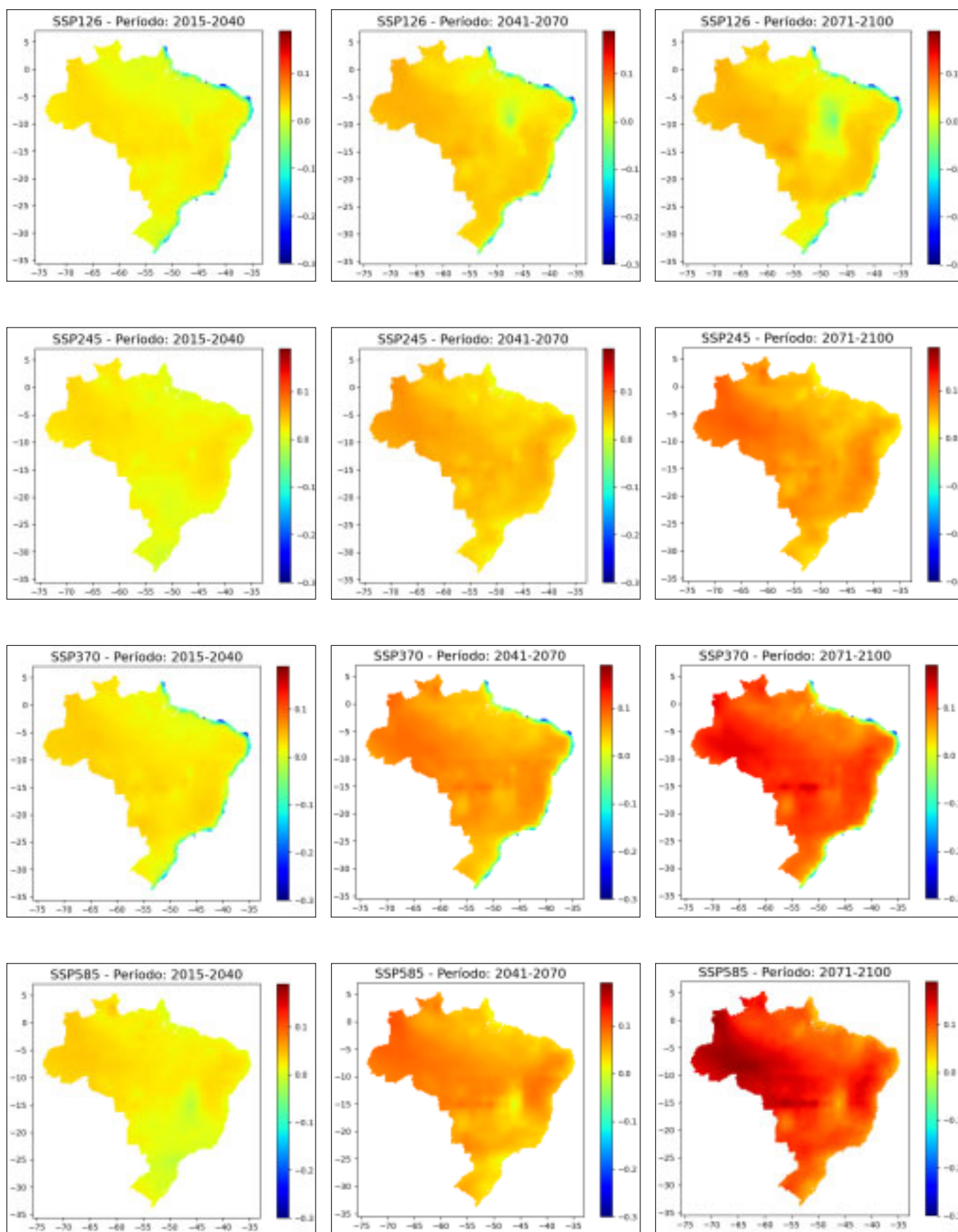
Figura 26 - Mapas da diferença relativa da E0 para todos os períodos e cenários de emissão do MCG BCC-CSM2-MR.
