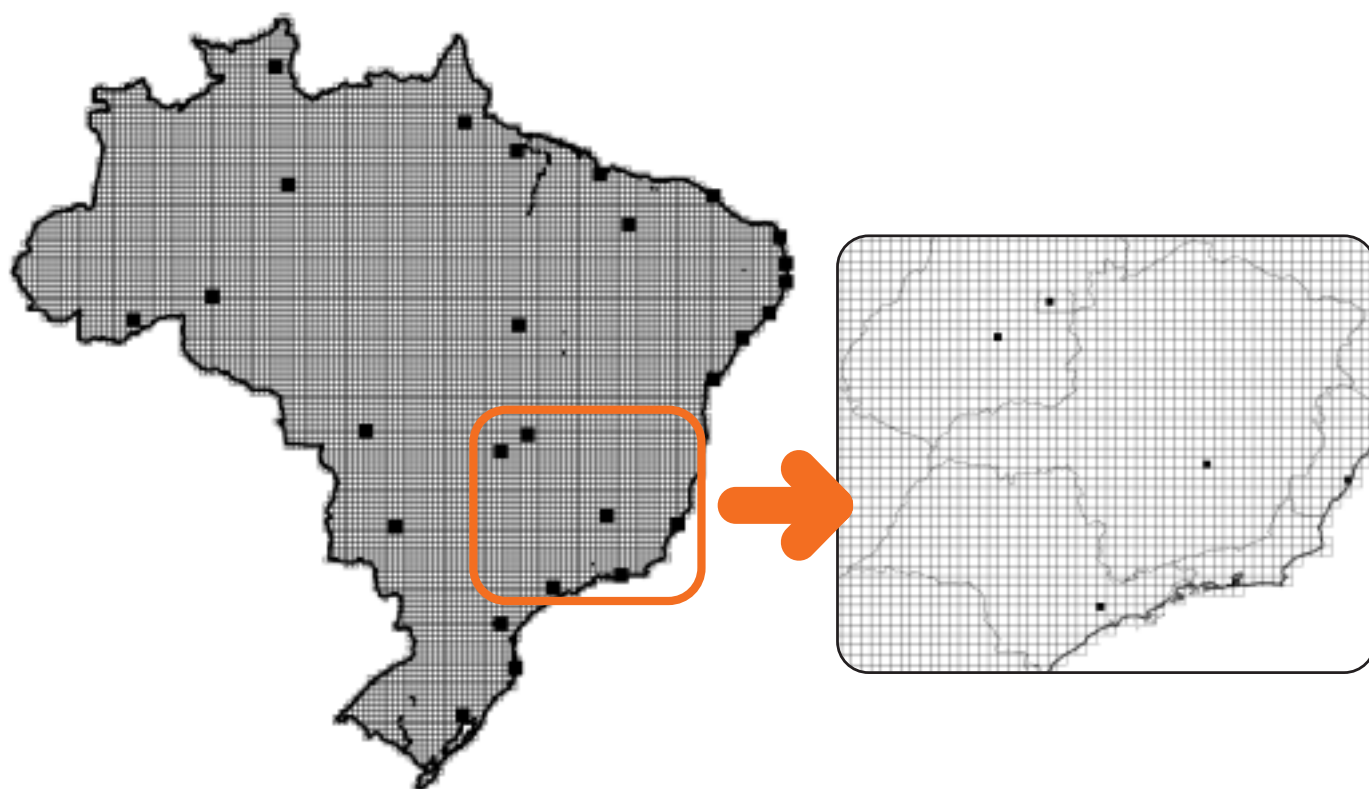
Figura 8 - Grade do projeto NEX-GDDP-CMIP6 recortada para o Brasil. A direita um zoom da grade na região sudeste do Brasil.
