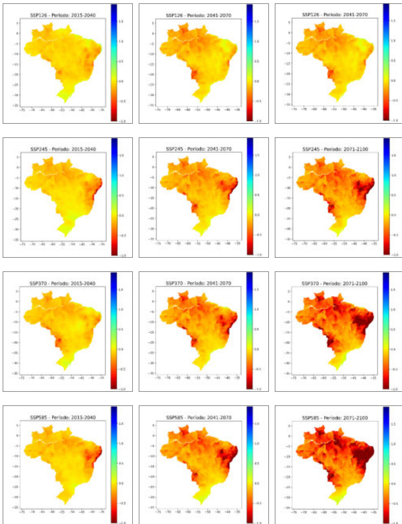
Figura 40 - Mapas da diferença relativa da Q_{m1t} para todos os períodos e cenários de emissão do MCG BCC-CSM2-MR.
