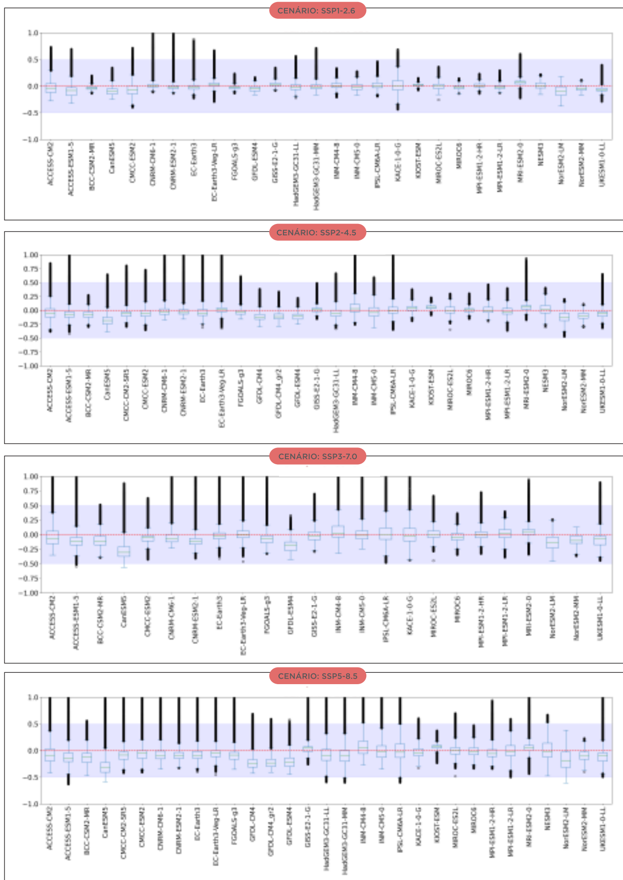
Figura 30 - Box Plot com todos os valores de P em todo o Brasil no período 2071-2100 considerando todos os MCGs e cenários de emissão.
