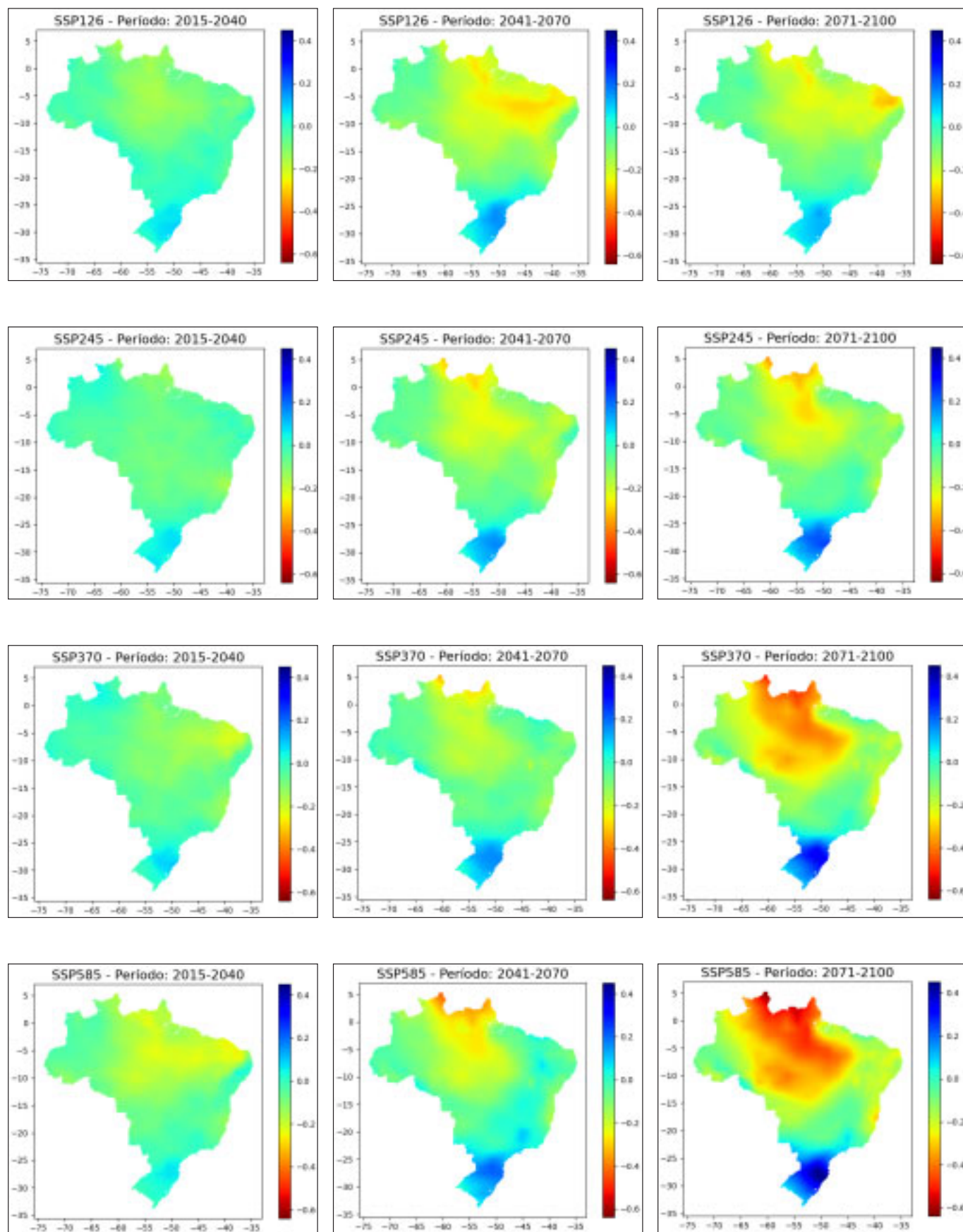
Figura 32 - Mapas da diferença relativa da P para todos os períodos e cenários de emissão do MCG ACCESS-ESM1-5.
