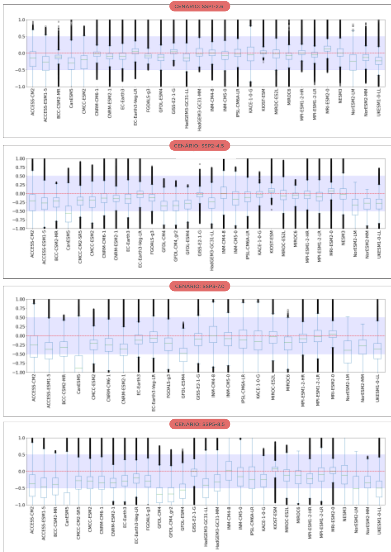
Figura 37 - Box Plot com todos os valores de Q_{mit} em todo o Brasil no período 2071-2100 considerando todos os MCGs e cenários de emissão.
