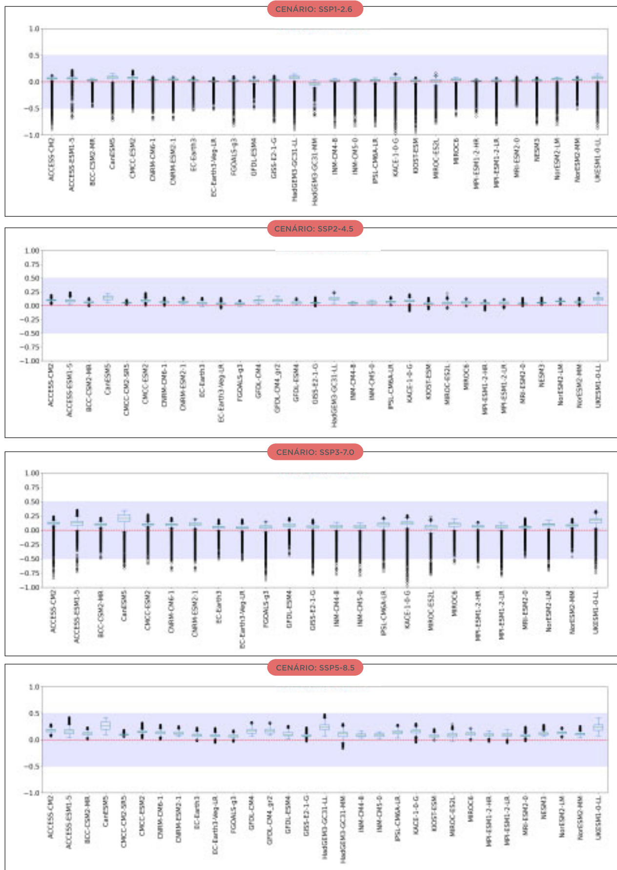
Figura 23 - Box Plot com todos os valores de E_0 em todo o Brasil no período 2071-2100 considerando todos os MCGs e cenários de emissão.
