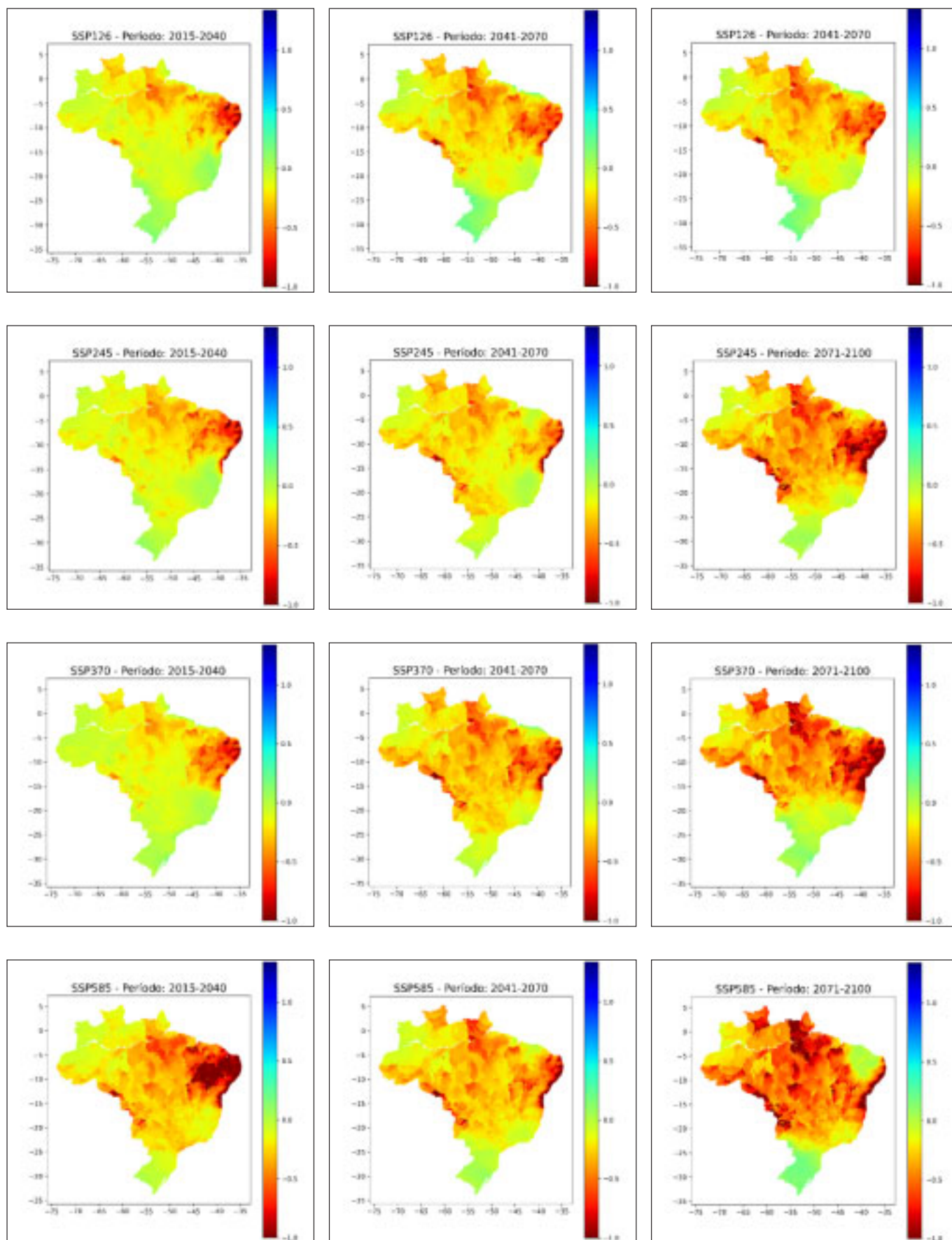
Figura 41 - Mapas da diferença relativa da P para todos os períodos e cenários de emissão do MCG NORESM2-MM
