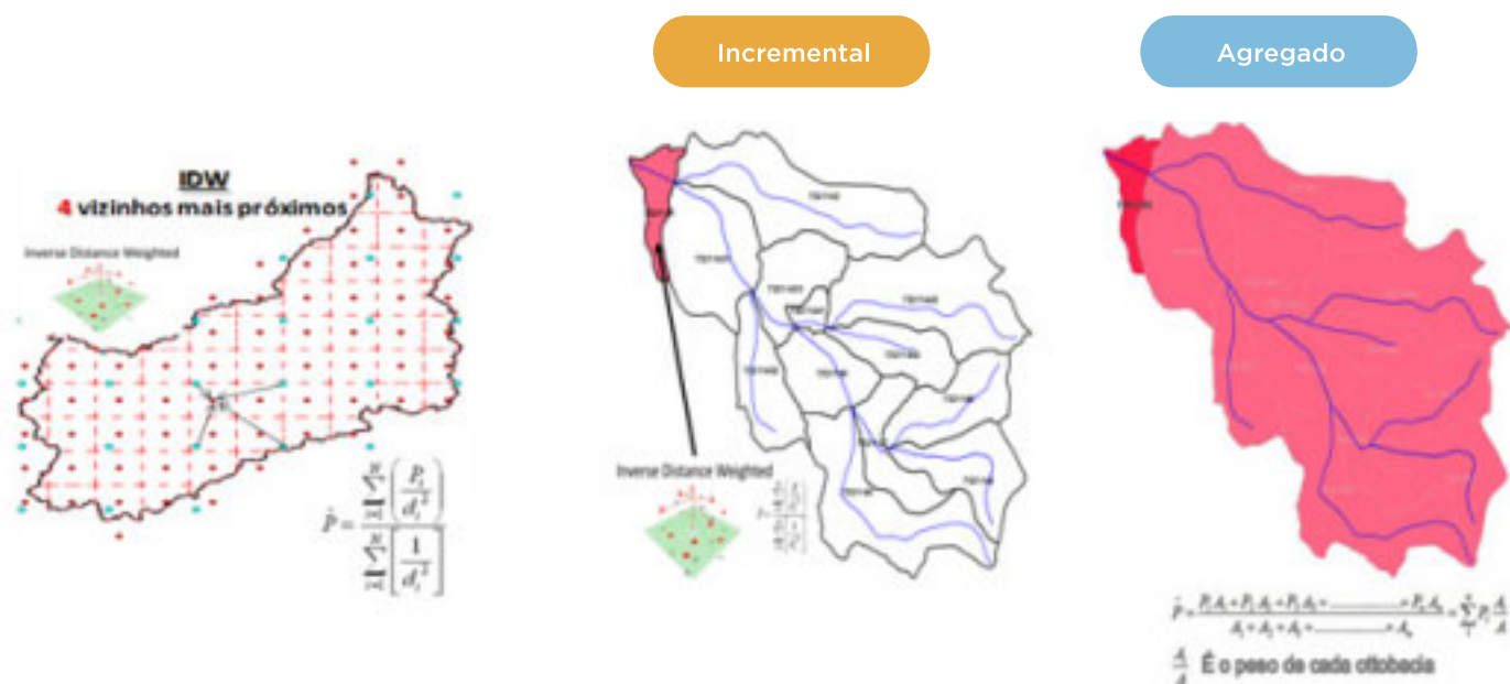
Figura 12 - Procedimento de transferências das estatísticas de interesse dos dados climáticos para a BHO na área incremental e agregada ou total.
