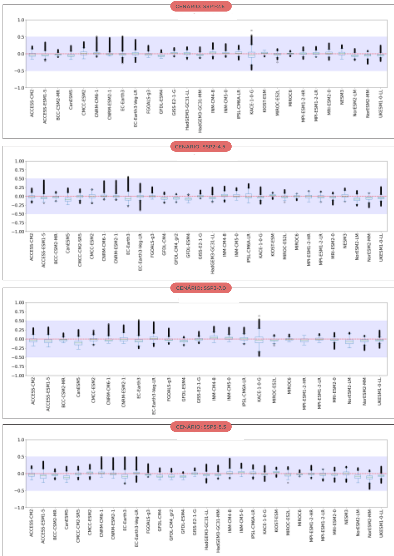
Figura 28 - Box Plot com todos os valores de P em todo o Brasil no período 2015-2040 considerando todos os MCGs e cenários de emissão.
