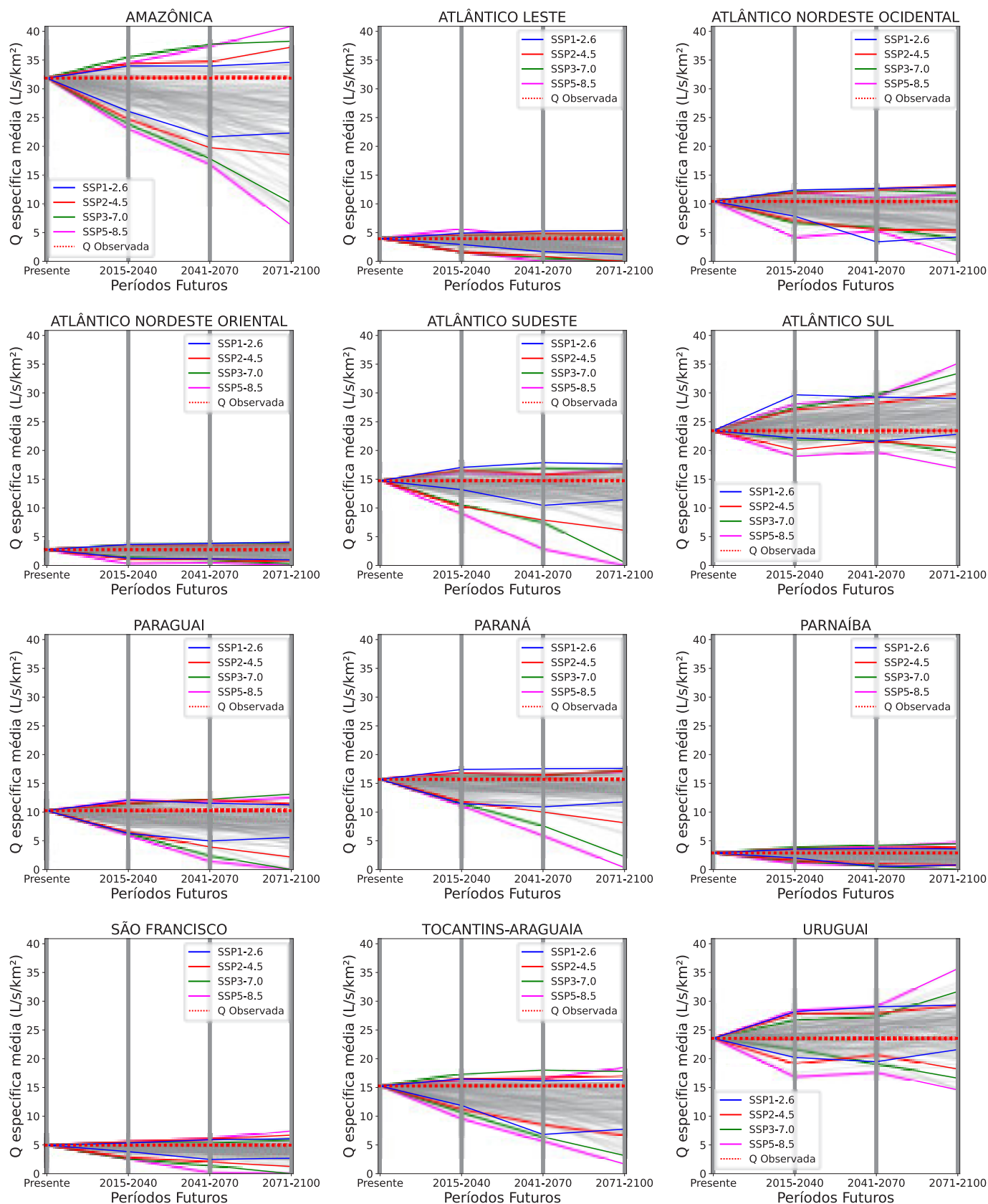
Figura 38 - Evolução das projeções futuras de Q_{mIt} específica incremental média de todos os MCGs e cenários de emissão para as 12 regiões hidrográficas brasileiras. As curvas coloridas são os limites de cada cenário.
