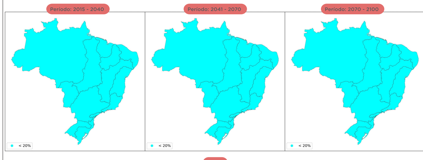
Figura 42 - Mapas do grau de convergência dos cenários climáticos para aumento na QmIt em todos os períodos.
