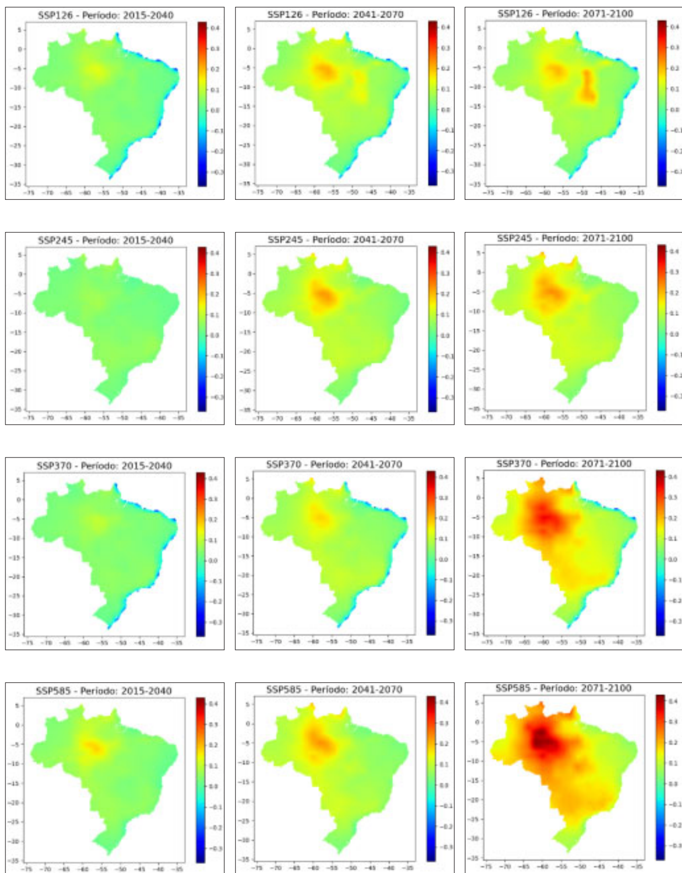
Figura 25 - Mapas da diferença relativa da E0 para todos os períodos e cenários de emissão do MCG ACCESS-ESM1-5.
