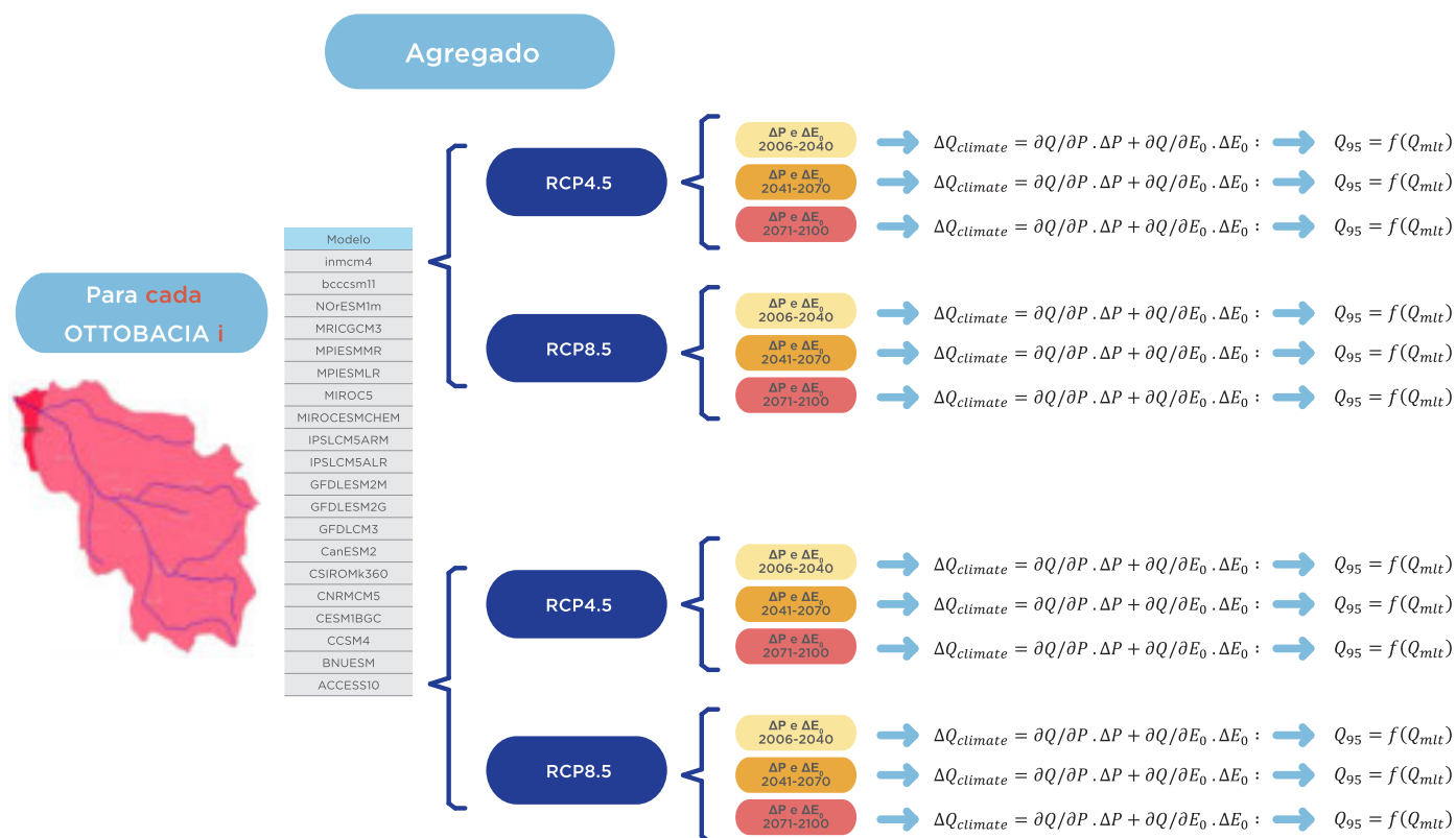
Figura 20 - Esquema de obtenção da mudança na Q_{mit} para cada ottobacia e cada cenário climático (MCG + cenários de emissão).
