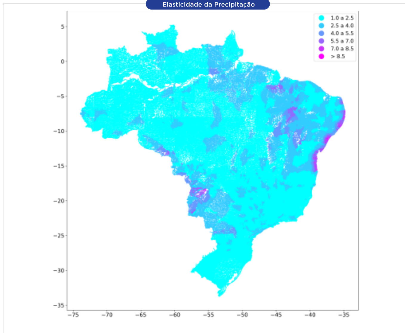
Figura 19 - Valores da elasticidade-precipitação ( \epsilon_1 ) com relação a vazão definidos para cada trecho ou ottobacia da BHO.tobacia da BHO.
