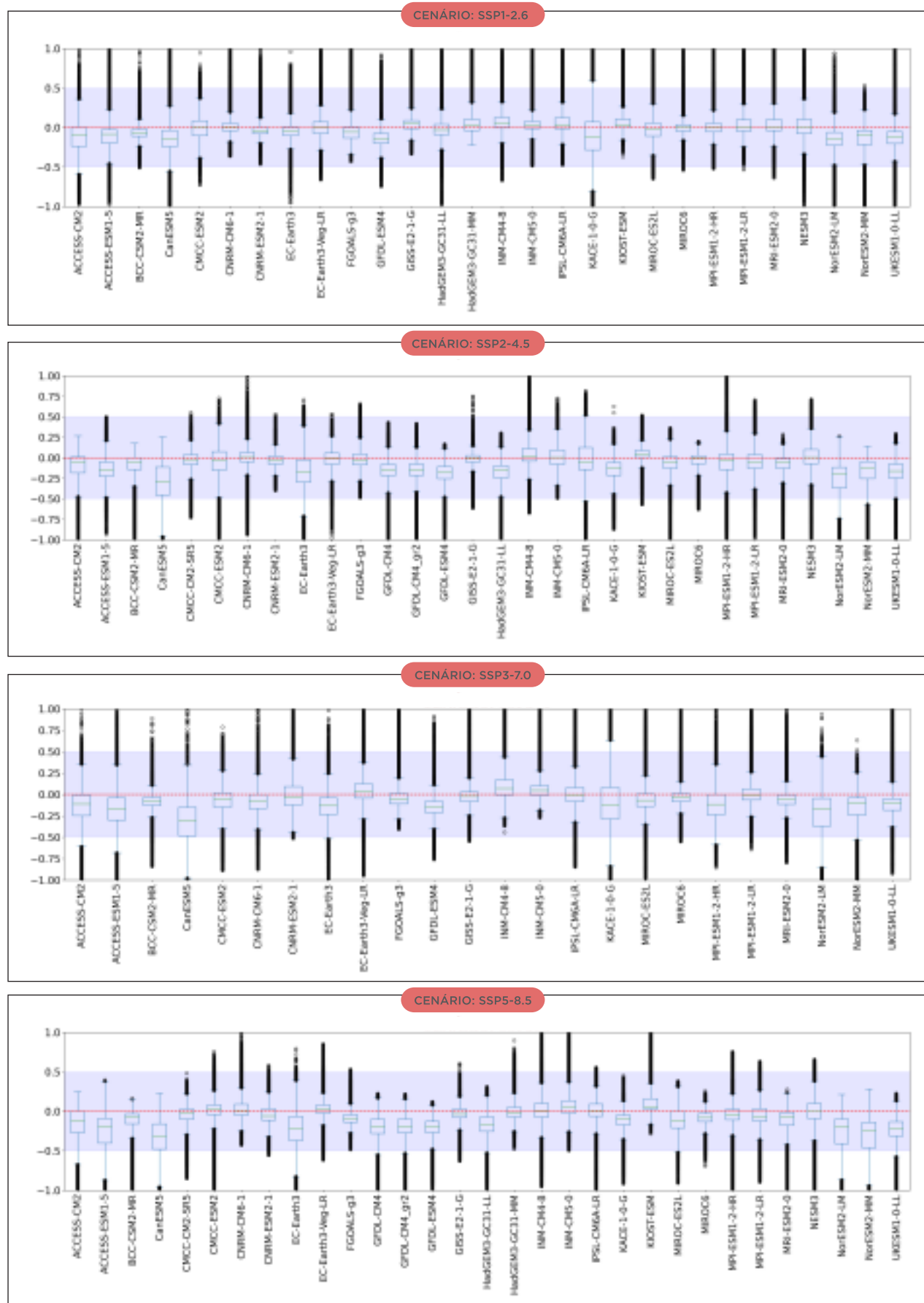
Figura 35 - Box Plot com todos os valores de Q_{m1} em todo o Brasil no período 2015-2040 considerando todos os MCGs e cenários de emissão.
