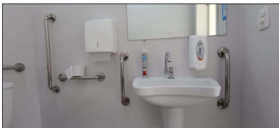
Figura 31 - Fotos do sanitário acessível masculino.
