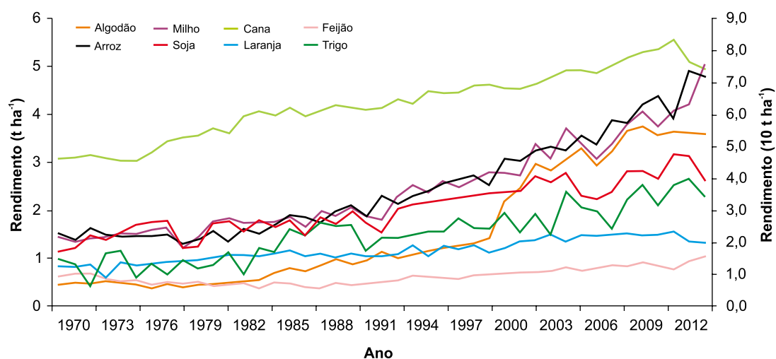
Figura 4. Rendimento biológico da terra (cana-de-açúcar e laranja: 10^4\ kg\ ha^{-1} ; demais, 10^3\ kg\ ha^{-1} ), para as culturas de algodão, arroz, cana-de-açúcar, feijão, laranja, milho, soja e trigo, no período de 1970 a 2012.
