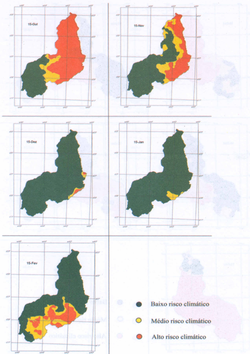
Fig. 5. Espacialização de riscos climáticos para o sorgo precoce em áreas com solo tipo 3.
