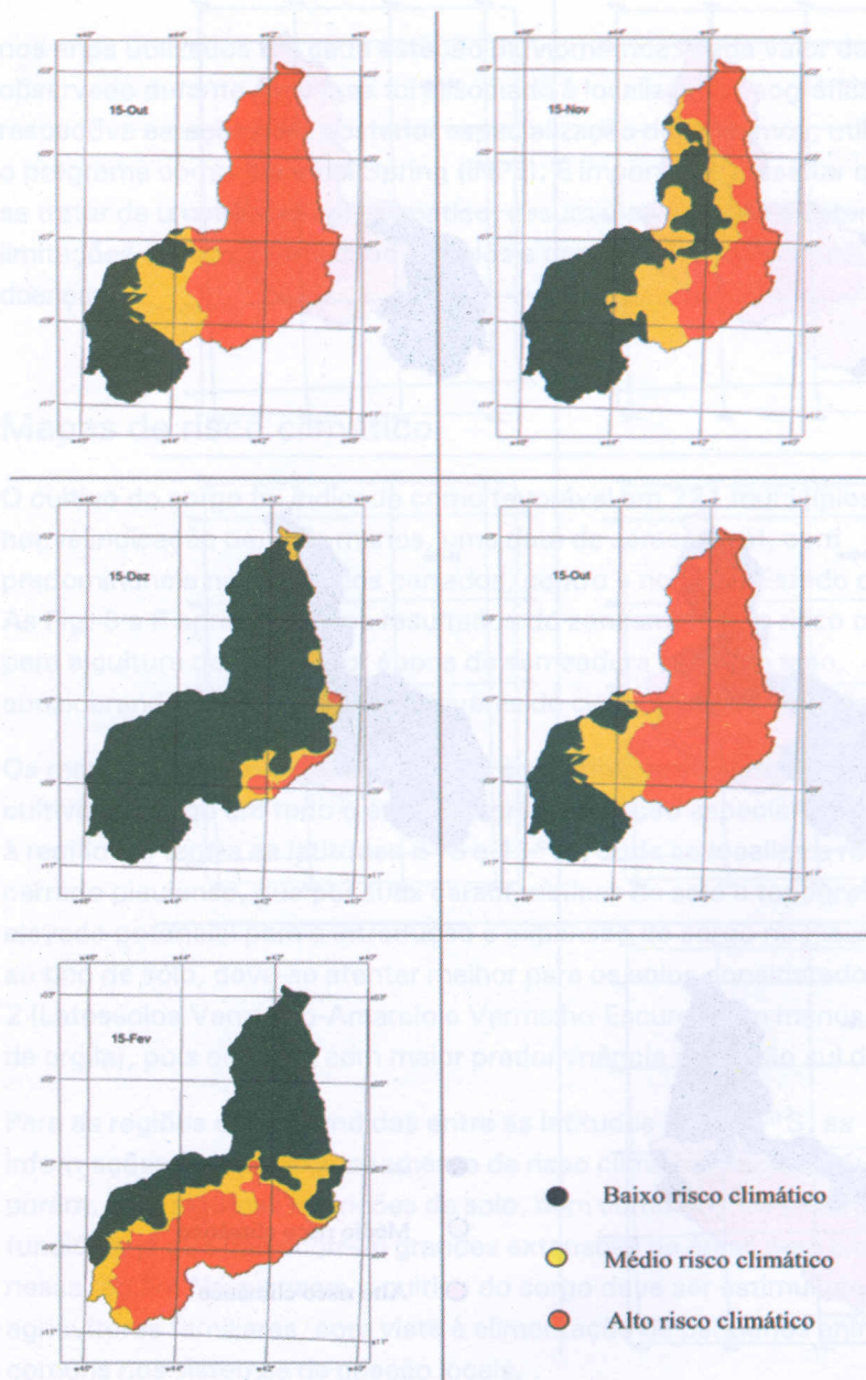
Fig. 4. Espacialização de riscos climáticos para o sorgo precoce em áreas com solo tipo 2.
