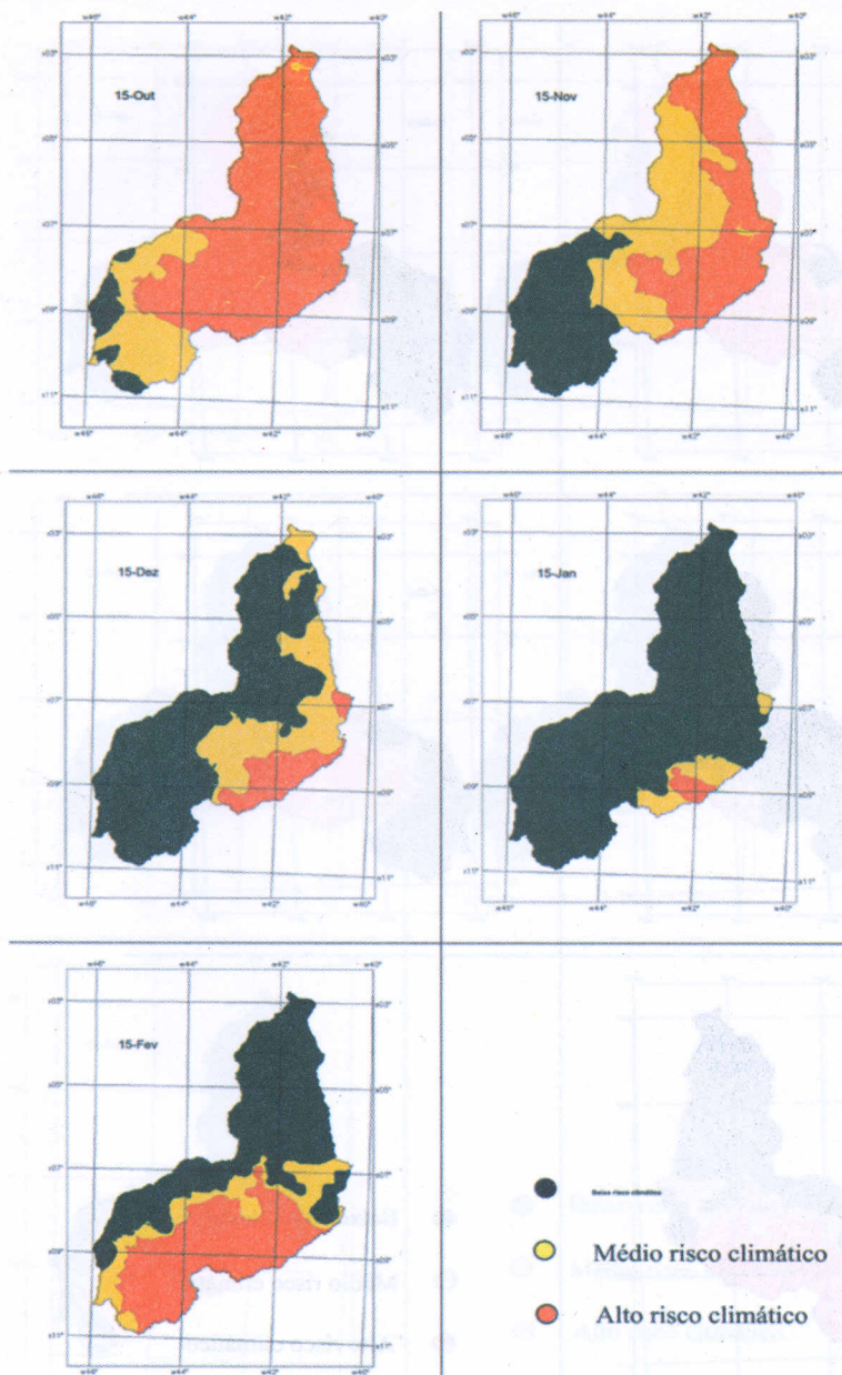
Fig. 3. Espacialização de riscos climáticos para o sorgo precoce em áreas com solo tipo 1.
